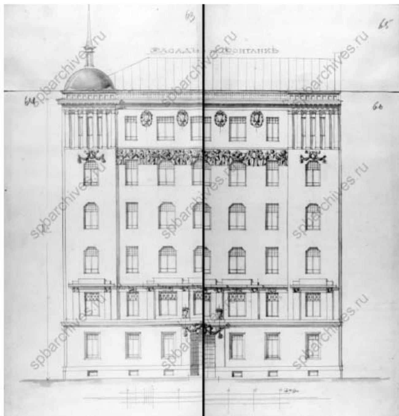
Илл. 18. Лицевой фасад д. 145 по наб. р. Фонтанки, проект Д. Фомичева, 1909 г. ЦГИА СПб ф. 513 оп. 102 д. 3893, л. 88
