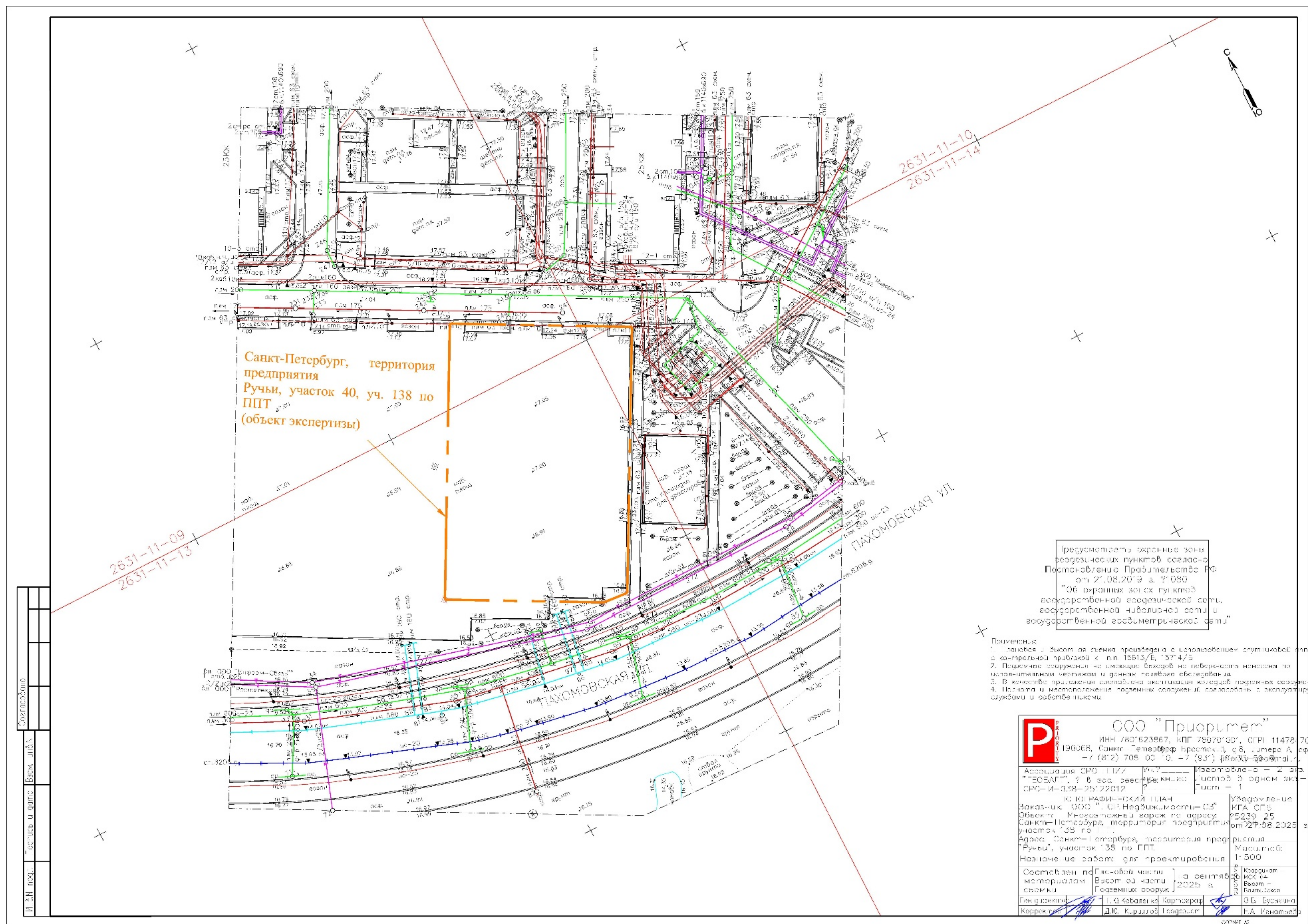
Рис. 26. Участок по адресу Санкт-Петербург, территория предприятия Ручьи, участок с/к 78:11:0005606:39008, уч. 138 по ППТ. Топографический план территории объекта.
