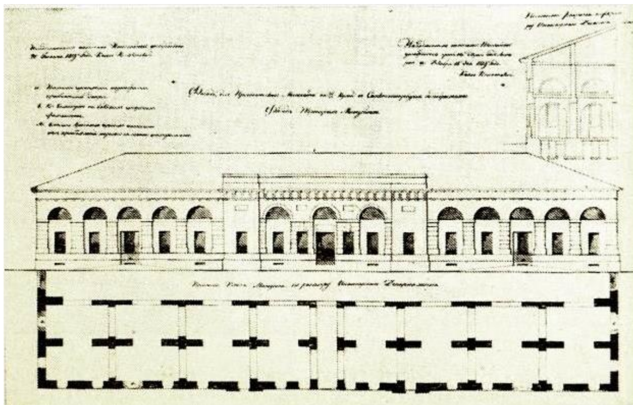
Илл. 1. Измайловские провиантские магазины. Корпус Восточный. Проект В.П. Стасова, 1819 г. Источник: https://www.citywalls.ru/photo600485.html
