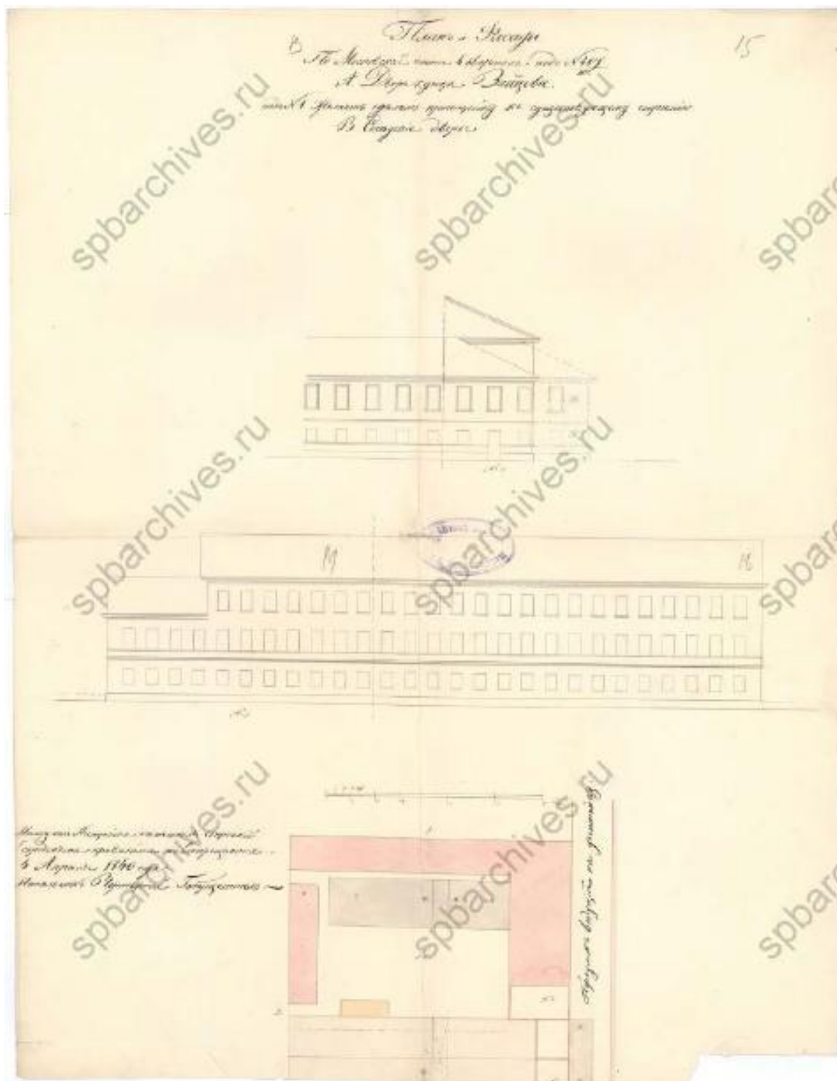
12. План и фасад двора Санкт-Петербургского купца С. Зайцова. Московская часть, 4 квартал, уч. №467. Проект перестройки и надстройки угловой части главного корпуса и примыкающего корпуса. Октябрь 1839 г. // ЦГИА СПб. Фонд 513. Описание 102. Дело 4841. Лл. 13-16.
