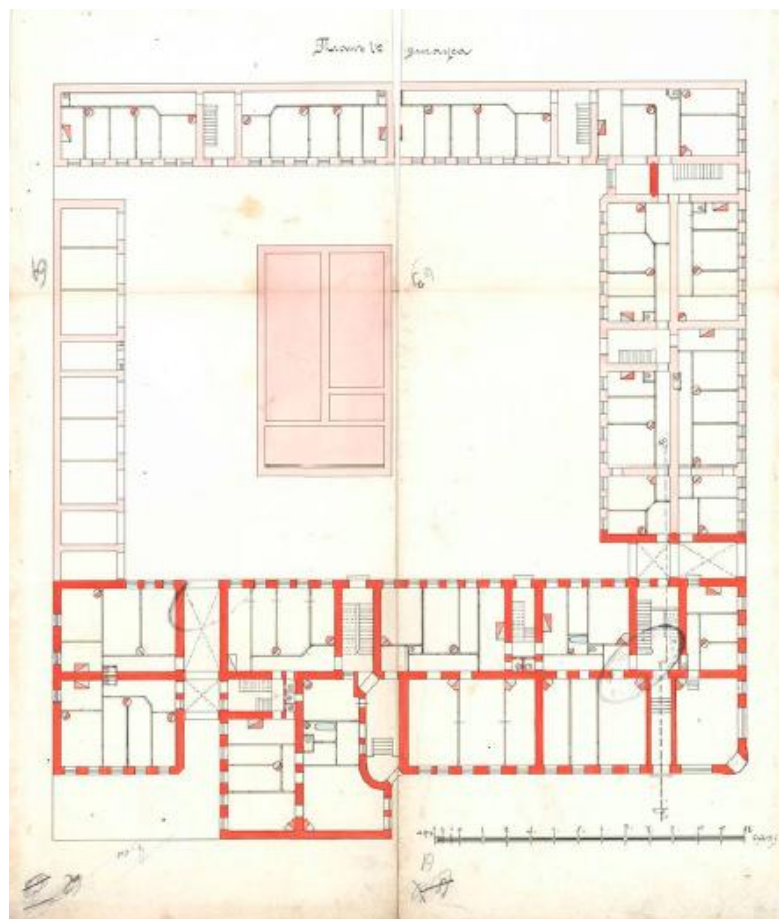
21. Проект дома Ф.И. Кривдина. План 1-го этажа. Архитектор А. Шильцов. 1905 г. // ЦГИА СПб. Фонд 513. Описание 102. Дело 4841. Лл. 61-64.
