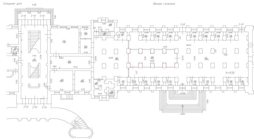
ПЛАН части 1 ЭТАЖА
