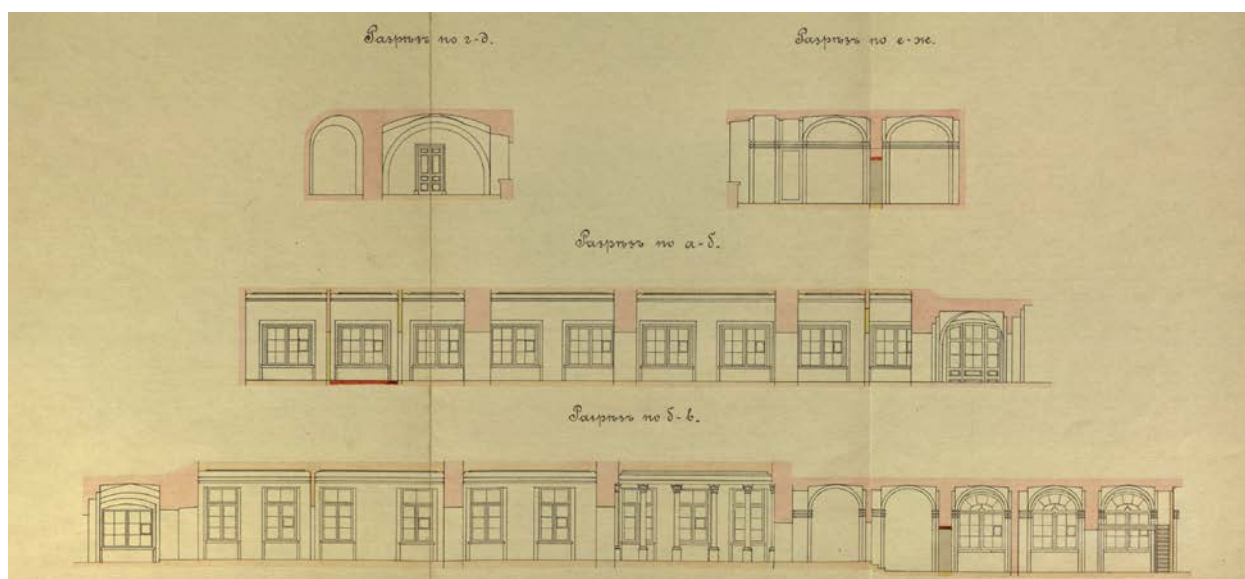
14. Архитектор Бах А.Р. План и четыре разреза первого этажа. 1904 г. ФГБУК "Государственный художественно-архитектурный дворцово-парковый музей-заповедник "Царское Село" ЕД-1531-ХIII.
