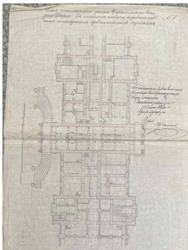
12. План нижнего этажа лестницы с прилегающими помещениями 186 г. ФГБУК "Государственный художественно-архитектурный дворцово-парковый музей-заповедник "Царское Село" ЕД-1486-ХIII
