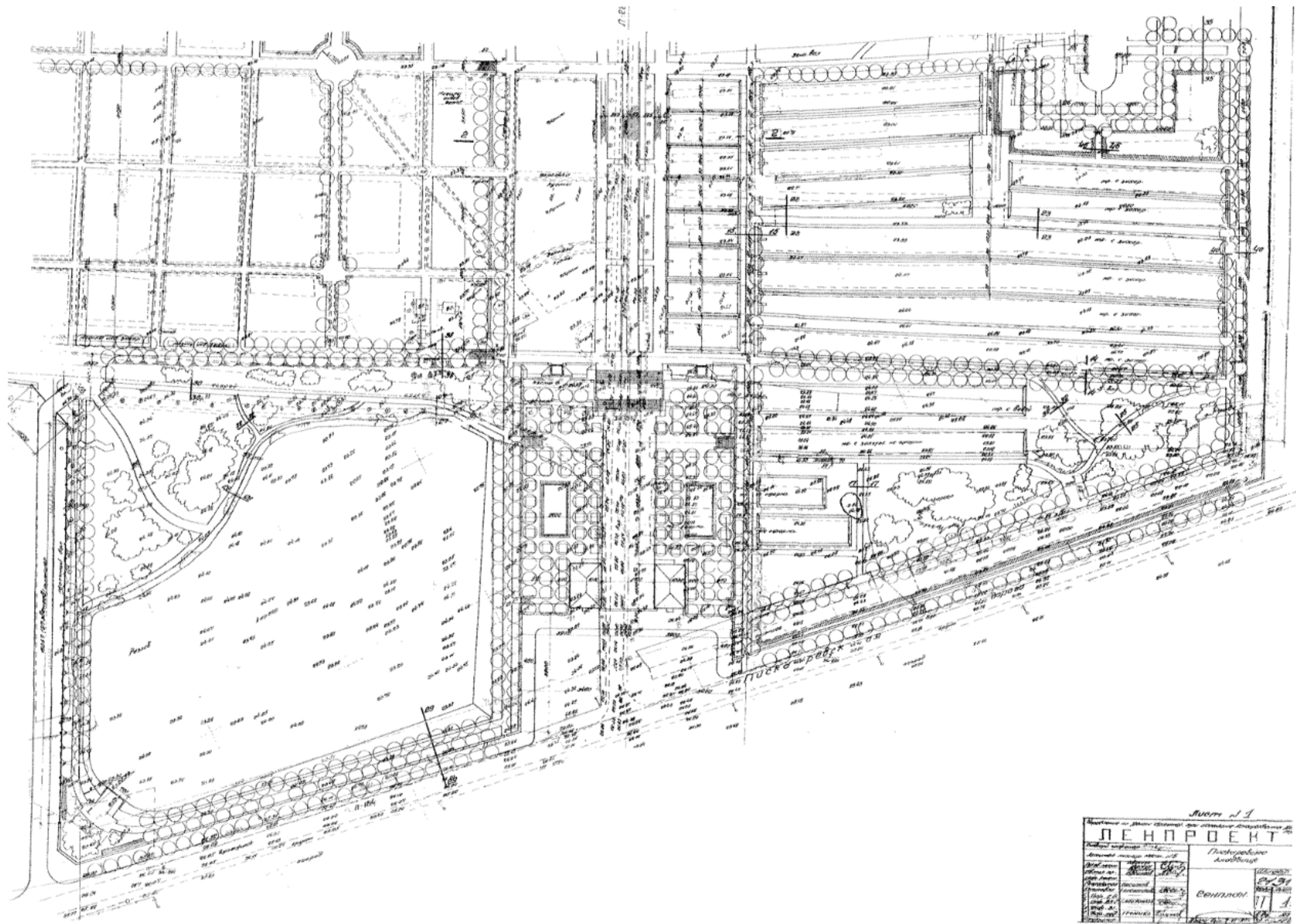
8. Проект устройства Пискаревского мемориального кладбища. Генплан. Ленпроект. 1950 г. // Архив ОАО «ЛенНИИПроект»
