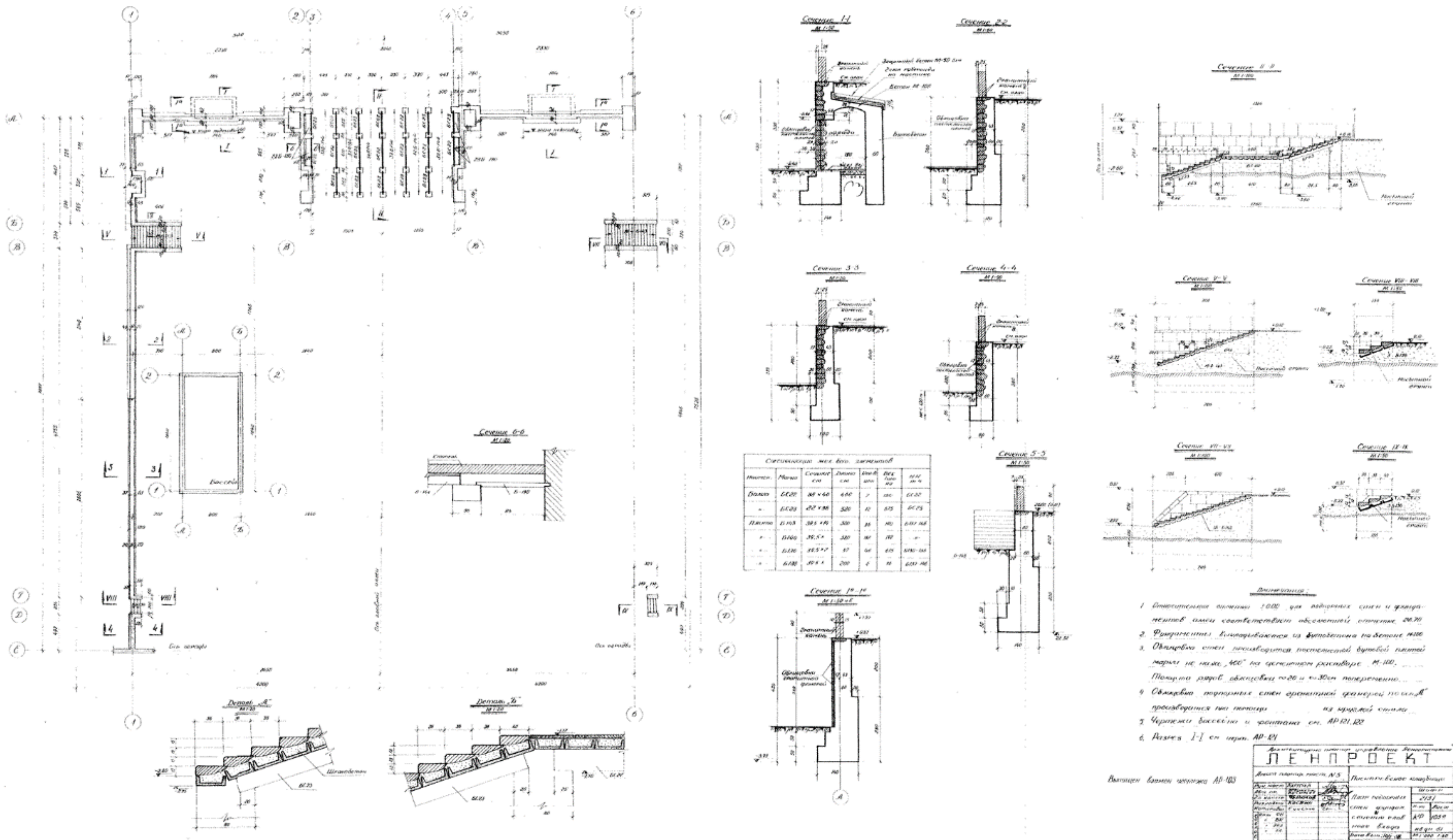
9. Проект устройства Пискаревского мемориального кладбища. План подпорных стенок и лестниц. Ленпроект. 1950 г. // Архив ОАО «ЛенНИИПроект»
