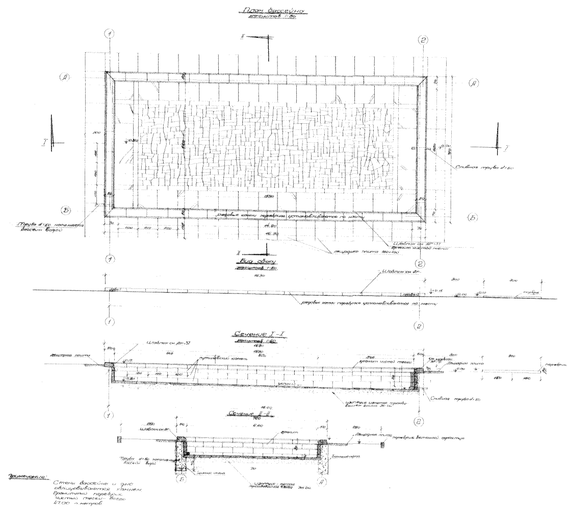
6. Проект устройства Пискаревского мемориального кладбища. План бассейна. Ленпроект. 1950 г. // Архив ОАО «ЛенНИИПроект»
