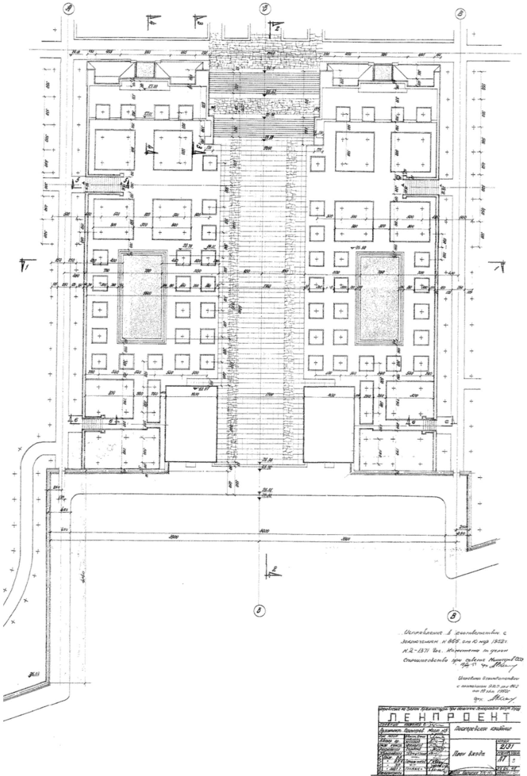
7. Проект устройства Пискаревского мемориального кладбища. План входа. Ленпроект. 1950 г. // Архив ОАО «ЛенНИИПроект»
