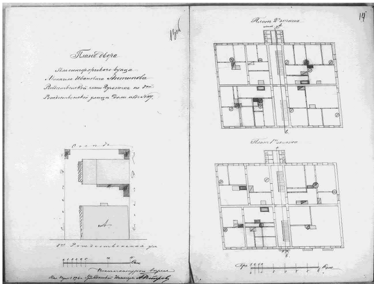
Илл.7. Планы двора и дома Антипова. ЦГИА СПб. Ф. 513. Оп. 102. Д. 9449
