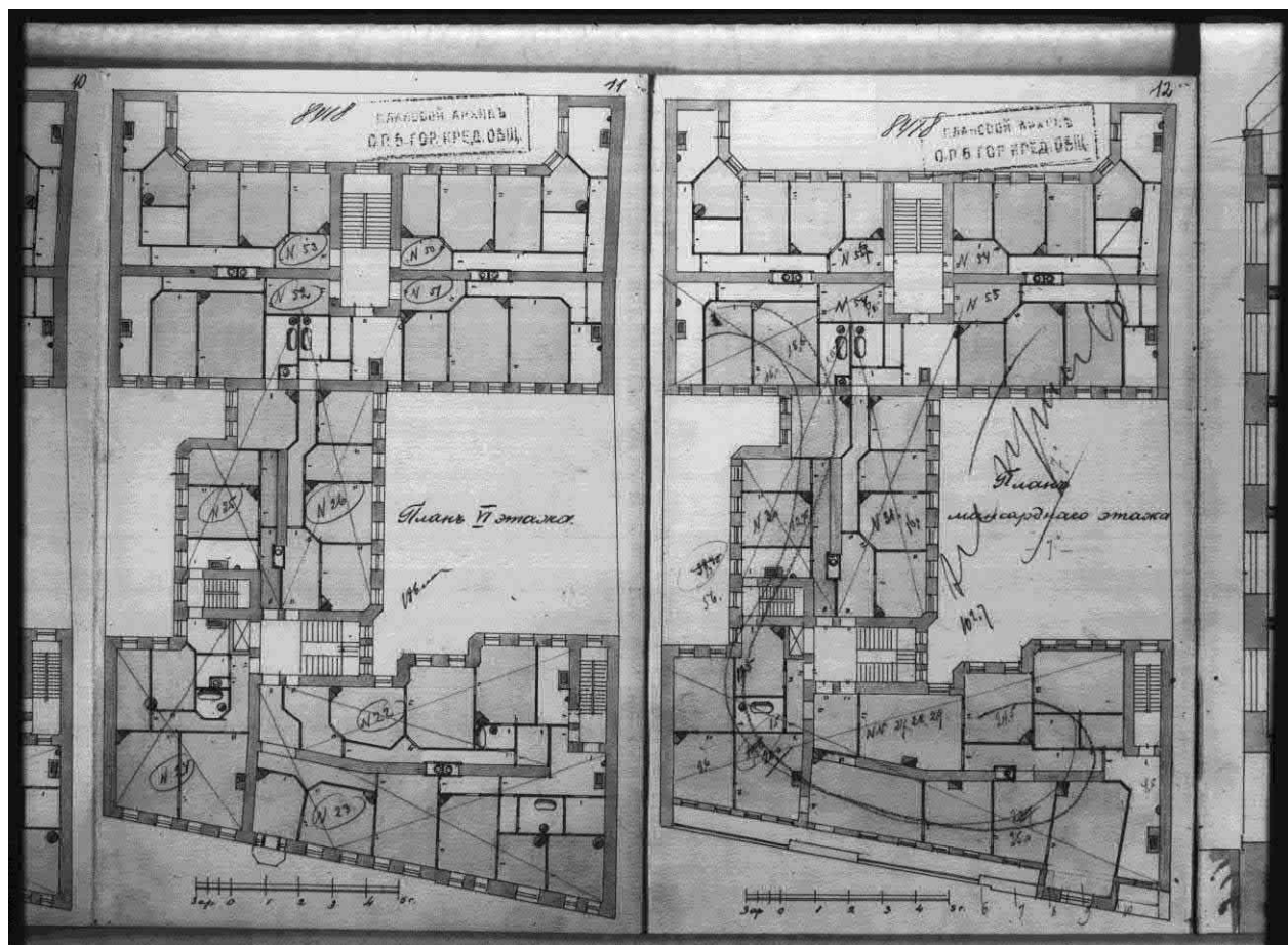
Илл.17. План 17 этажа и мансарды дома Э. Э. Арнольда ЦГИА СПб. Ф. 515. Оп. 4. Д. 5175
