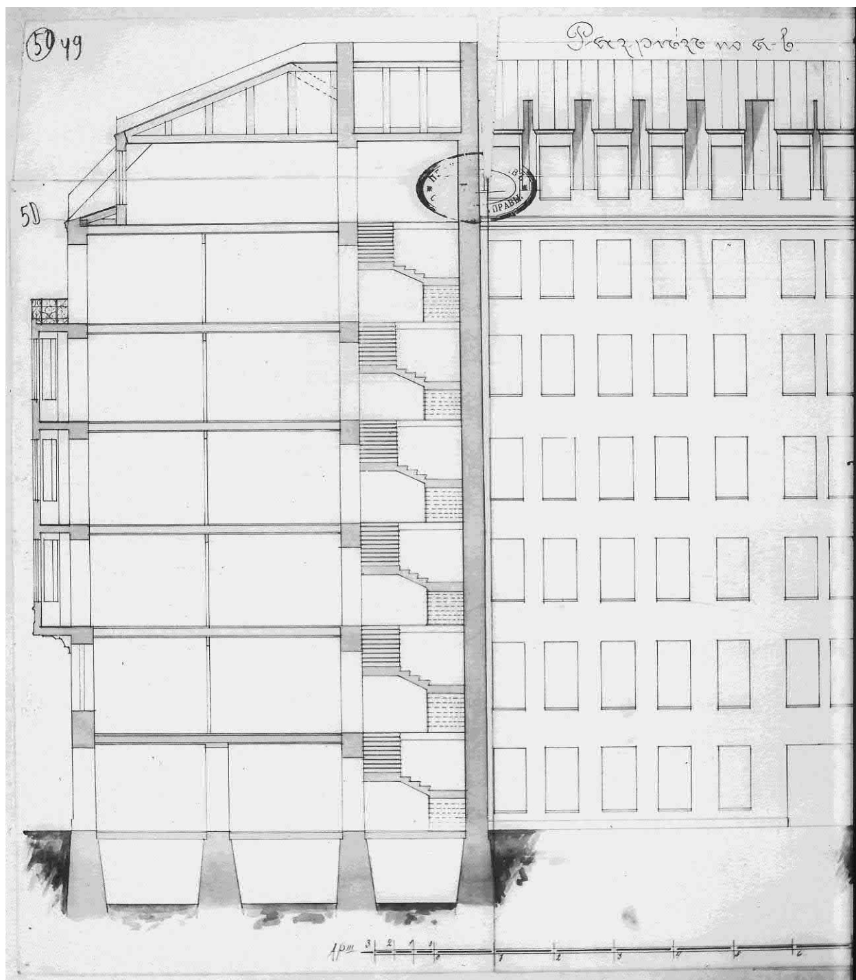
Илл.13. Разрез а-в дома Э. Э. Арнольда. ЦГИА СПб. Ф. 513. Оп. 102. Д. 9449
