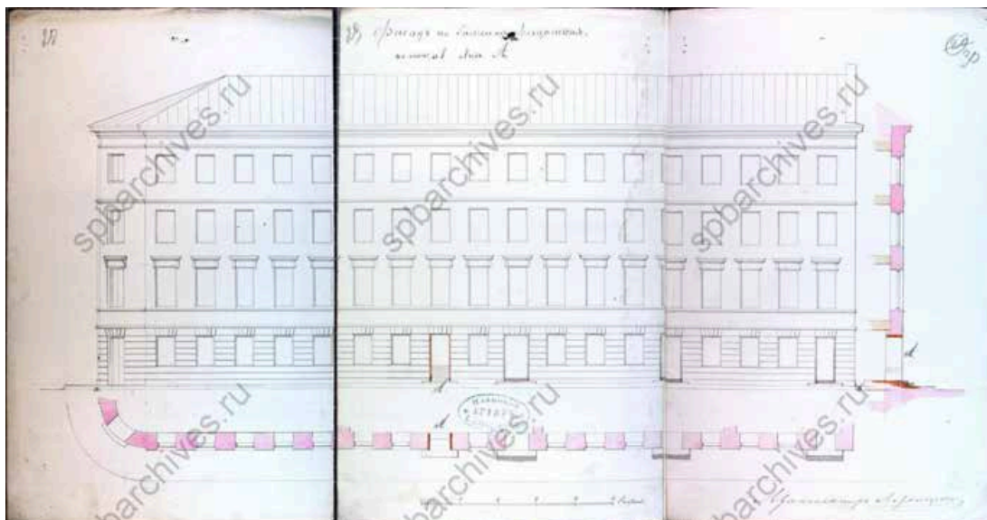
32. ЦГИА СПб. Фонд 513. Опись 102. Дело 3305. 1835-1883 гг. Чертежи дома на участке, принадлежавшем Артемьеву, Е. Артемьевой по Казанской ул., 34 и Демидову пер., 7. Петроградская Городская Управа. Петроград. 1870-1918 гг.
