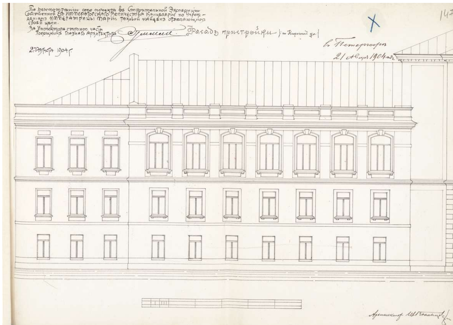
19. Проект расширения института императрицы Марии (реализован с изменениями). Чертеж лицевого фасада 3-этажного (западного) флигеля по Кирочной улице. Арх. И.Н. Коковцев. Утвержден 21 августа 1904 г. // РГИА. Ф. 759. Оп. 25. Д. 298. Л. 147.
