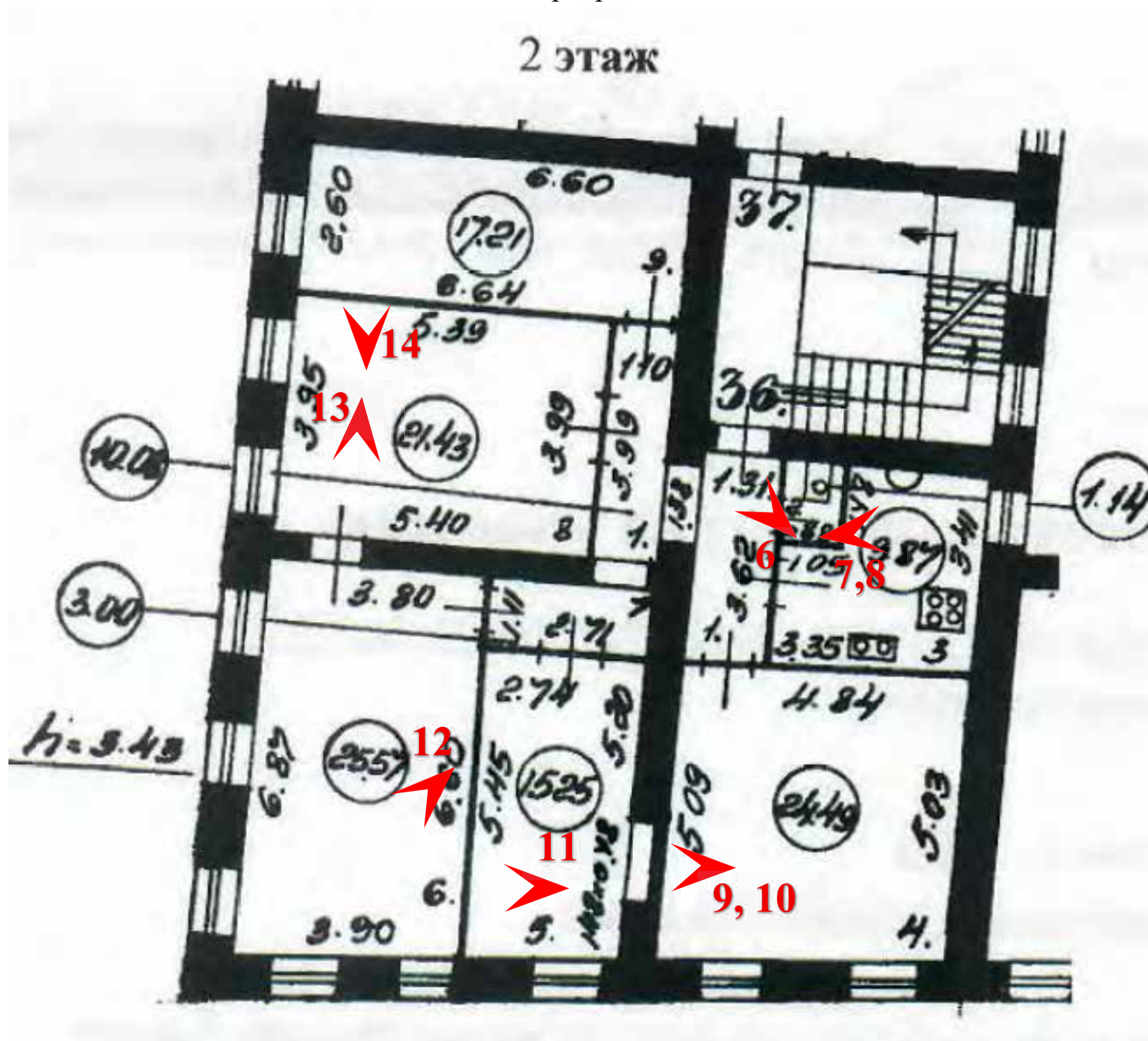
Фрагмент плана 2 этажа Квартира 36
