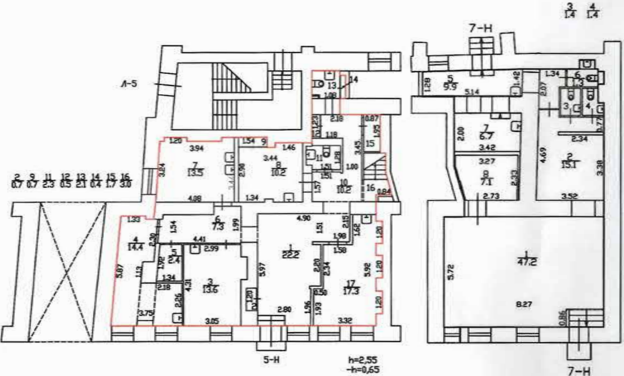
План части цокольного этажа
