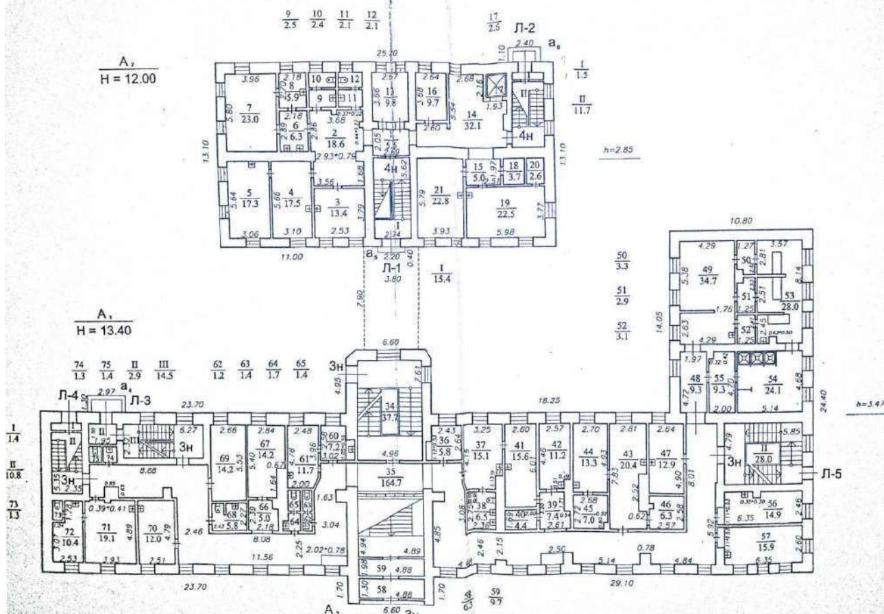
План I этажа
