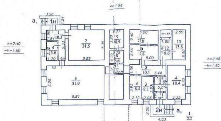
План цокольного этажа
