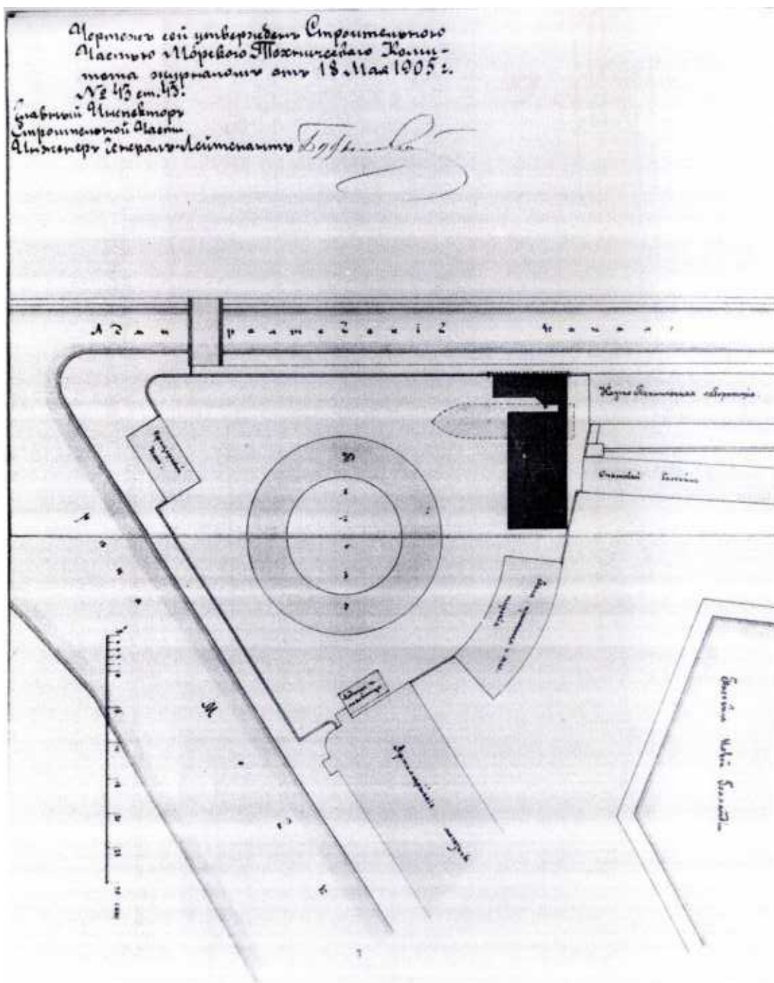
35. Инж. Лебедев, И.И. Тимошук. Проект здания мастерских и бани при тюрьме. Генплан. 1905 г. РГА ВМФ Ф. 409. Оп. 2. Д. 5767.
