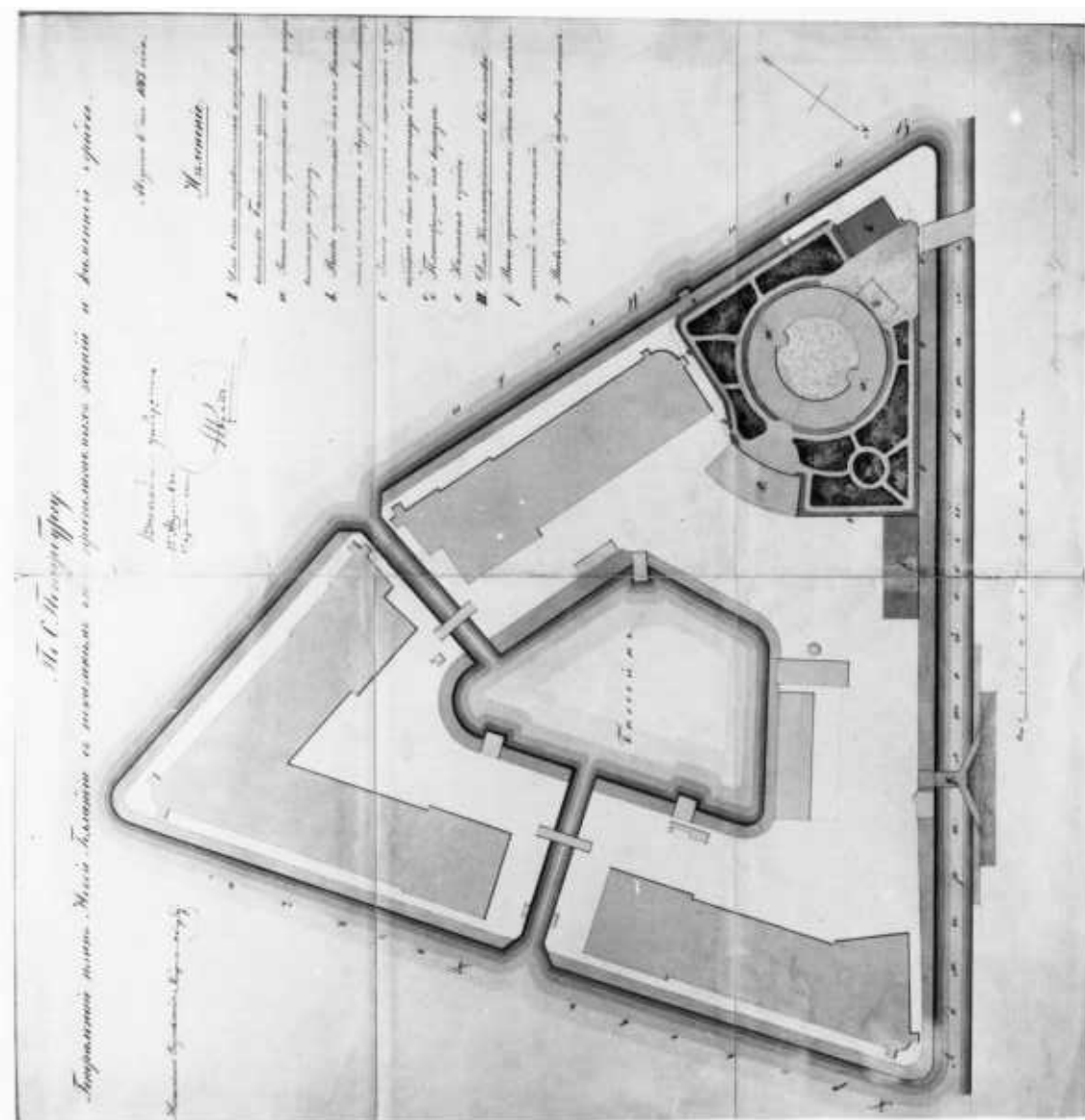
29. Инж. Н. А. Лифантьев. Проект переоборудования здания тюрьмы под военно-исправительную тюрьму Морского ведомства, постройки мясосоольной, комендантского дома, ограды и благоустройства тюремной территории. Генплан. 1863 г. РГА ВМФ. Ф. 326. Оп. 1. Д. 10516.
