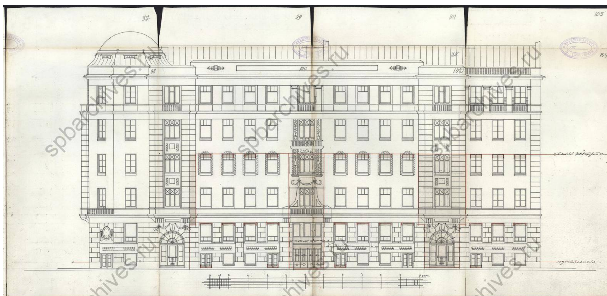
36. Чертежи дома на участке, принадлежавшем М.Волошиновой, Соколову, Ю.К.Додоновой по Большому пр. В.О., 38 и 14-й линии В.О., 11. ЦГИА СПб. Фонд 513. Опись 102. Дело 1208
