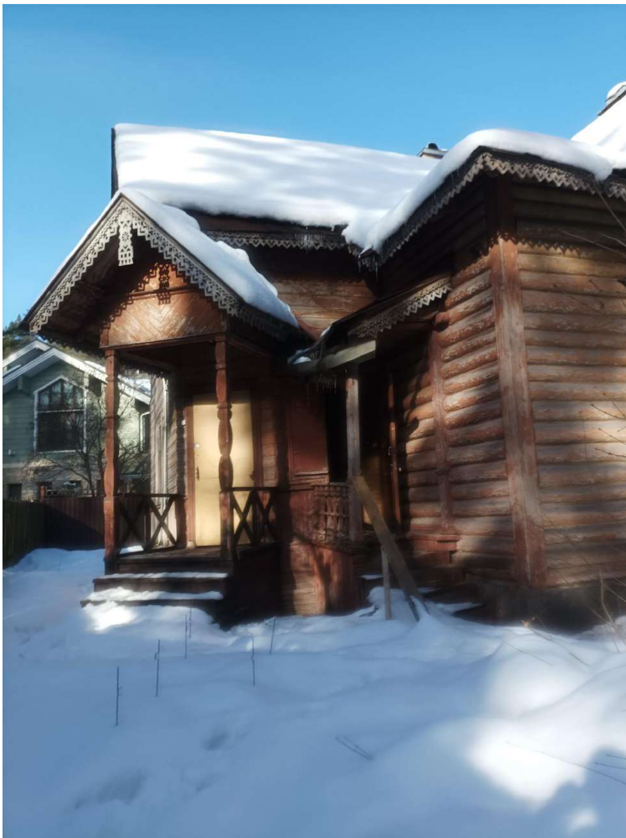
Фото 12. Вид на южный фасад объекта культурного наследия регионального значения «Дача Е. Н. Макаровой (семьи академика А. Е. Фаворского)».
