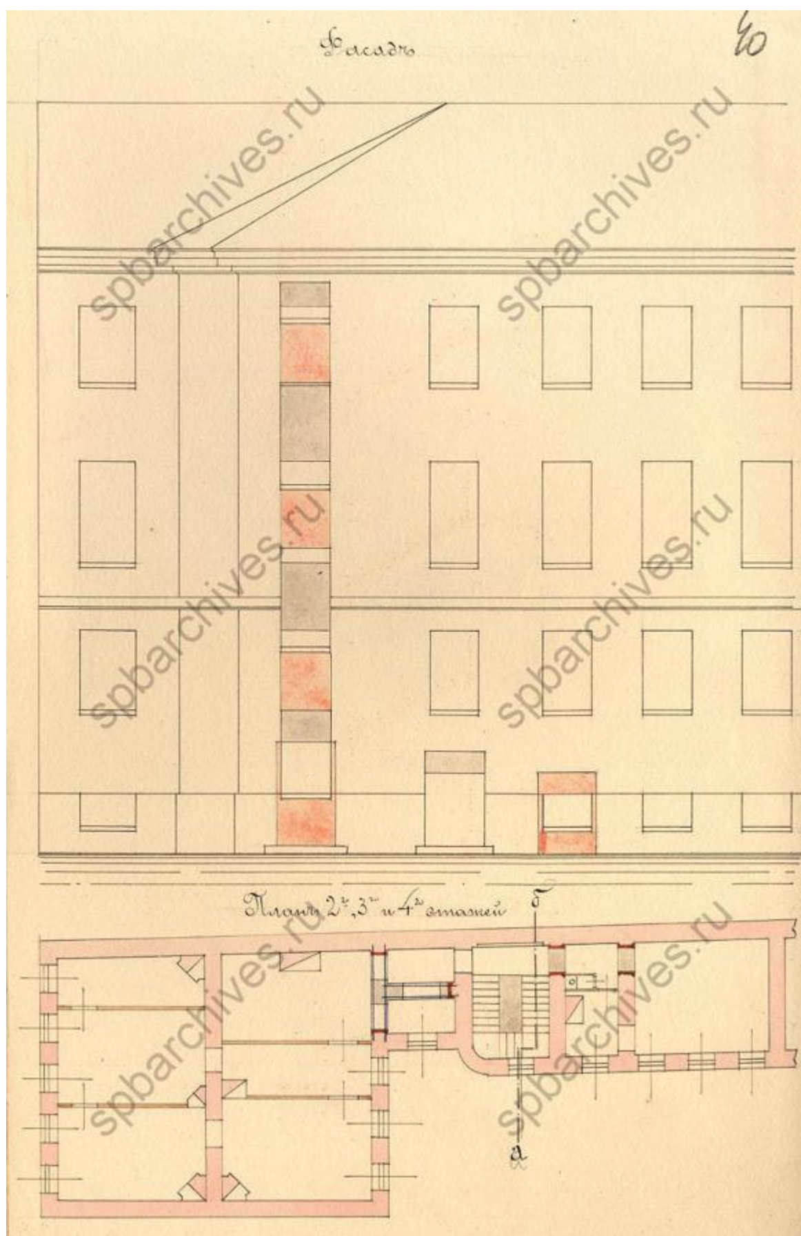
Илл. 11. Фрагмент фасада и поэтажного плана (2-4-й этажи) над исследуемой квартирой.
