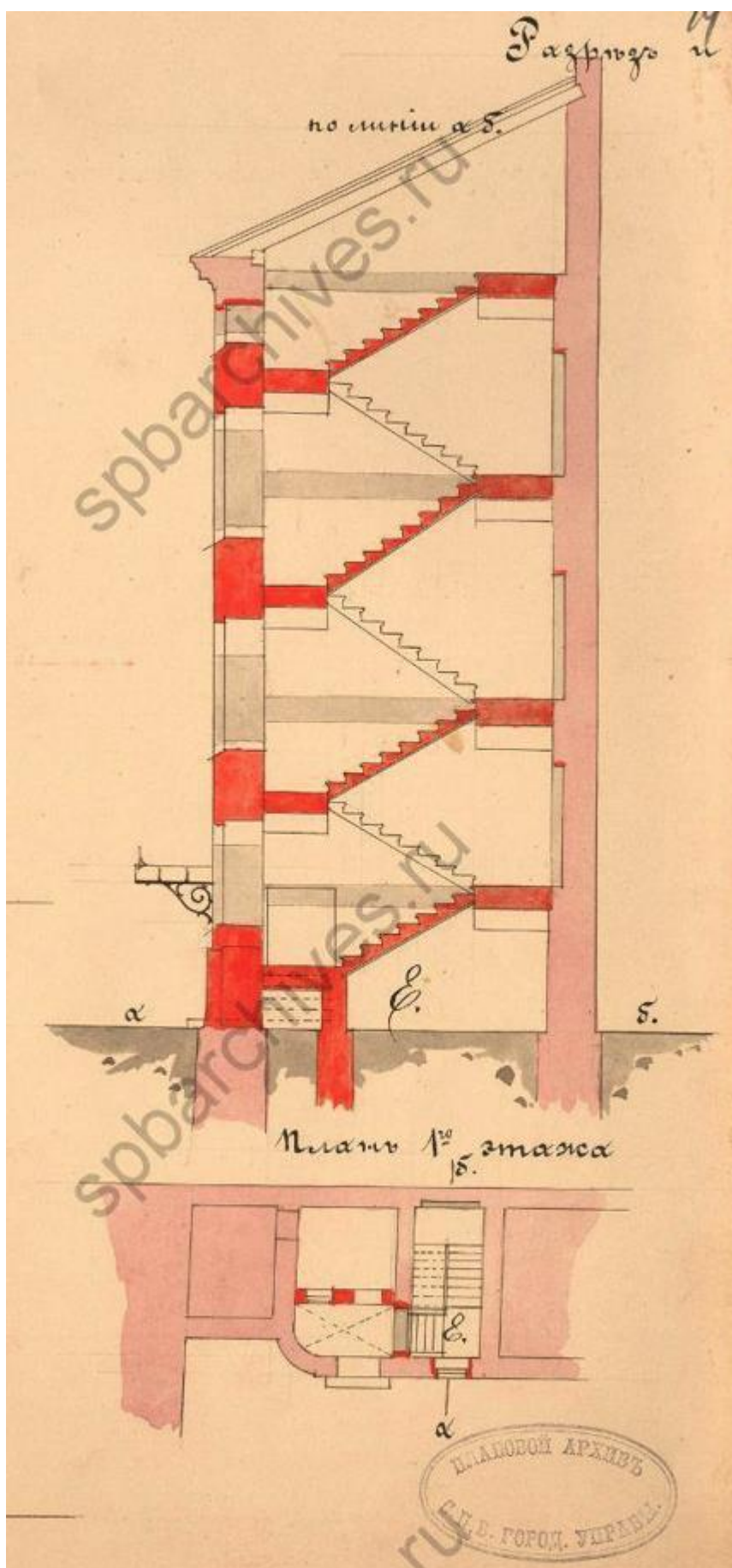
Илл. 8. Разрез и фрагмент плана 1-го этажа помещения, смежного с исследуемым. Дата: 1884 г. Источник: ЦГИА СПб, ф. 513, оп. 102, д. 5332.
