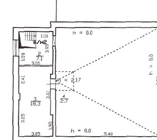
План чердака
