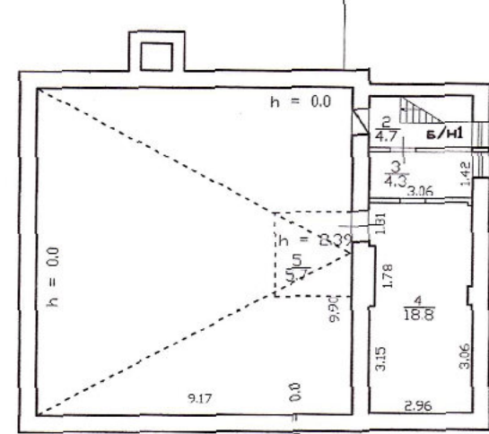
План чердака
