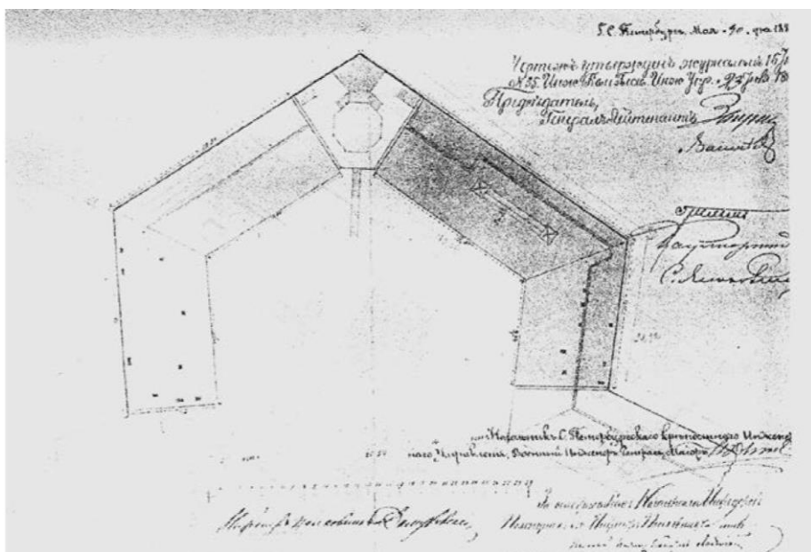
19. План Флагшточной башни. Деталь проектного чертежа по устройству металлического покрытия башни Нарышкина. 1887 г. РГА ВМФ. Ф. 3/л. Оп. 35. Д. 5936.
