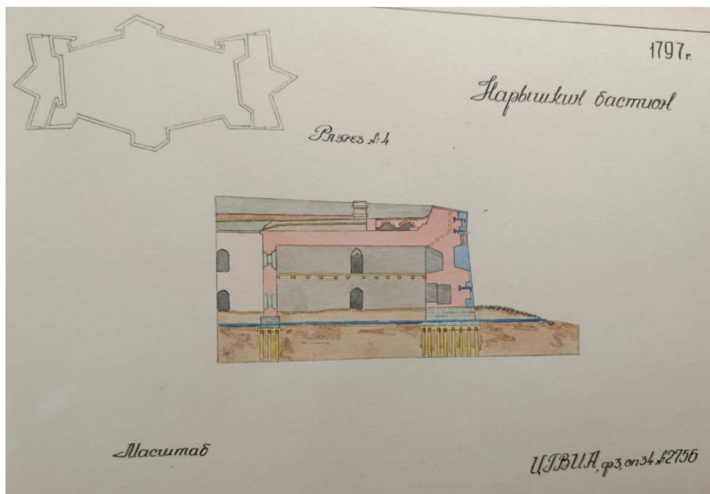
10. Кожевников А.С. Петропавловская крепость. Нарышкин бастион. Разрез 4. Чертеж. 1797 г. РГВИА. Ф. 3. Оп. 34. Д. 2756.
