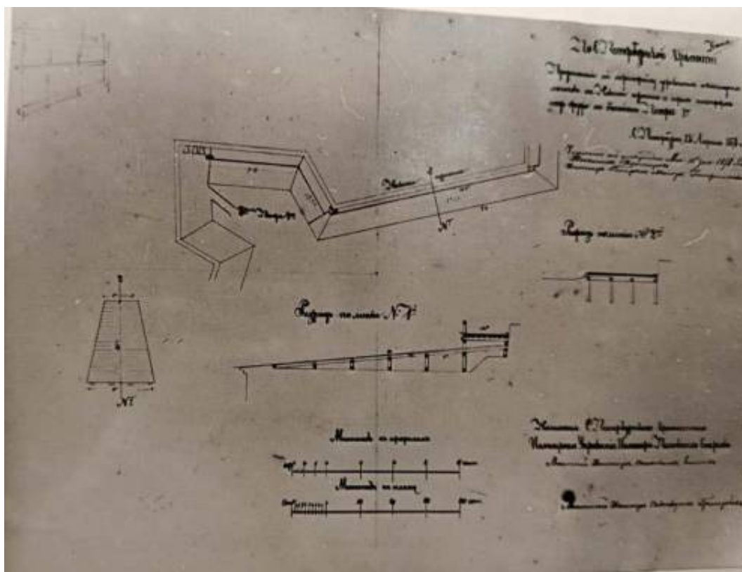
23. Предположение на перестройку деревянных пешеходных мостиков на Невской куртине. 1878 г. РГВИА (ЦГВИА). Ф. 16082. Оп. 2. Д. 625. Л. 1.
