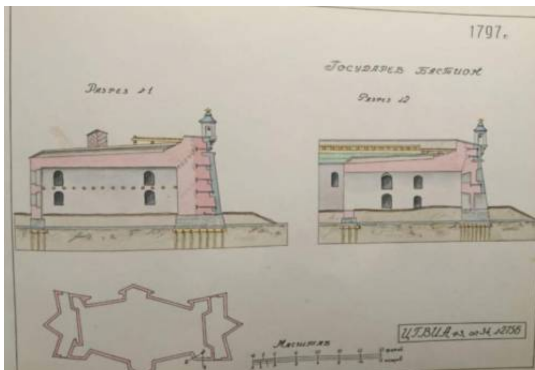
11. Кожевников А.С. Петропавловская крепость. Государев бастион. Разрез 1,2. Чертеж. 1797 г. РГВИА (ЦГВИА). Ф. 3. Оп. 34. Д. 2756.
