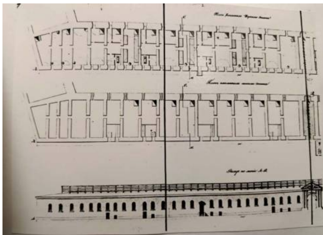
19. Чертеж казематов Невской куртны. Фрагмент. 1844 г. РГА ВМФ. Ф. 3/л. Оп. 34. Д. 3805.
