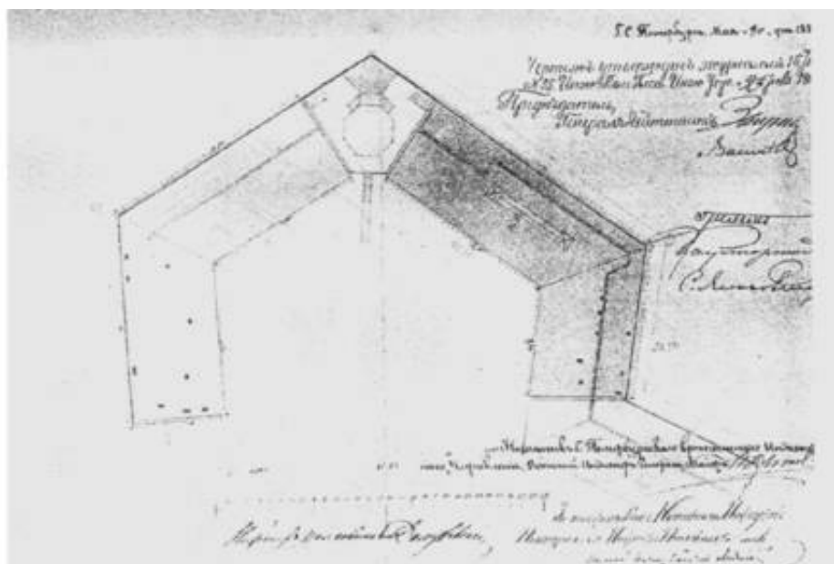
24. План Флагшточной башни. Деталь проектного чертежа по устройству металлического покрытия бастиона Нарышкина. 1887 г. РГА ВМФ. Ф. 3/л. п. 35. Д. 5936.
