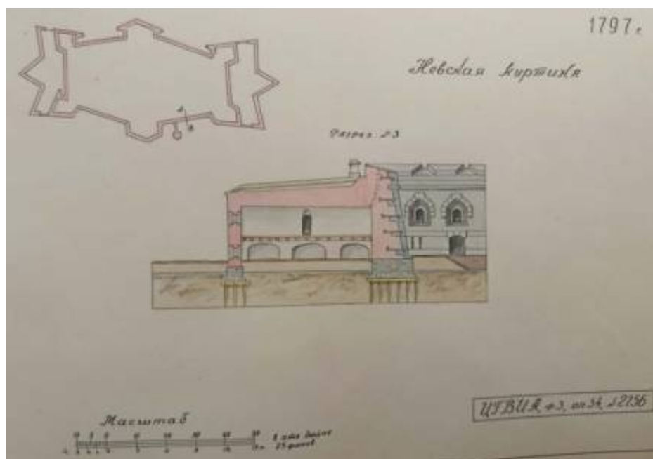
10. Кожевников А.С. Петропавловская крепость. Невская куртина. Разрез 3. Чертеж. 1797 г. РГВИА (ЦГВИА). Ф. 3. Оп. 34. Д. 2756.
