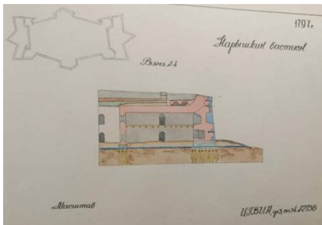
12. Кожевников А.С. Петропавловская крепость. Нарышкин бастион. Разрез 4. Чертеж. 1797 г. РГВИА (ЦГВИА). Ф. 3. Оп. 34. Д. 2756.
