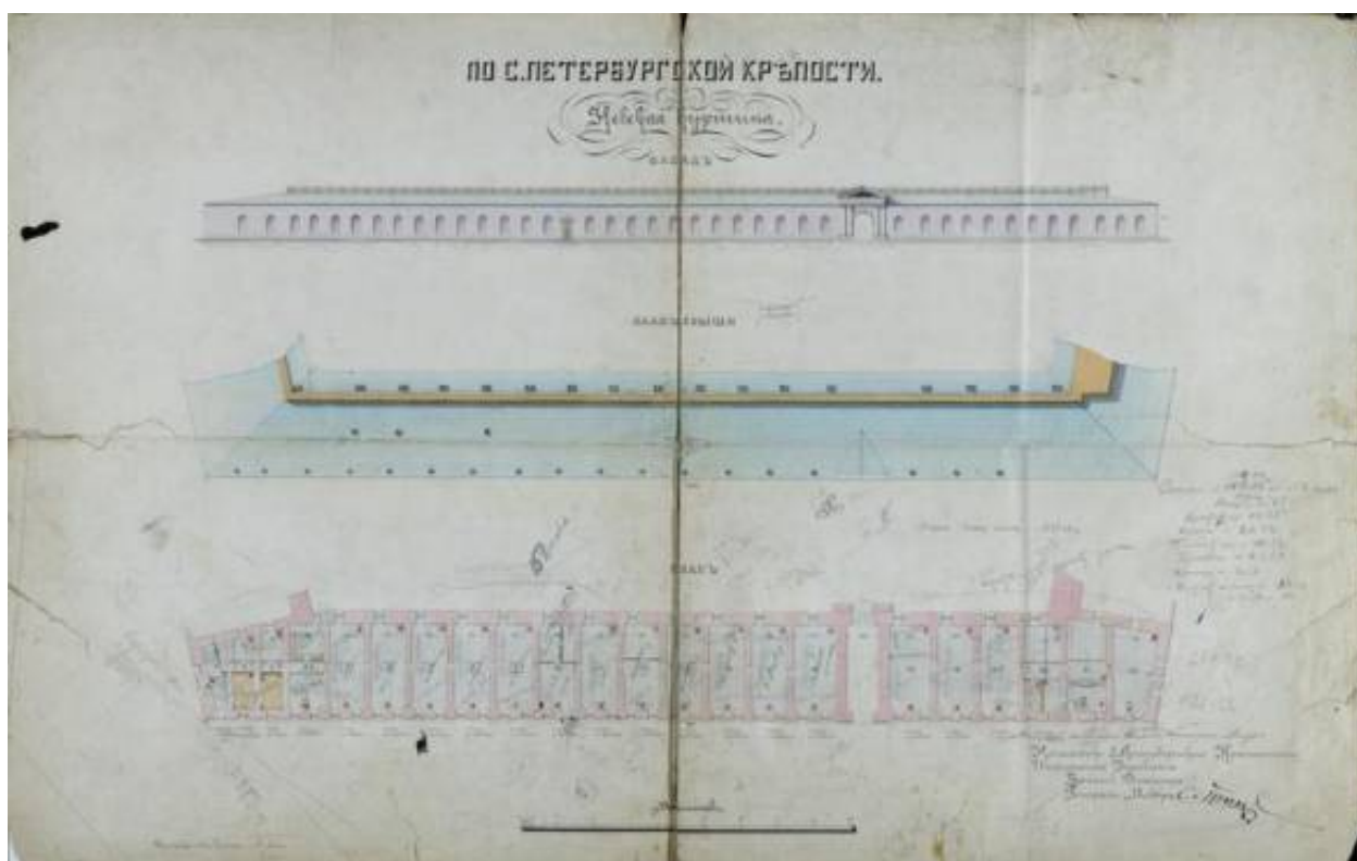
25. По С. Петербургской крепости. Невская куртина. Фасад. План крыши. План. 1890 г. РГА ВМФ. Ф. 3/л Оп. 35. Д. 5964.
