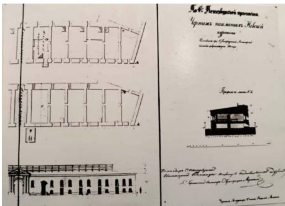
18. Чертеж казематов Невской куртны. Фрагмент. 1844 г. РГА ВМФ. Ф. 3/л. Оп. 34. Д. 3805.
