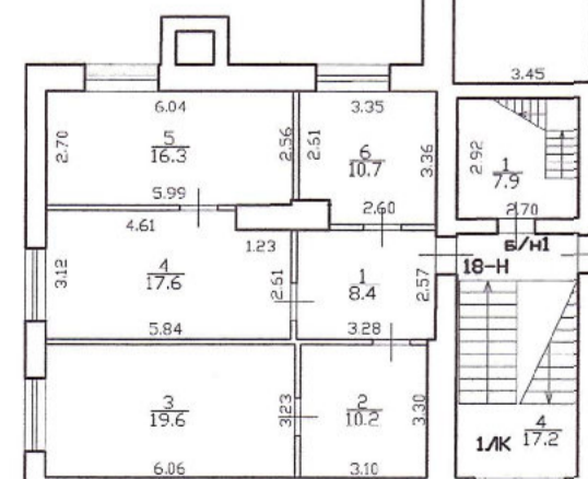
План 4 этажа
