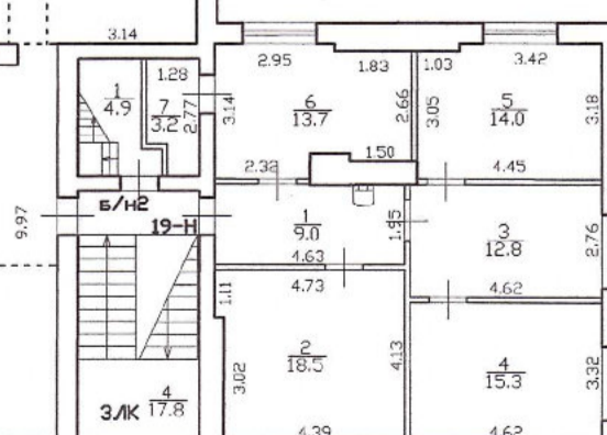
План 4 этажа
