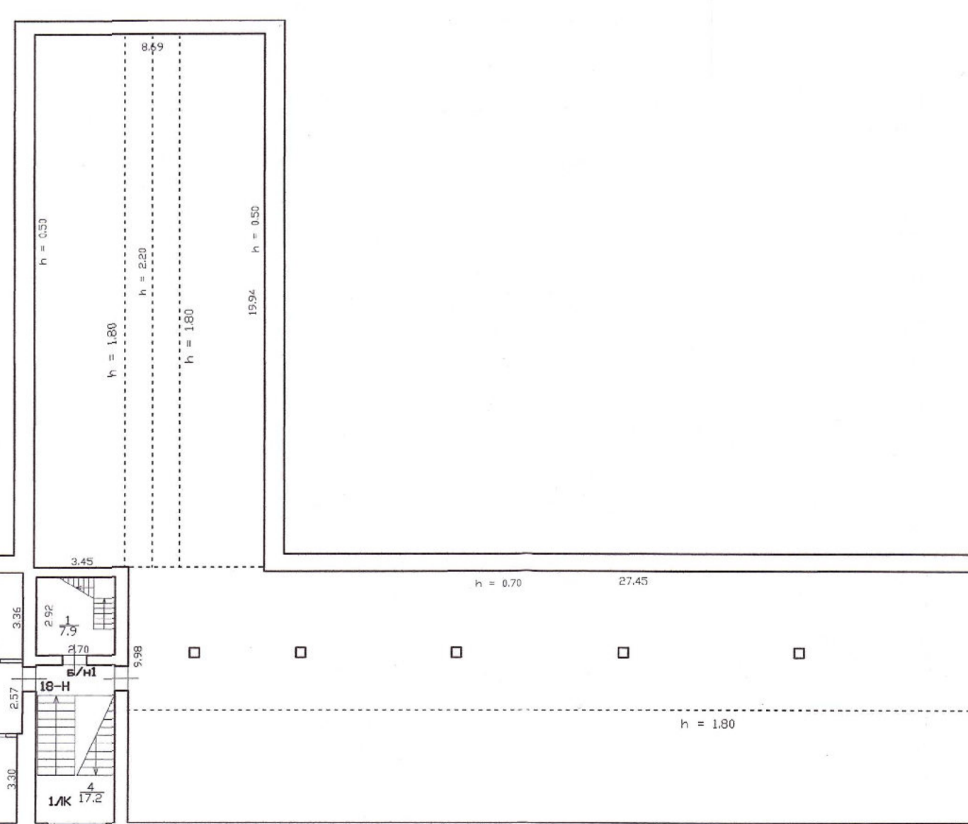
План чердака
