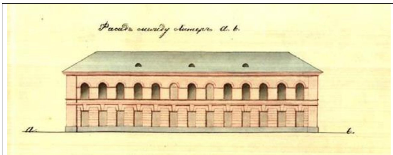
8. Фасад каменного 2-этажного здания для ледников и Анатомического театра при Военном Морском госпитале. Фрагмент. РГА ВМФ Ф. 326, оп. 1, д. 6221
