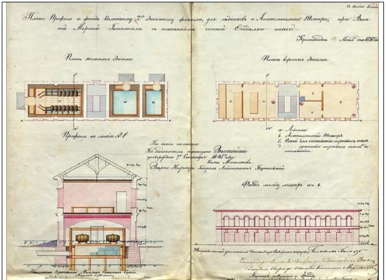
10. План, профиль и фасад каменному 2-хэтажному флигелю Анатомическому театру при Военной Морской госпитали с показанием чистой отделки оного. Кронштадт. 11 мая 1850 года. Составил инженер Штабс Капитан Мартынов». РГА ВМФ Ф. 326, оп. 1, д. 6669.
