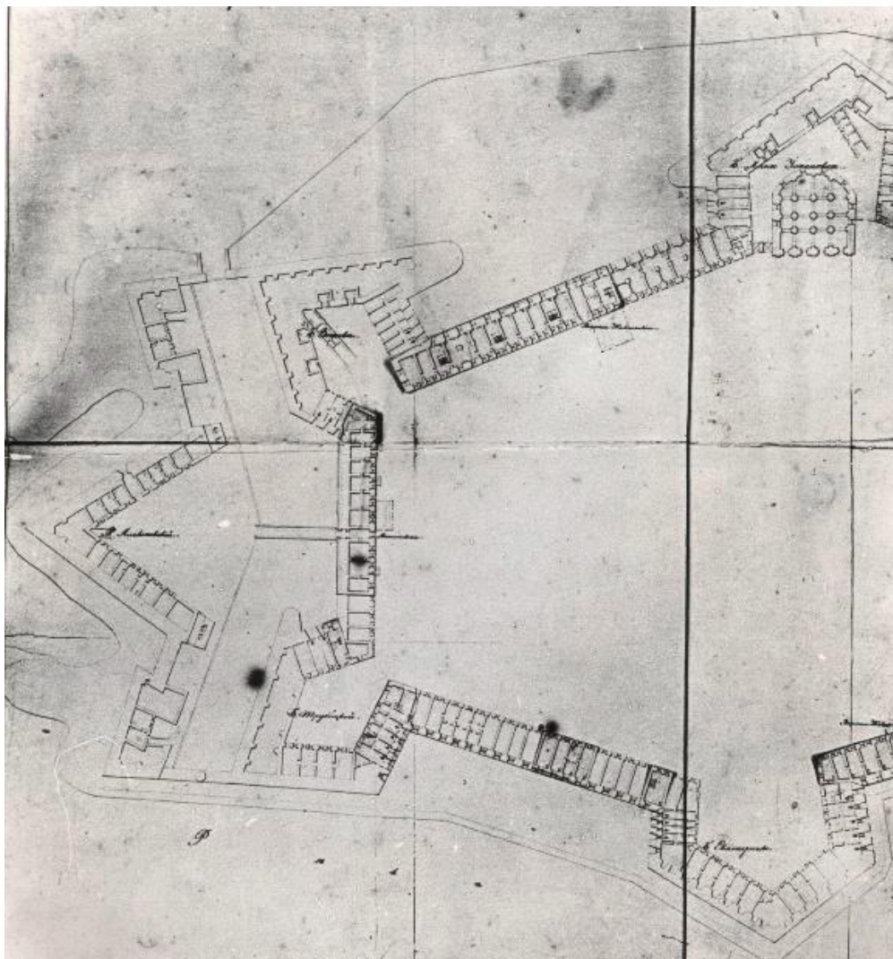
14. Фрагмент генерального плана СПб-й крепости. 1835 г. РГА ВМФ. Ф. 3/л. Оп. 34. Д. 3534.
