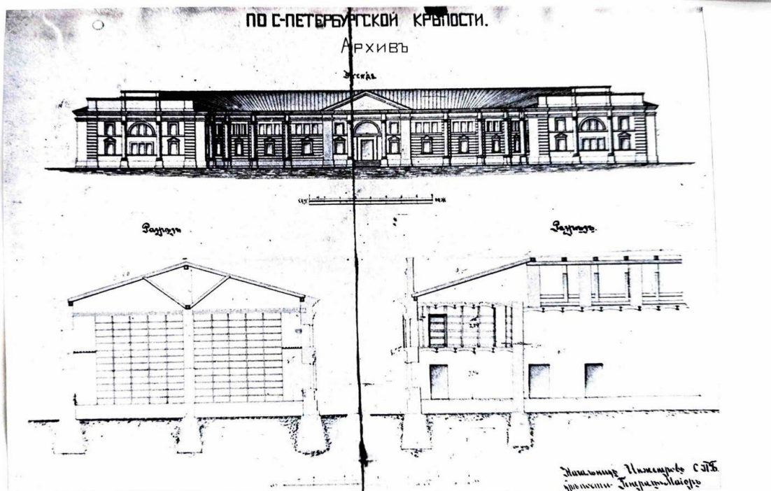
19. Чертеж зданий архивов Главных Управлений Военного Министерства. 1892 г. РГА ВМФ. Ф. 3/л. Оп. 35. Д. 5995.
