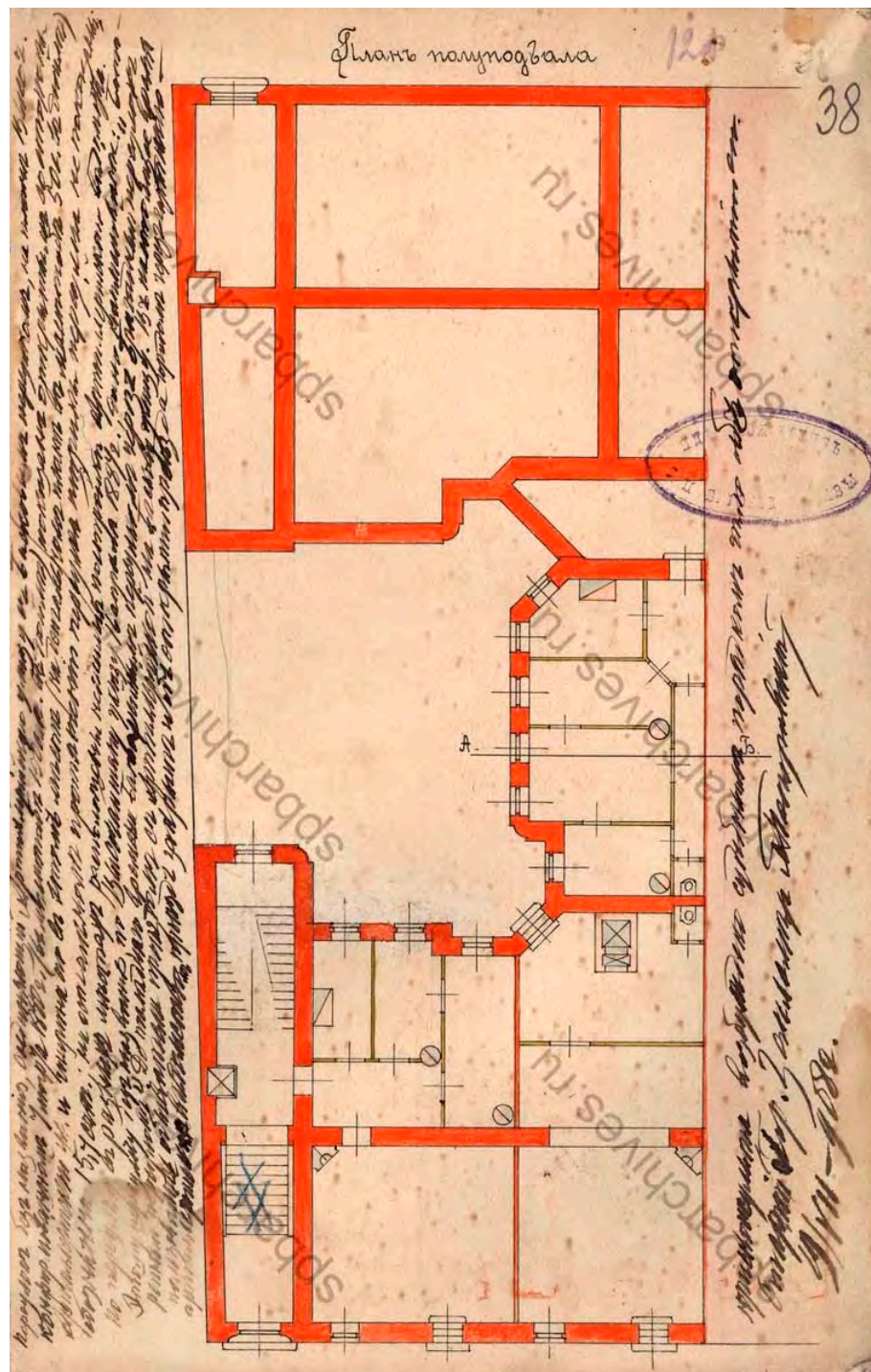
Илл. 18. План полуподвала. 1908 г. ЦГИА СПб. Ф. 513. Оп. 102. Д. 4306. Л. 38.
