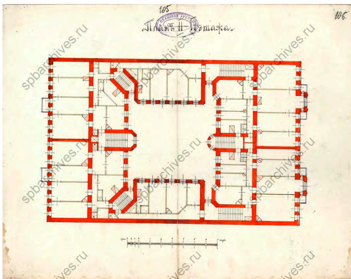
Илл. 35. План 2-6 этажа. 1903 г. ЦГИА СПб. Ф. 513. Оп. 102. Д. 4306. Л. 105-106.
