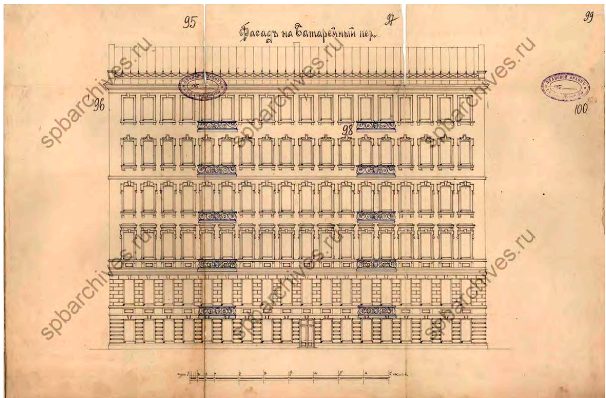
Илл. 32. Фасад на Батарейный переулоч. 1903 г. ЦГИА СПб. Ф. 513. Оп. 102. Д. 4306. Л. 95-100.
