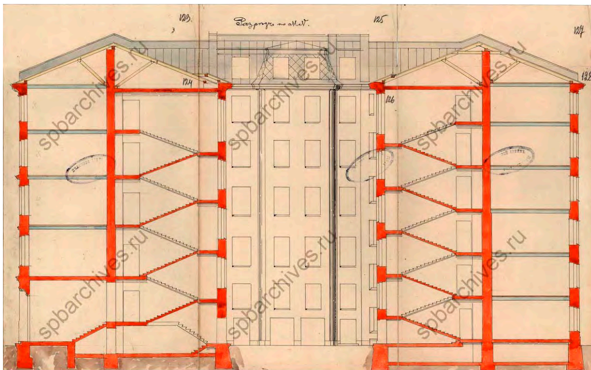
Илл. 43. Разрез по MN. 1905 г. ЦГИА СПб. Ф. 513. Оп. 102. Д. 4306. Л. 123-128.
