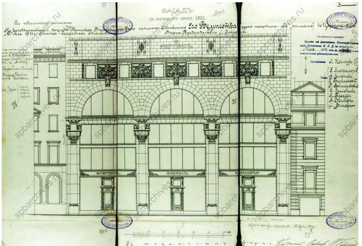
Илл. 43. Фасад по Невскому пр. № 21 Торгового дома Ф. Л. Мертенс. 1911.
