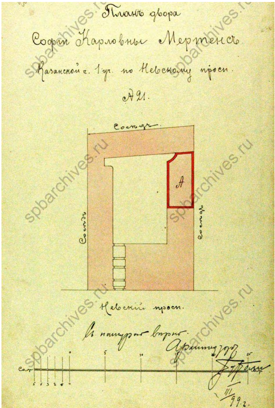
Илл. 26. План двора дома С. К. Мертенс. 1899. Проект перedelки каменного 3х этажного на подвале надворного флигеля. ЦГИА СПб. Ф. 513. Оп. 102. Ф. 3420. Л. 40об.
