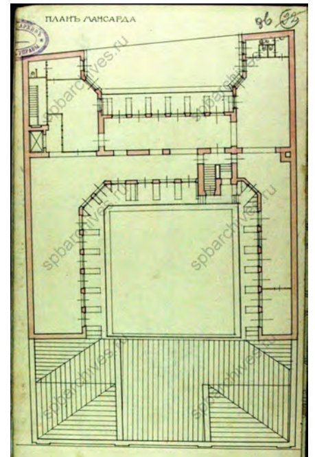
План мансарды
