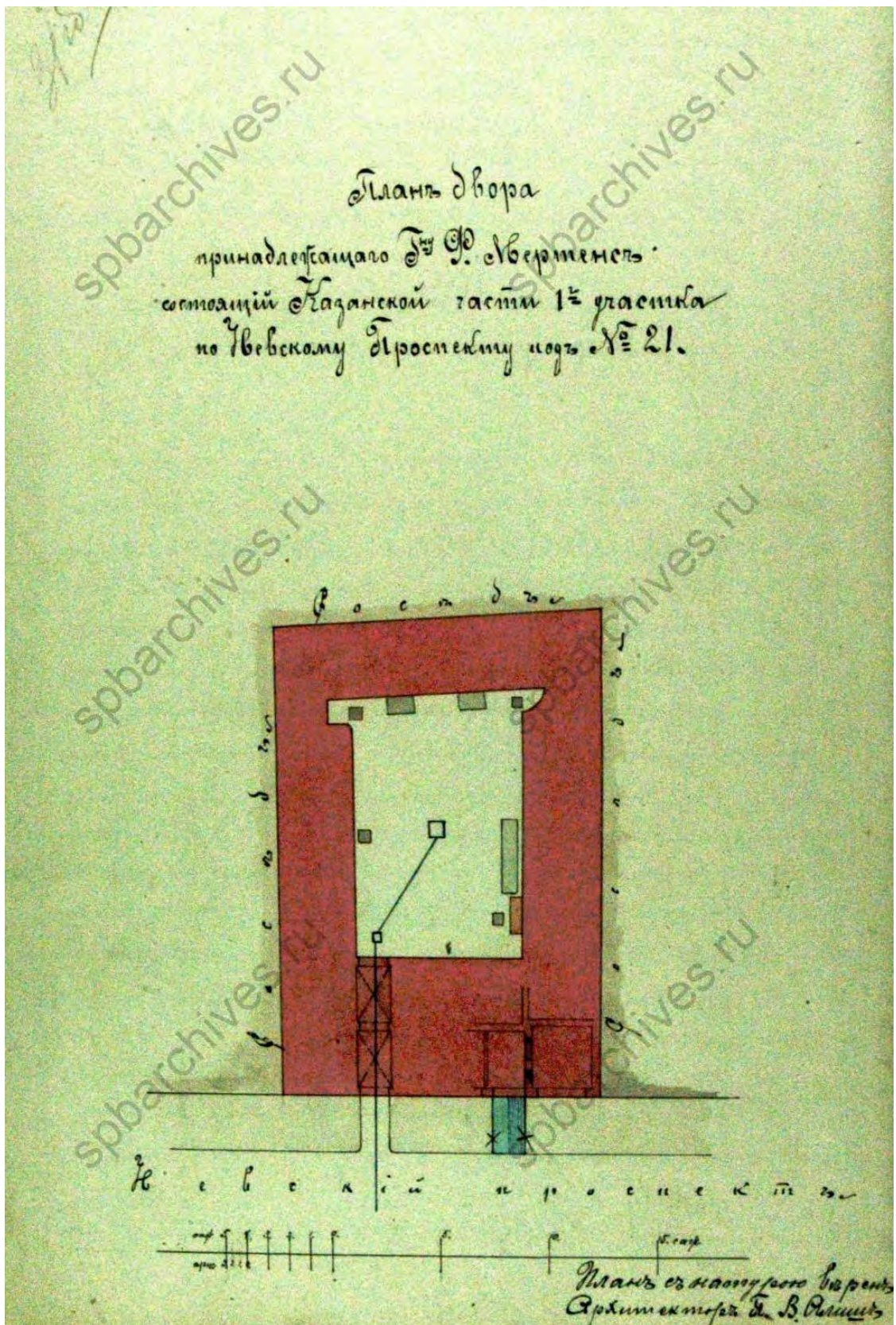
Илл. 19. План двора дома Ф. Мертенса. 1887. Архитектор Я.В. Алиш. Проект устройства внутреннего проема в пожарной стене первого этажа и переделки тамбура входа. ЦГИА СПб. Ф. 513. Оп. 102. Ф. 3420. Л. 31об.
