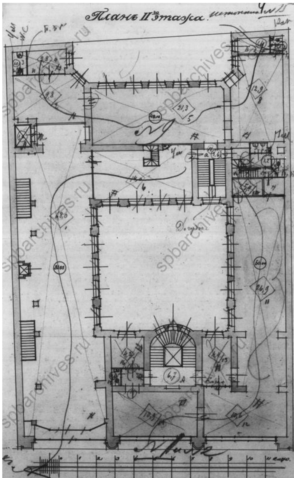
Илл. 55. План 2-го этажа дома Торгового дома Ф. Л. Мертенс. 1913. ЦГИА СПб. Ф. 515. Оп. 4. Д. 3887. Л. 4.
