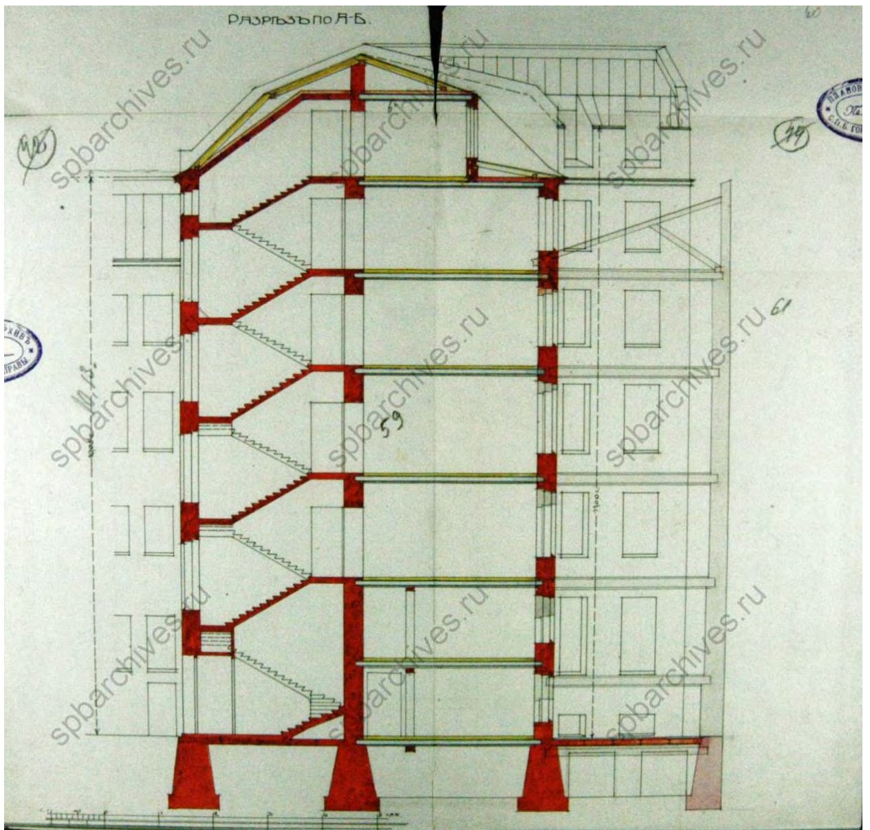
Илл. 40. Разрез А-Б дворового флигеля Торгового дома Ф. Л. Мертенса и наследников Ф. Л. Мертенса. 1911. Архитектор М. С. Лялевич.
