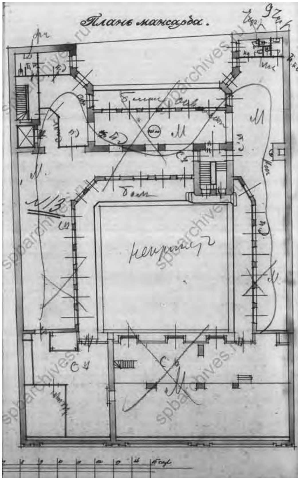
Илл. 59. План мансарды дома Торгового дома Ф. Л. Мертенс. 1913. ЦГИА СПб. Ф. 515. Оп. 4. Д. 3887. Л. 9.
