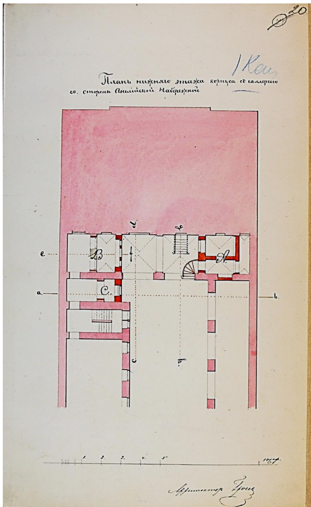
Илл.15. Арх. Г.Ф. Гросс. План нижнего этажа корпуса по Английской набережной («набережного Дома») с галереей. 1871 г. ЦГИА СПб. Ф. 513. Оп. 102. Д. 75, л.20.
