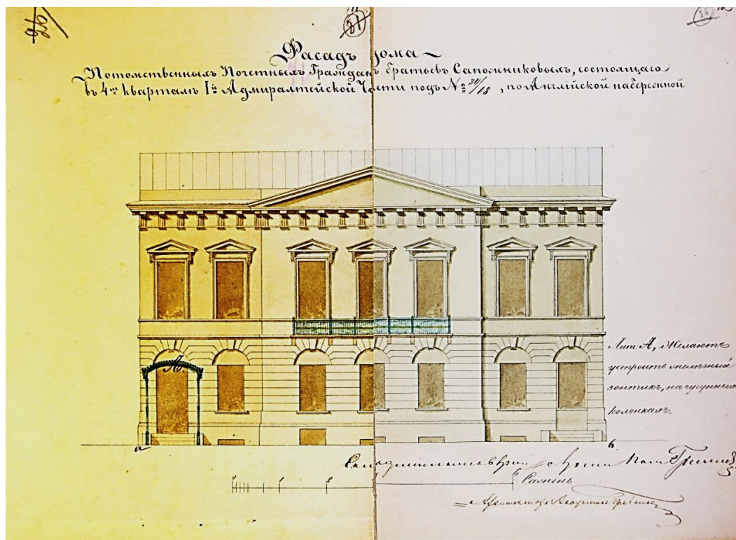
Илл.11. Главный (лицевой) фасад «набережного Дома». Проект устройства металлического зонтика на чугунных колонках над парадной дверью по фасаду со стороны Английской набережной. 1856 г. ЦГИА СПб. Ф. 513. Оп. 102. Д. 75, лл.11-12.
