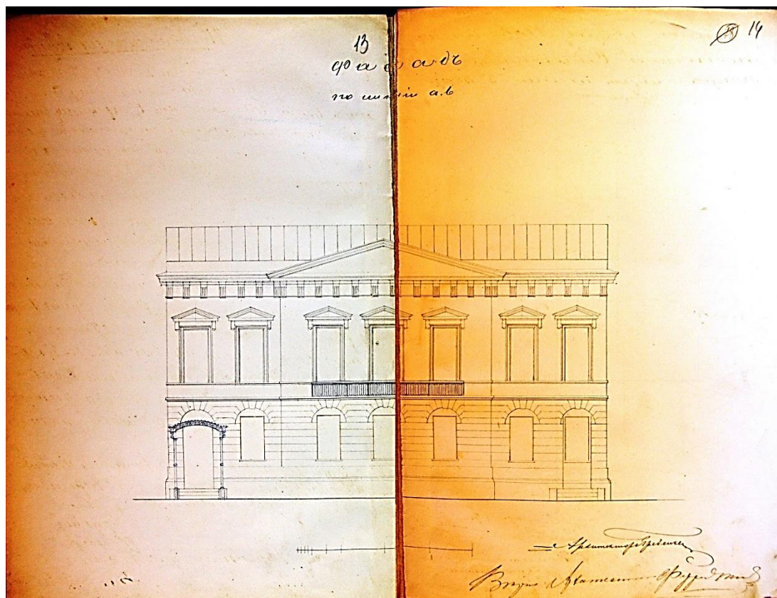
Илл.12. Главный (лицевой) фасад «набережного Дома». Проект устройства металлического козырька над парадной дверью по фасаду со стороны Английской набережной. 1856 г. Фасад по линии а-в. ЦГИА СПб. Ф. 513. Оп. 102. Д. 75, лл.13-14.
