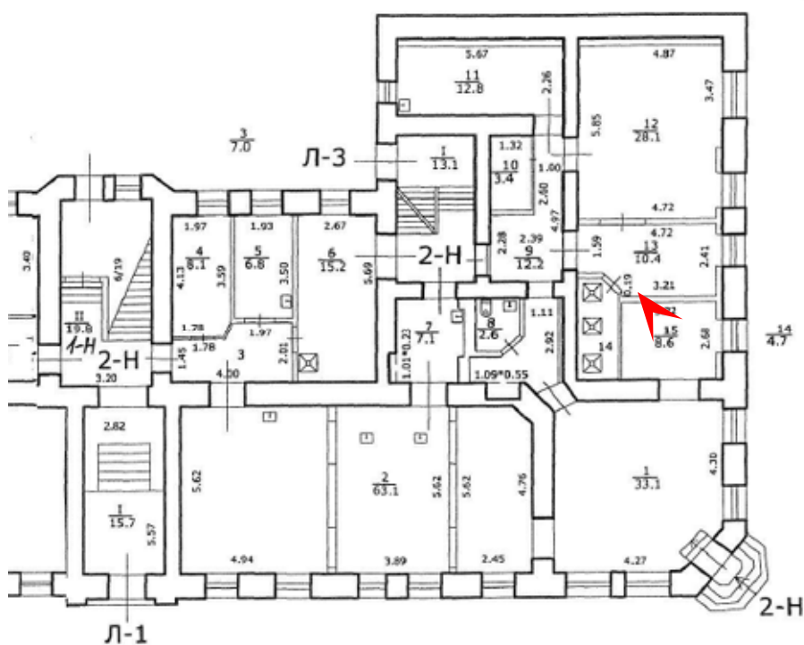
15. Объект культурного наследия регионального значения «Доходный дом Ю.К. Добберт» по адресу: улица Лизы Чайкиной, дом 4/12, литера А Фрагмент плана 1 этажа. Пом. 2-Н Дата съемки: 25.05.2026
