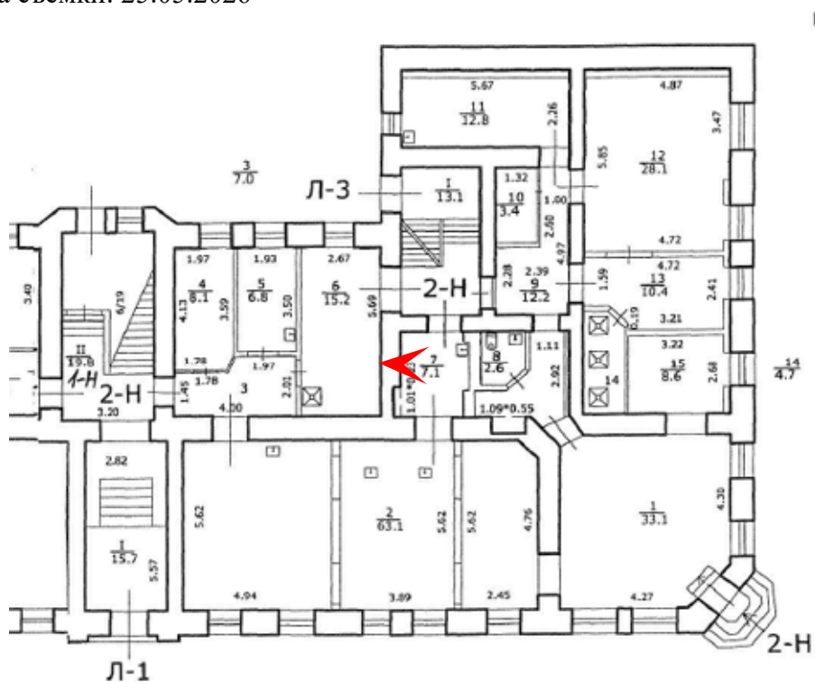
31. Объект культурного наследия регионального значения «Доходный дом Ю.К. Добберт» по адресу: улица Лизы Чайкиной, дом 4/12, литера А Фрагмент плана 1 этажа. Пом. 2-Н Дата съемки: 25.05.2026
