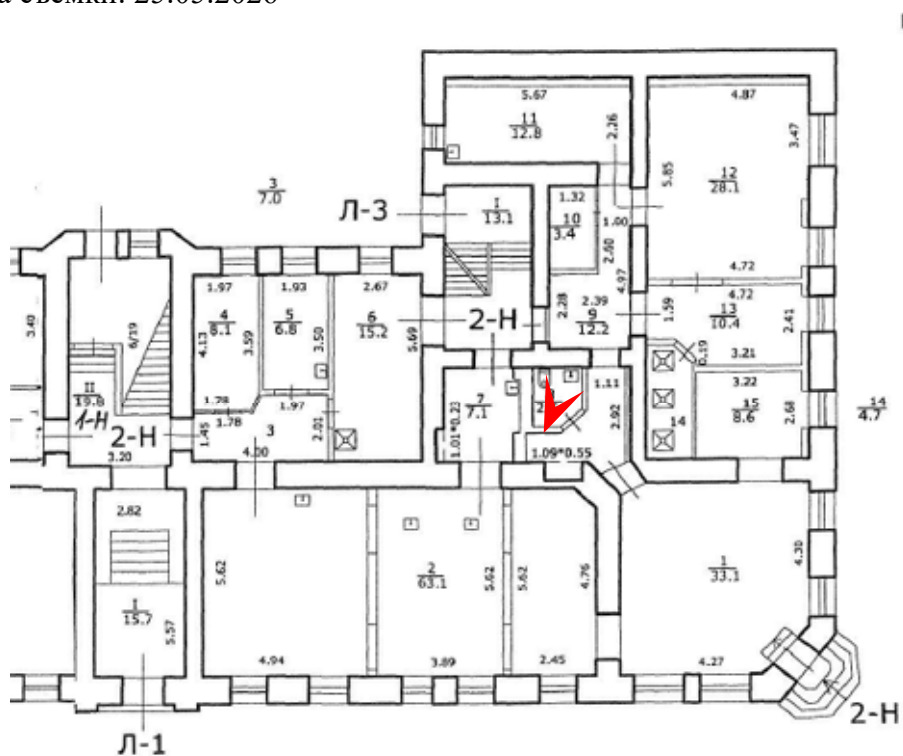
23. Объект культурного наследия регионального значения «Доходный дом Ю.К. Добберт» по адресу: улица Лизы Чайкиной, дом 4/12, литера А Фрагмент плана 1 этажа. Пом. 2-Н Дата съемки: 25.05.2026
