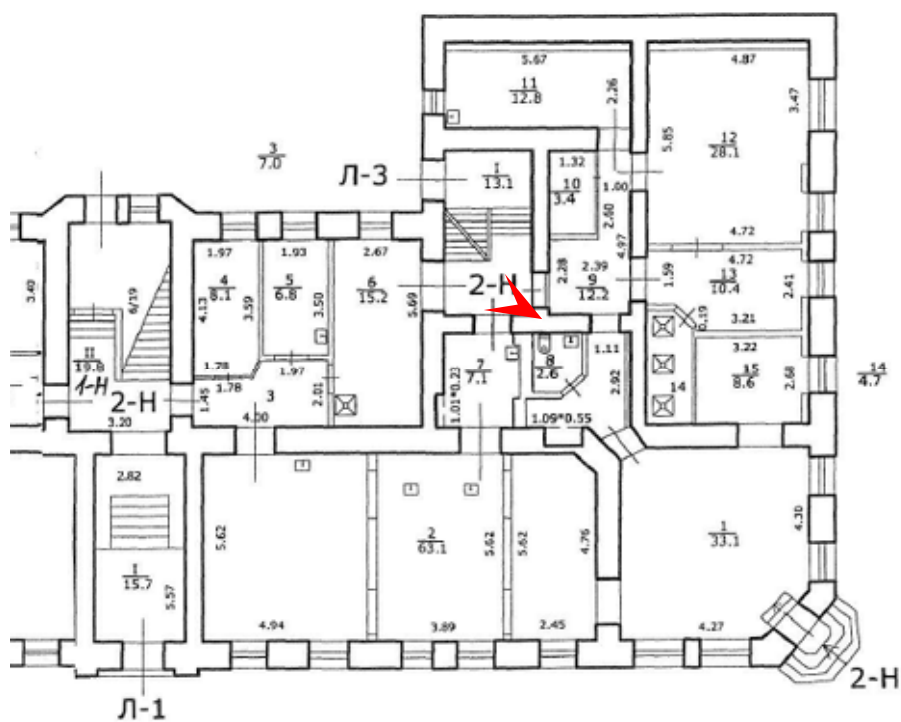
32. Объект культурного наследия регионального значения «Доходный дом Ю.К. Добберт» по адресу: улица Лизы Чайкиной, дом 4/12, литера А Фрагмент плана 1 этажа. Вид на лестницу Дата съемки: 25.05.2026
