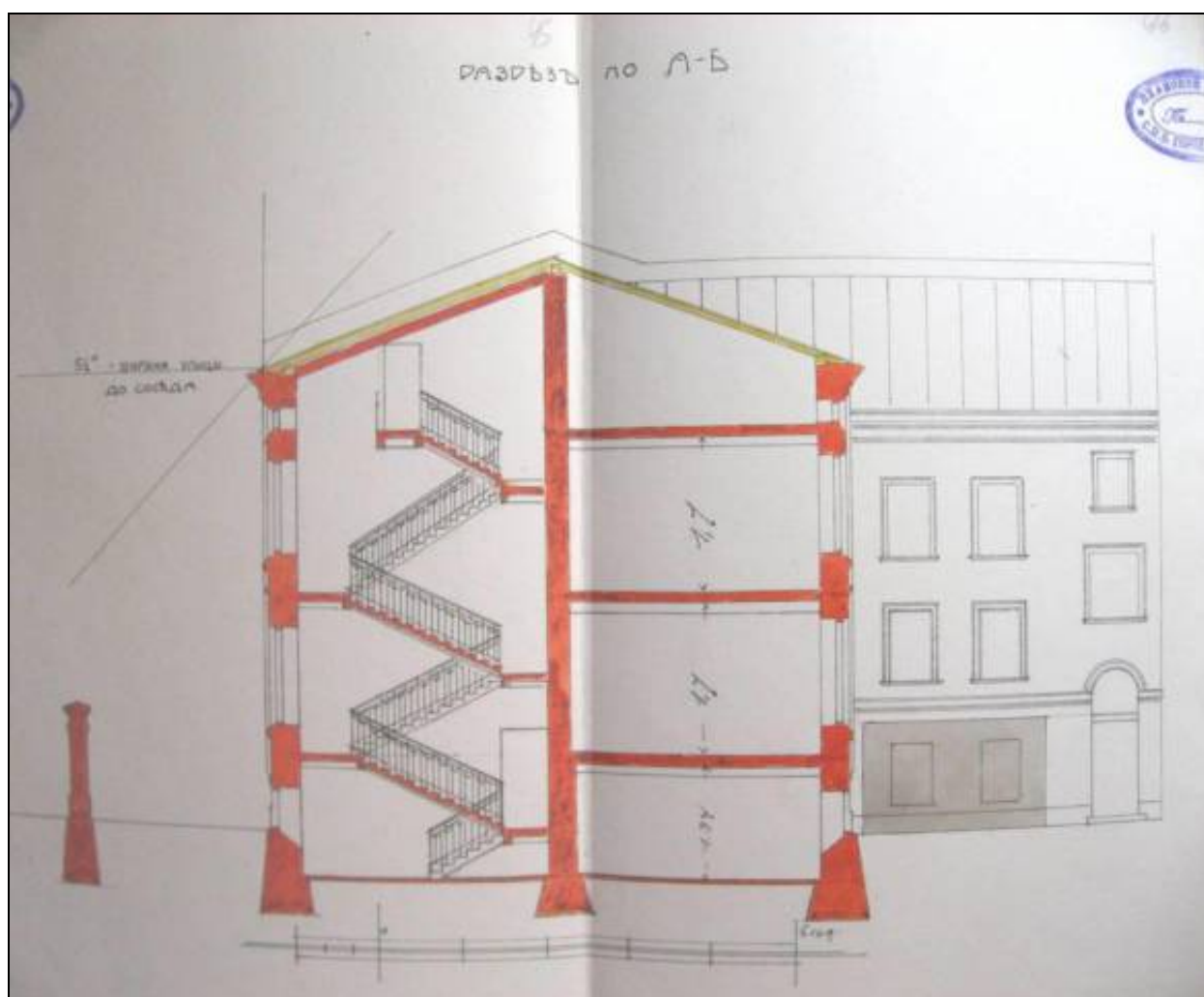
22. Разрез фабричного флигеля по линии А-В на участке № 22. 1913 г. ЦГИА СПб.
