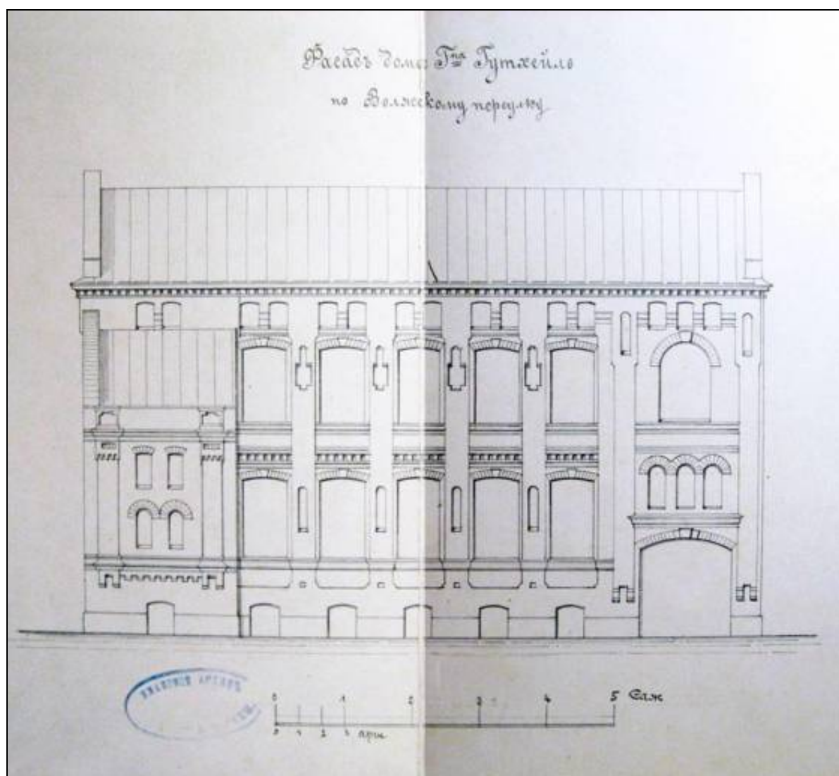
13. Фасад фабричного флигеля по Волжскому переулку. 1890 г. ЦГИА СПб.
