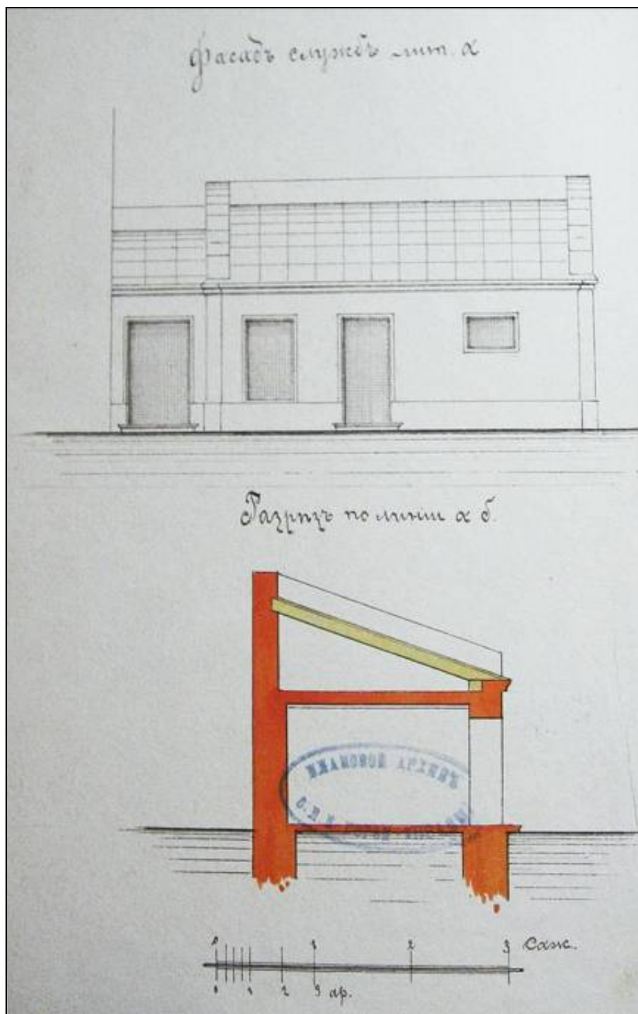
17. Фасад и разрез одноэтажных служб Лит Л. 1890 г. ЦИИА СПб.
