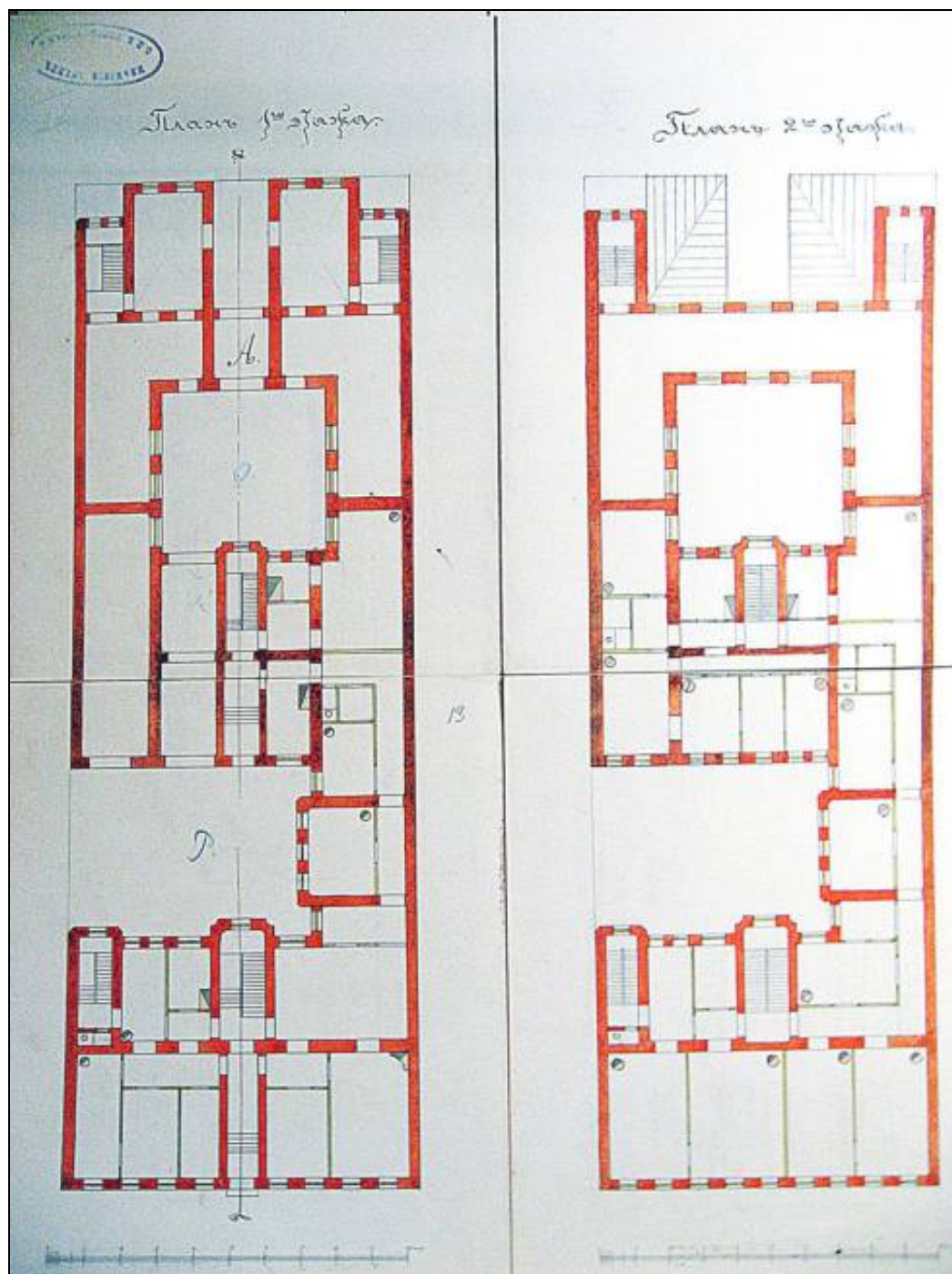
9. Поэтажные планы строений на участке Ф.А. Гутхейля. Планы 1, 2 этажей. 1889 г. ЦГИА СПб.
