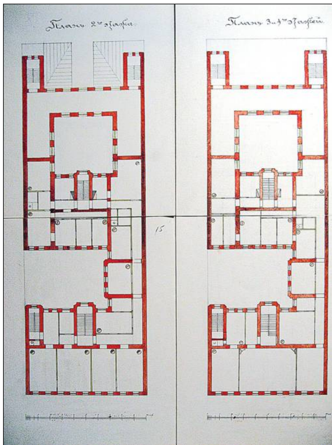
10. Поэтажные планы строений на участке Ф.А. Гутхейля. Планы 3 и 4 этажей. 1889 г. ЦГИА СПб.
