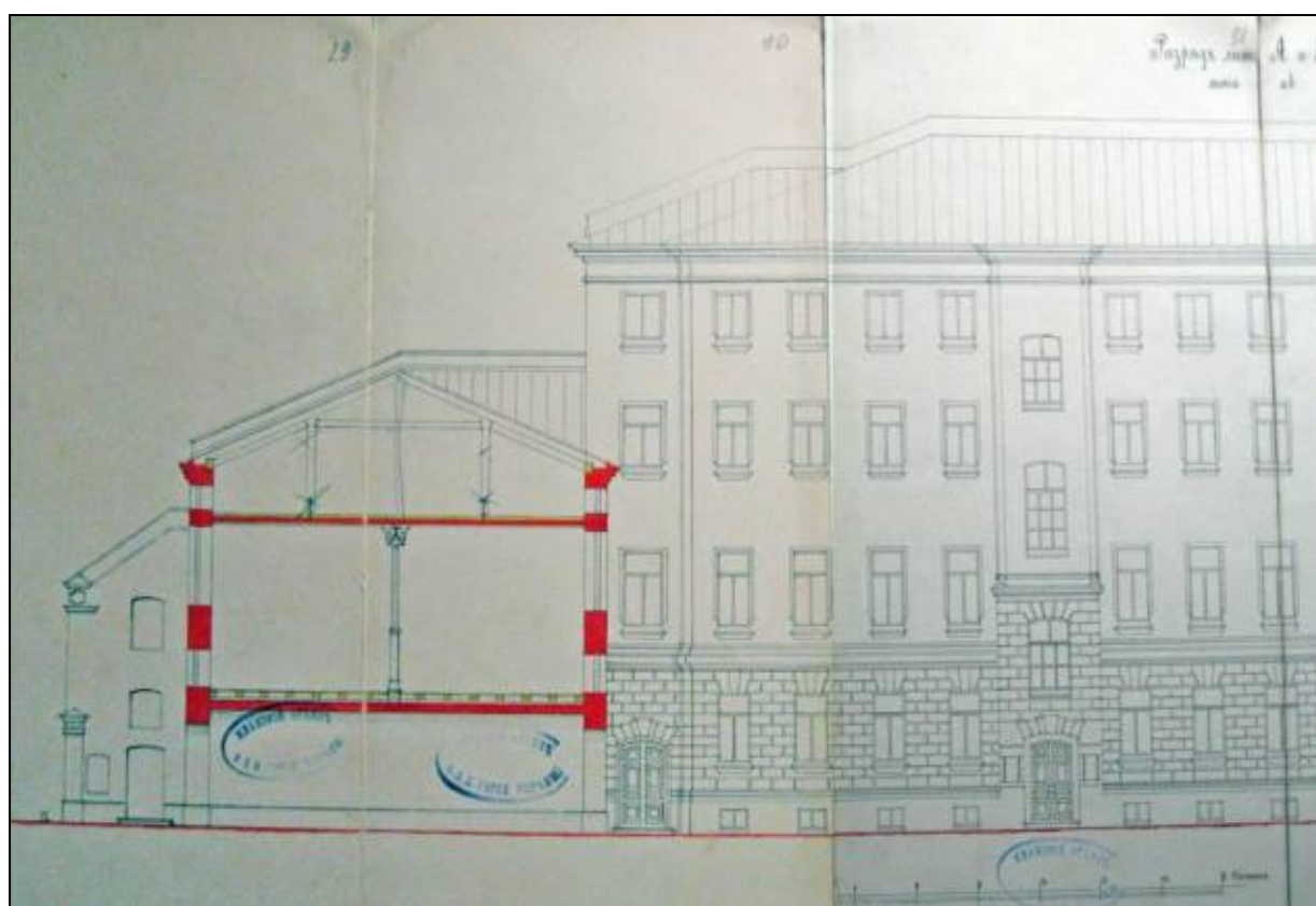
16. Разрез фабричного флигеля и дома Ф.А. Гутхейля по линии аб. 1890 г. ЦГИА СПб.
