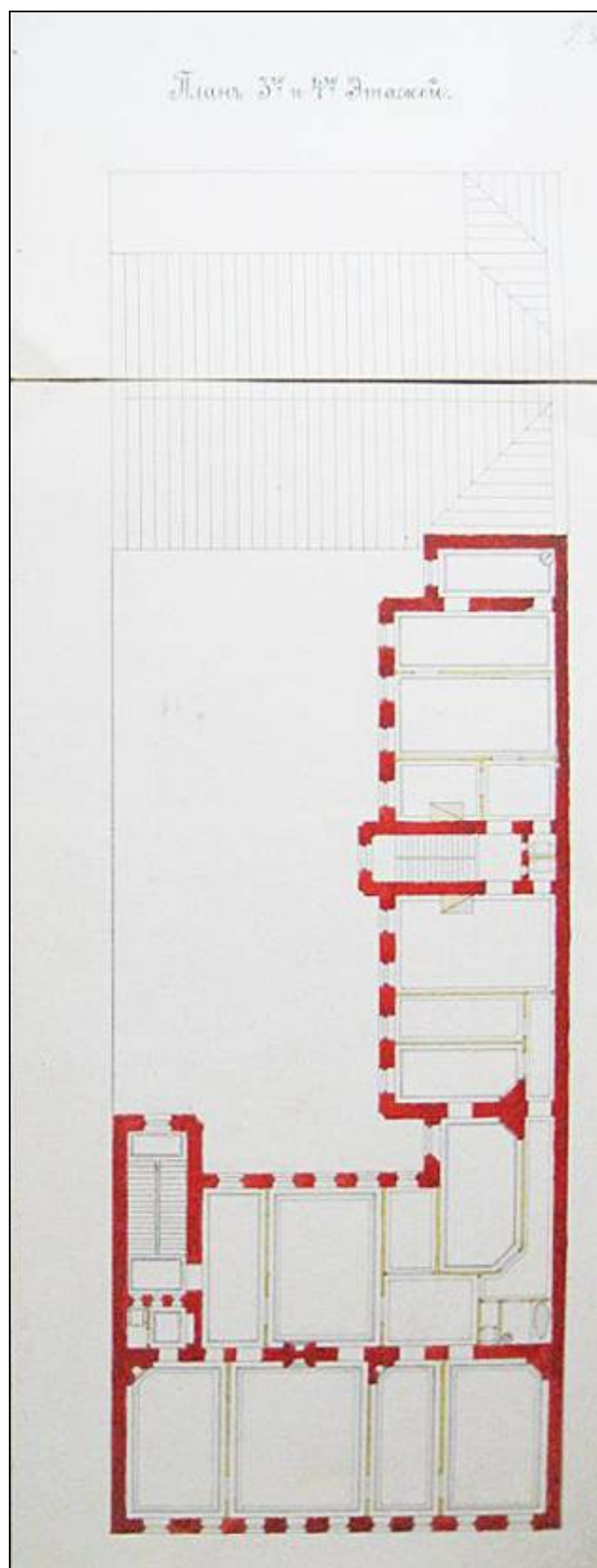
15 Поэтажный план строений 3, 4 этажей на участке Ф.А. Гутхейля. 1890 г. ЦГИА СПб.
