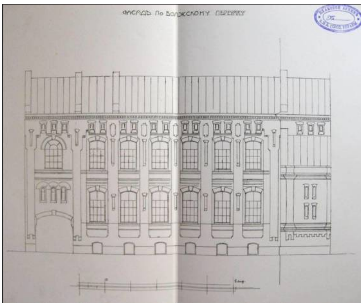
19. Фасад симметричного фабричного флигеля по Волжскому переулку на соседнем участке № 22. 1913 г. ЦГИА СПб.
