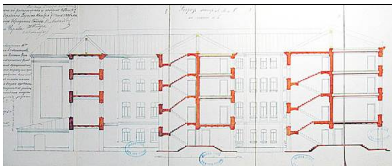
8. Разрез фасада лицевого здания по 5 линии Лит С и флигелей Лит А и В по линии аб. 1889 г. ЦГИА СПб.
