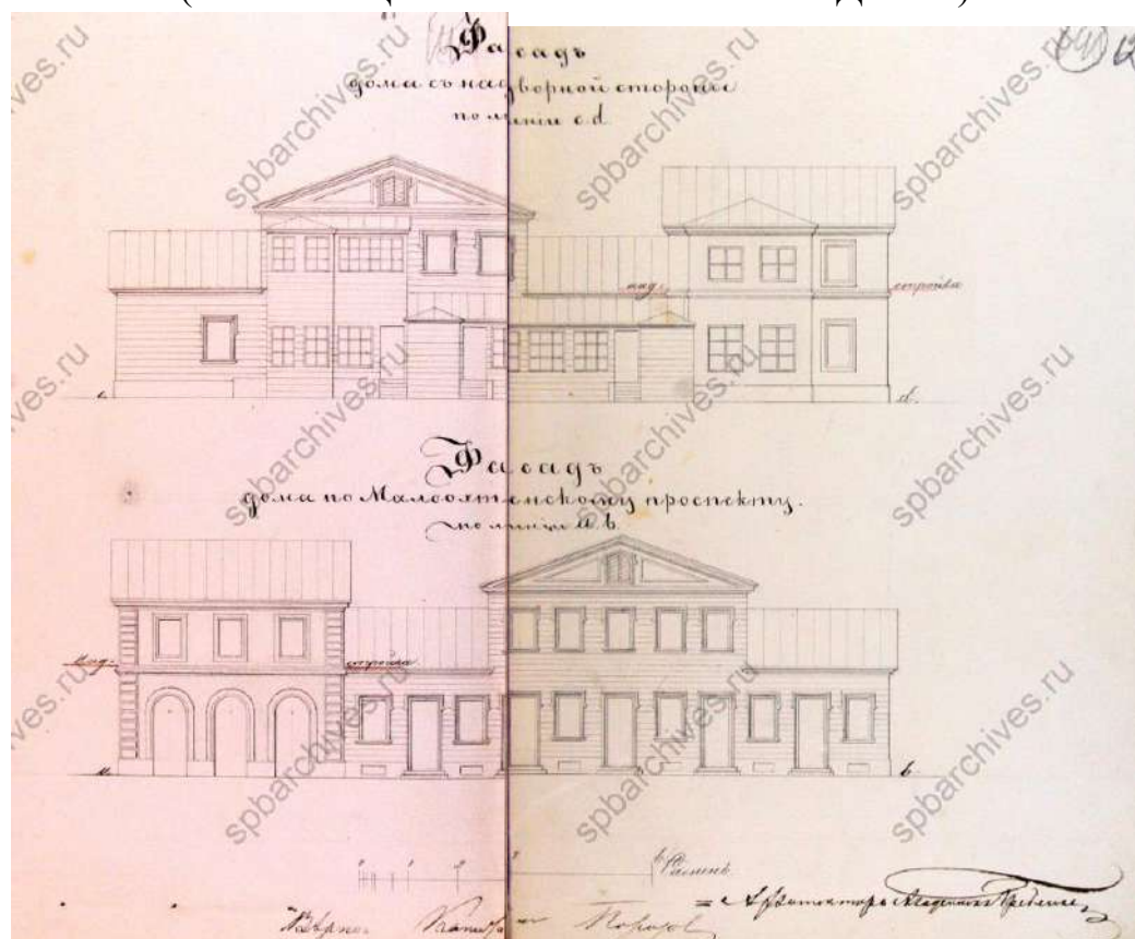
Илл. 11. Фасады дома с надворной стороны и по Малоохтенскому проспекту. 1855 г. (источник: ЦГИА СПб. Ф. 513. Оп. 102. Д. 9154).
