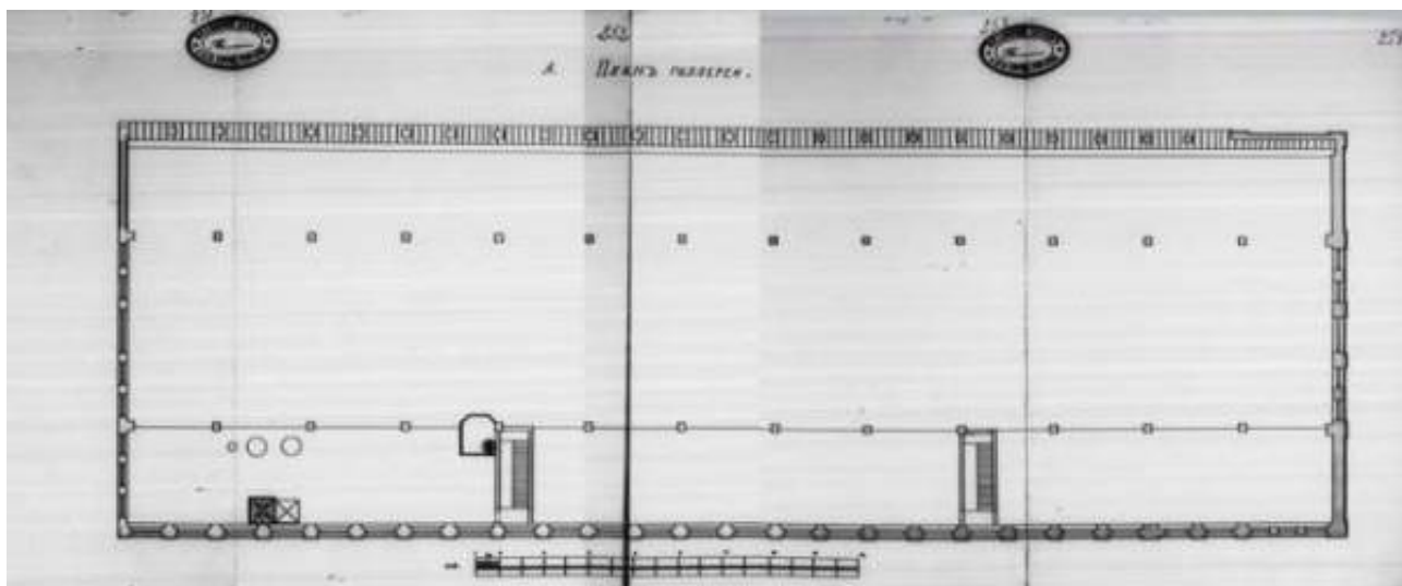
Илл. 31. Проект чугунолитейного цеха. План галереи. Инж.-механик Г.Ф. Джонсон. 1913 г. ЦГИА СПб Ф. 513. Оп. 102. Д. 2859. Л. 251-254.
