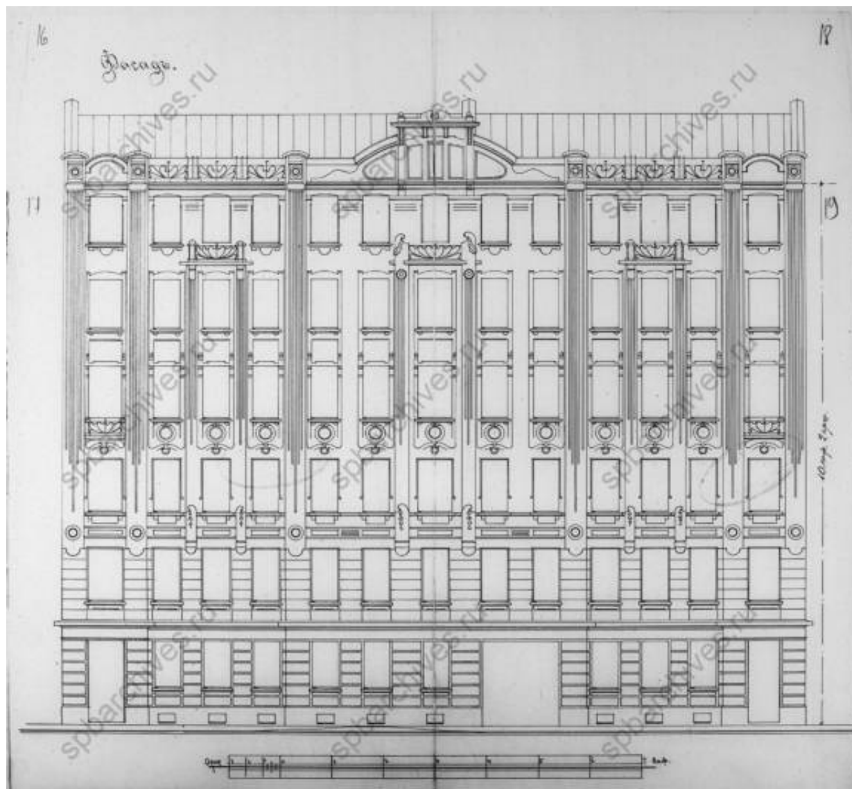
11. Фасад. 1906 г. // Источник: ЦГИА СПб Ф.513 Оп.102 Д.9372 Лл.16-19.
