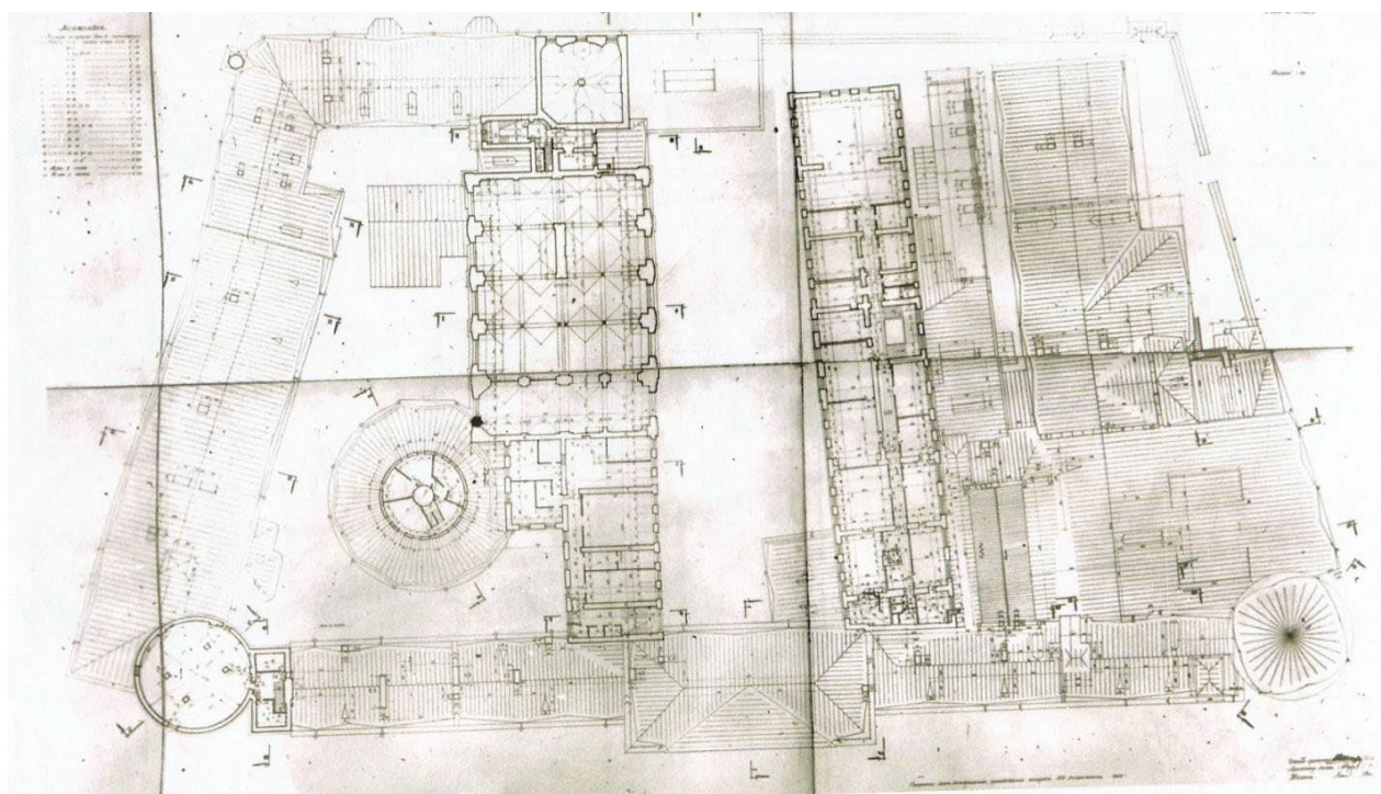
26. Монетный двор. Обмерный чертеж плана 3 этажа. 1964 г. Архив КГИОП.
