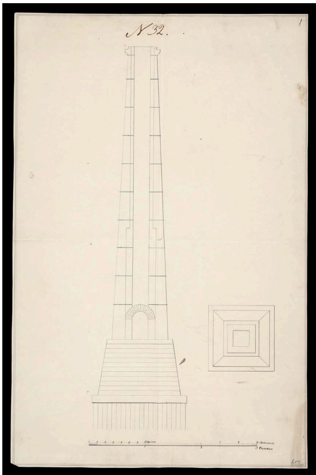
37. Монетный двор. Чертеж трубы от двух паровых котлов. 1844? РГИА.Ф.570. РГИА. Ф.570. Оп.14. Д.201.Л.1.
