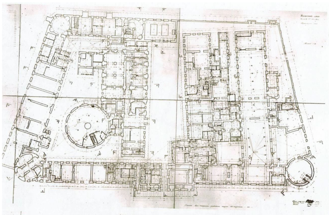
24. Монетный двор. Обмерный чертеж плана 1 этажа. 1964 г. Архив КГИОП.
