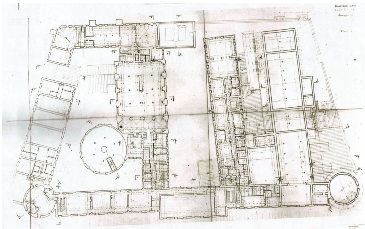
25. Монетный двор. Обмерный чертеж плана 2 этажа. 1964 г. Архив КГИОП.
