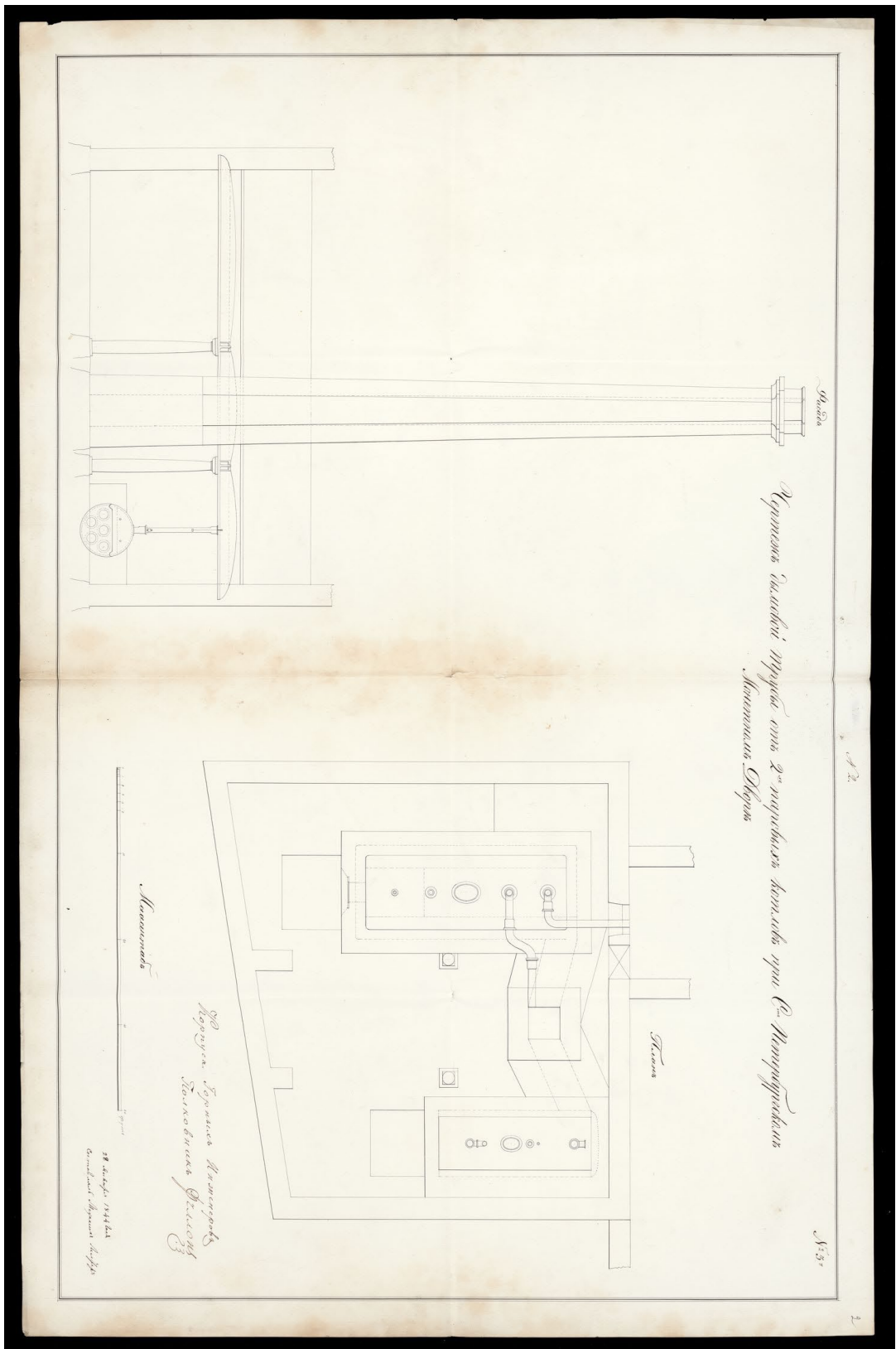
38. Монетный двор. Чертеж трубы от двух паровых котлов. 1844. РГИА.Ф.570. РГИА. Ф.570. Оп.14. Д.201.Л.2.
