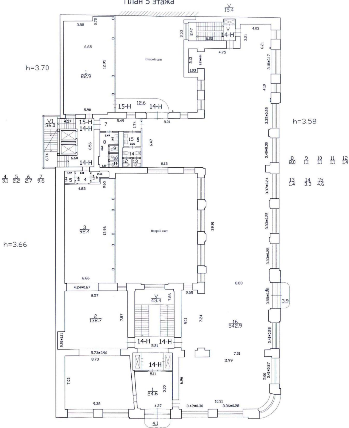
План 5 этажа
