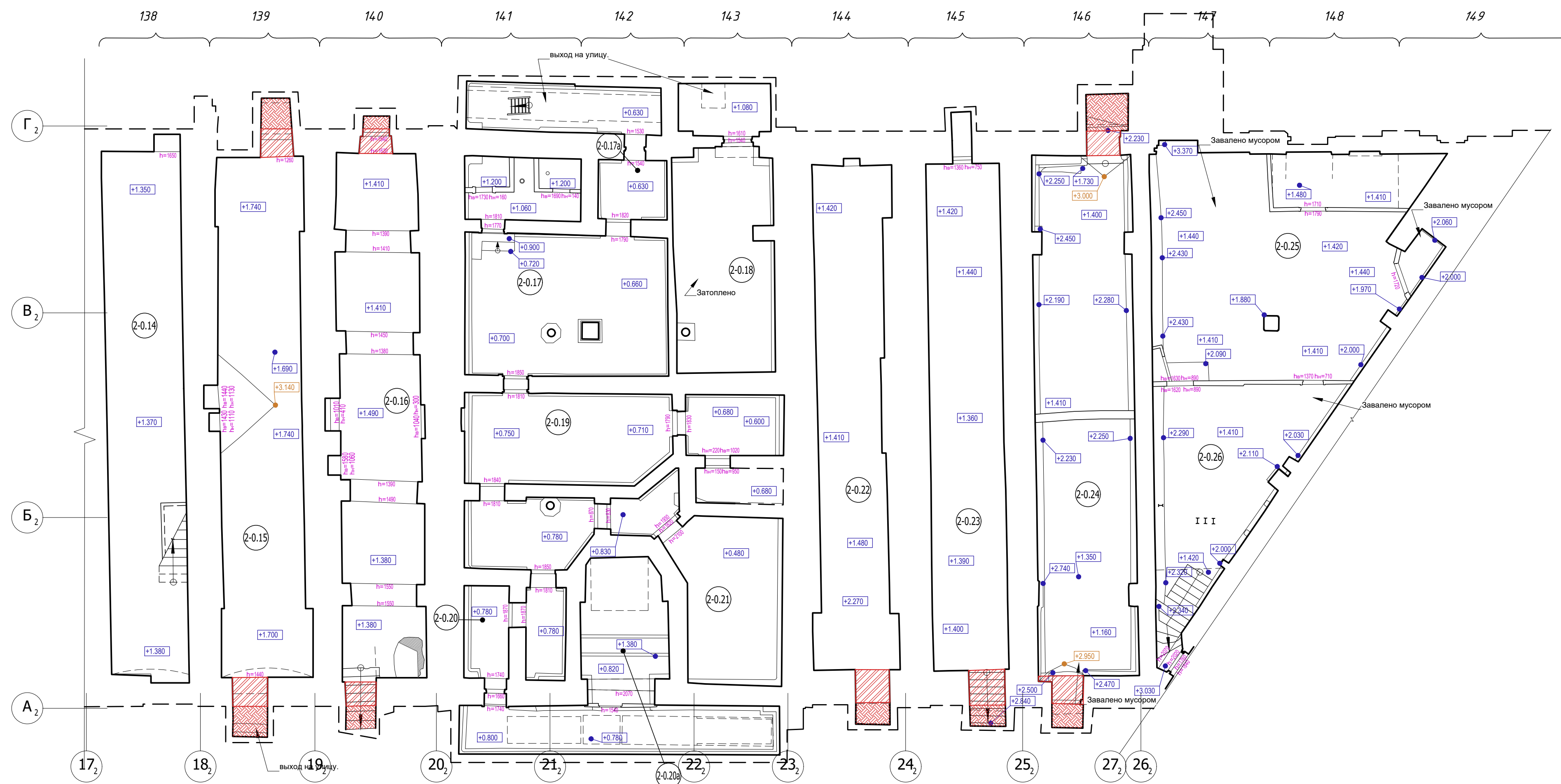
План подвала участка в осях 18 2 -27 2
