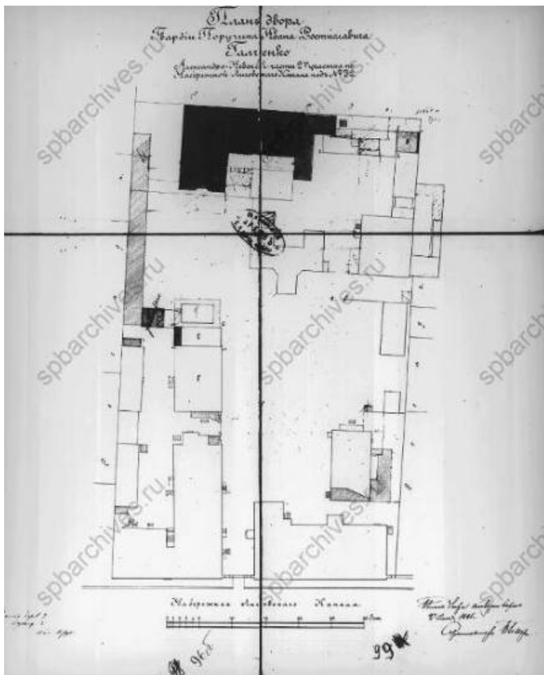
Илл. 7. План двора гвардии поручика И.Р. Галченкова. Александр-Невской части, 2-го участка, по набережной Лиговского канала под № 32. 1875 г. ЦГИА СПб. Ф. 513. Оп. 102. Д. 524. Л. 96об.- 99.
