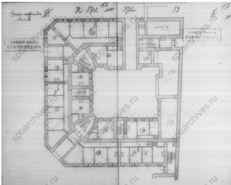
Илл. 18. План подвалов флигеля под Лит. В. Комплект чертежей владения, заверенный архитектором Кредитного общества в 1912 г. ЦГИА СПб. Ф. 515. Оп. 4. Д. 2502. Л. 156, 157.
