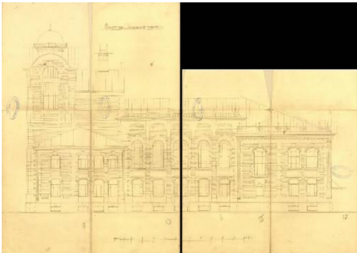
Илл. 25. Фасад по Прилукской улице, предполагаемого к постройки каменного двухэтажного лицевого дома, показанного на плане двора под лит. А. 1901 г. // ЦГИА СПб. Фонд 513. Опись 102. Дело 1004.
