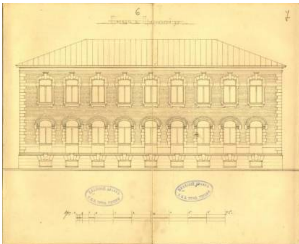
Илл. 13. Фасад по Прилукской улице, предполагаемого к постройки каменного двухэтажного, на нежиле подвале лицевого дома, показанного на плане двора под лит. А. 1901 г. // ЦГИА СПб. Фонд 513. Опись 102. Дело 1004.
