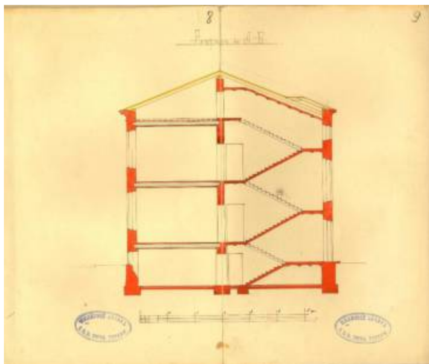
Илл. 12. Разрез по линии А-Б, предполагаемого к постройки каменного двухэтажного, на нежилом подвале лицевого дома, показанного на плане двора под лит. А. 1901 г. // ЦГИА СПб. Фонд 513. Опись 102. Дело 1004.
