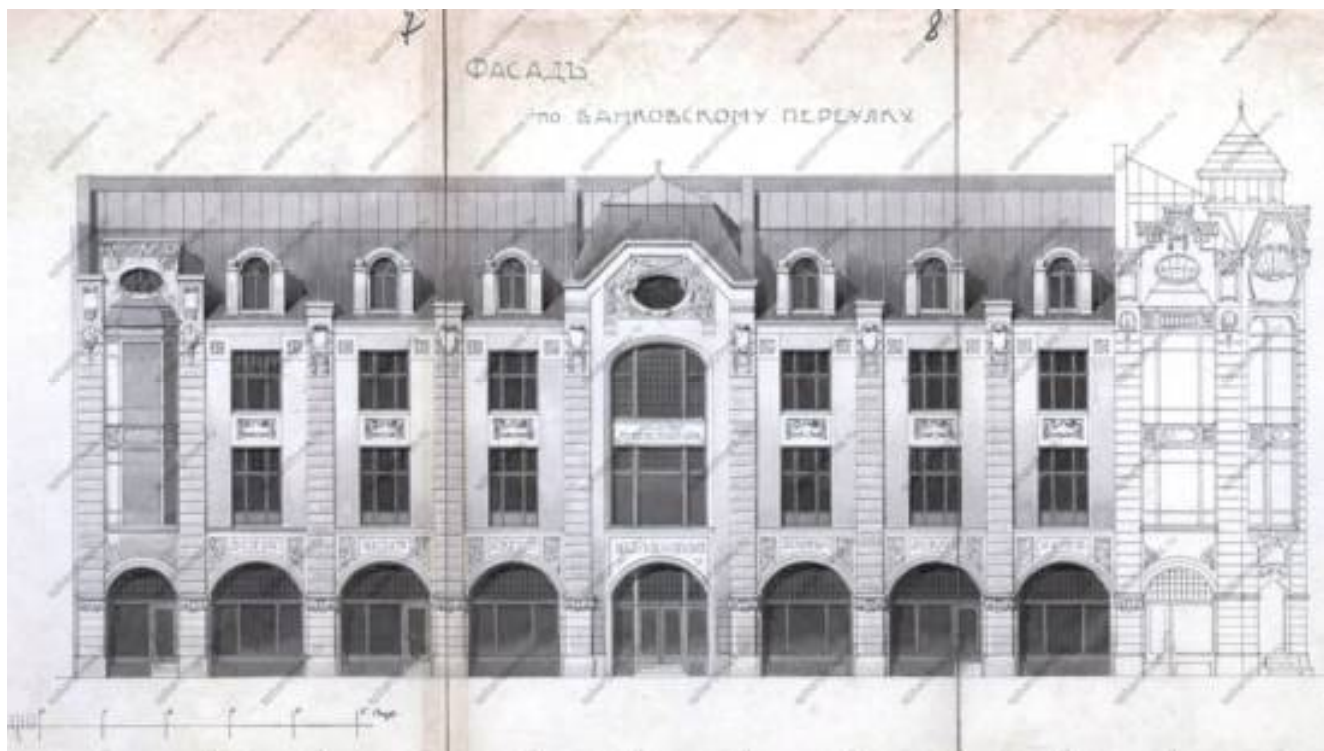
Илл.16. Фасад по Банковскому переулку. 1904 г. арх. Лидваль Ф.И. (неосущ. проект). ЦГИА СПб. Фонд 513. Описание 115. Дело 652. Л.7-9.
