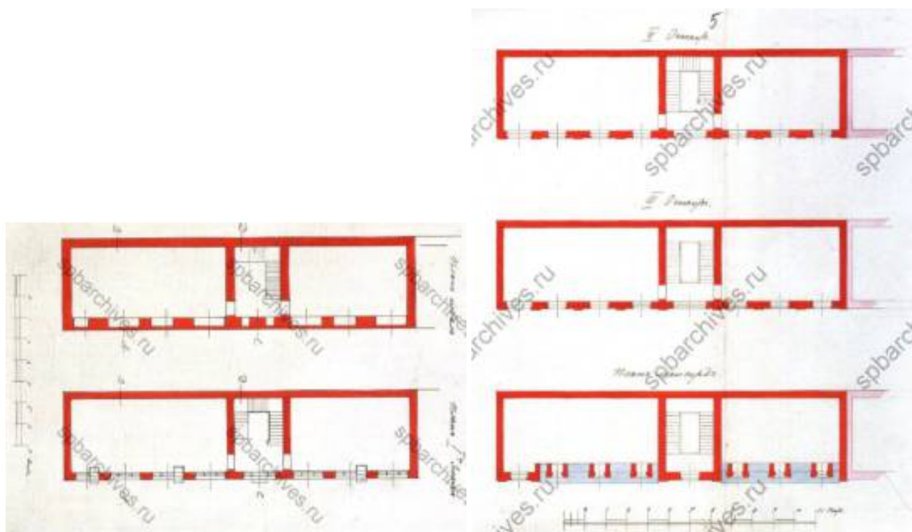
Илл.17. Планы подвала, 1-2-3-го этажей и мансарды. 1904 г. арх. Лидваль Ф.И. (неосущ. проект). ЦГИА СПб. Фонд 513. Описание 115. Дело 652. Л.4-6.
