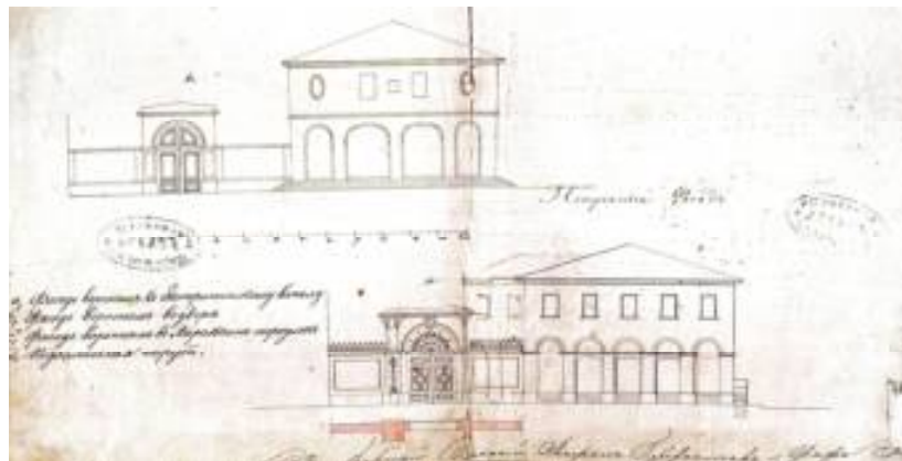
Илл.10. Проект переустройства лавок старого флигеля для торгу железным и мучным товаром. Фасад по Екатерининскому каналу. 1836 г. ЦГИА СПб Ф.513. Оп.115. Д.706. Л.10-11.
