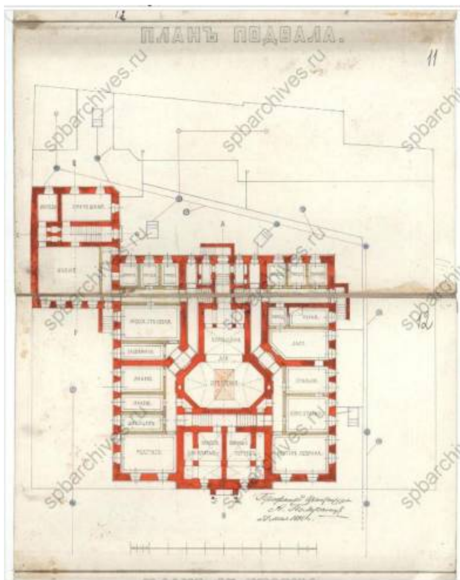
12. Арх. А.Н. Померанцев. Дом-особняк Н.В. Спиридонова на Фурштатской улице, №58. План подвала. 1895 г. ЦГИА СПб. Ф. 513. Оп. 102. Д. 4551. Лл. 11-12.
