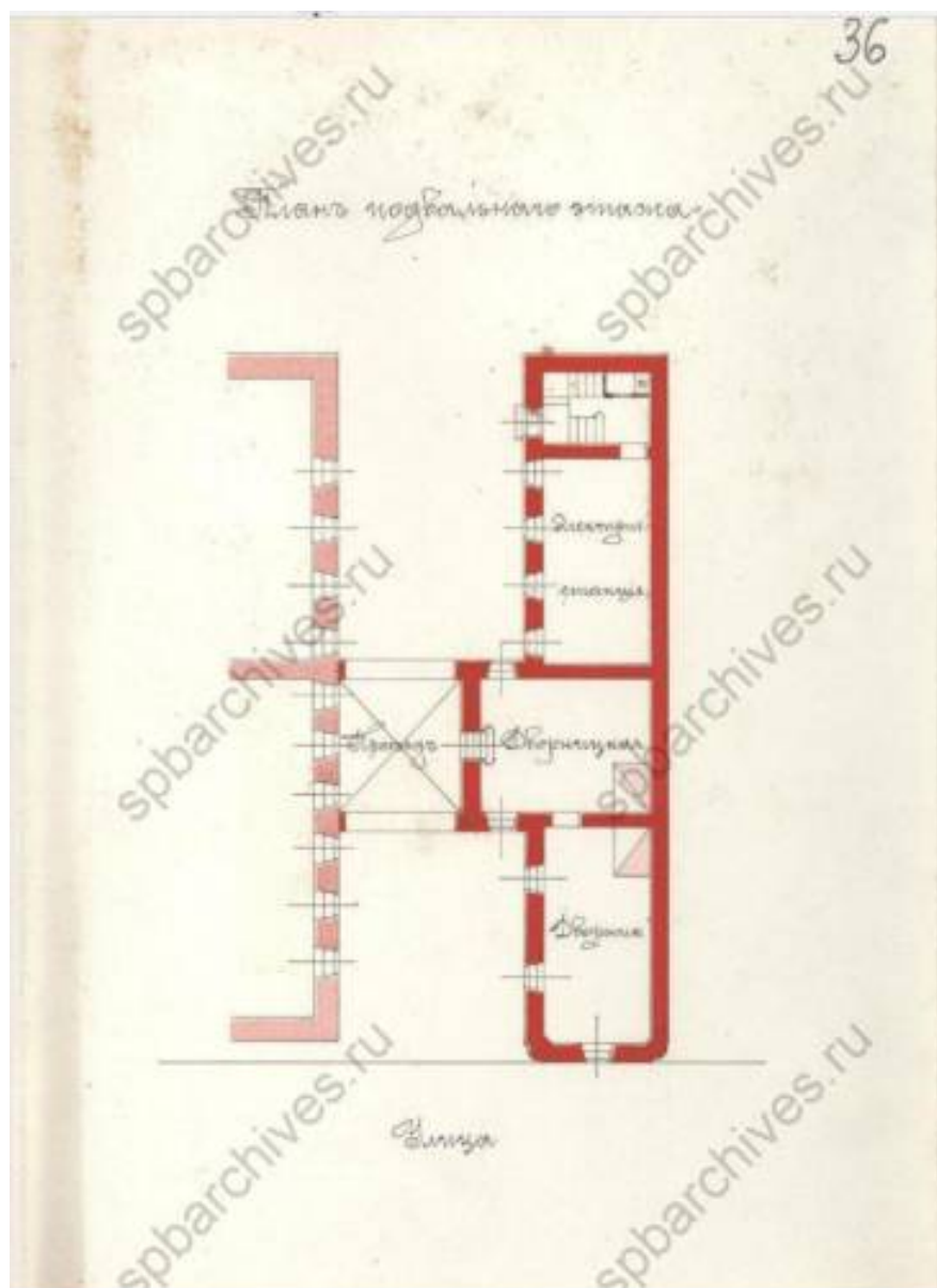
21. Арх. И.С. Китнер. Домовладение Коллежского Советника Н.В. Спиридонова (Фурштатская ул., №58). Службный флигель с зимним садом. План подвального этажа. Проект. 1896 г. ЦГИА СПб. Ф. 513. Оп. 102. Д. 4551. Л. 36.
