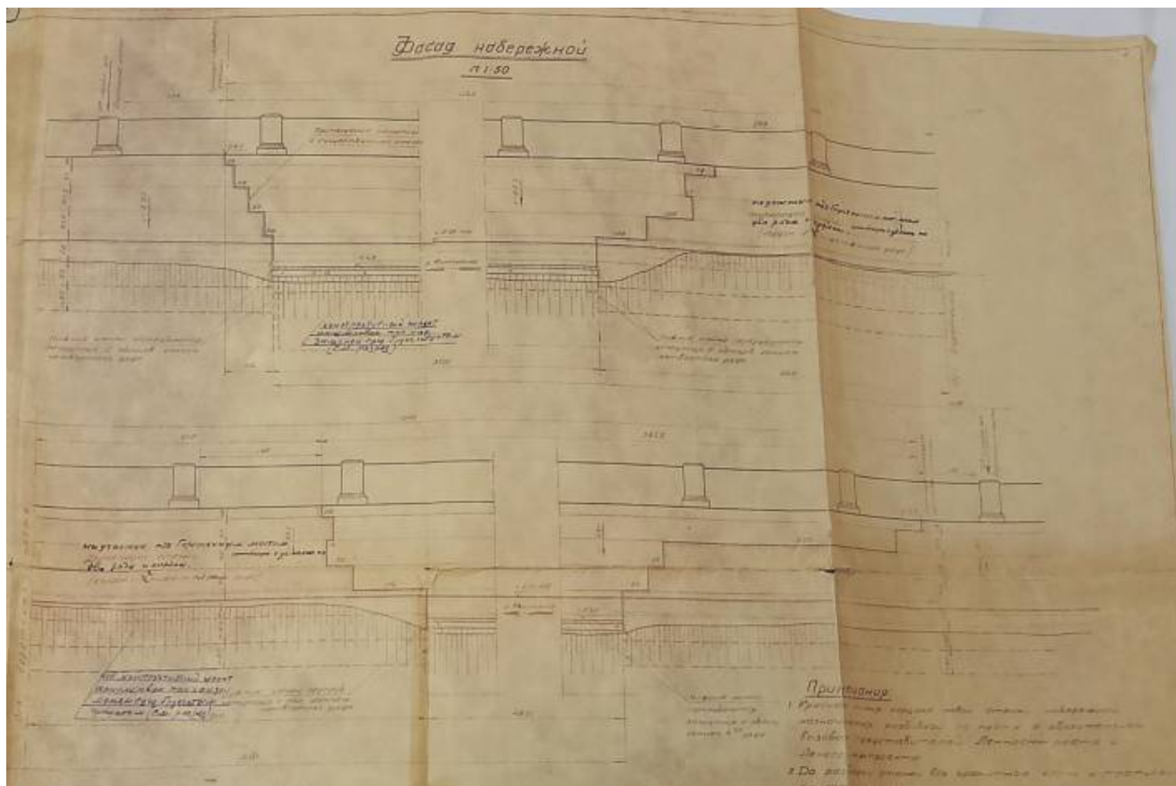
7. Набережная правого берега у д. 91-93. Исполнительный чертеж к проекту капитального ремонта (фрагмент). 1952. Архив Мостотреста. Папка 98/2.
