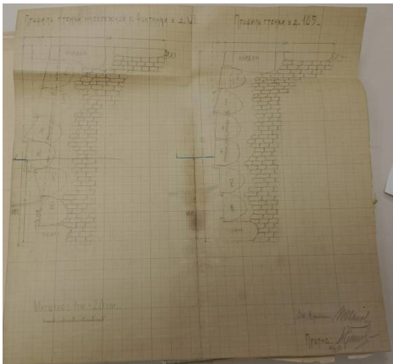
2. Профиль стенки набережной у д. 103 и 109. Архив Мостотреста. Папка 98/5.
