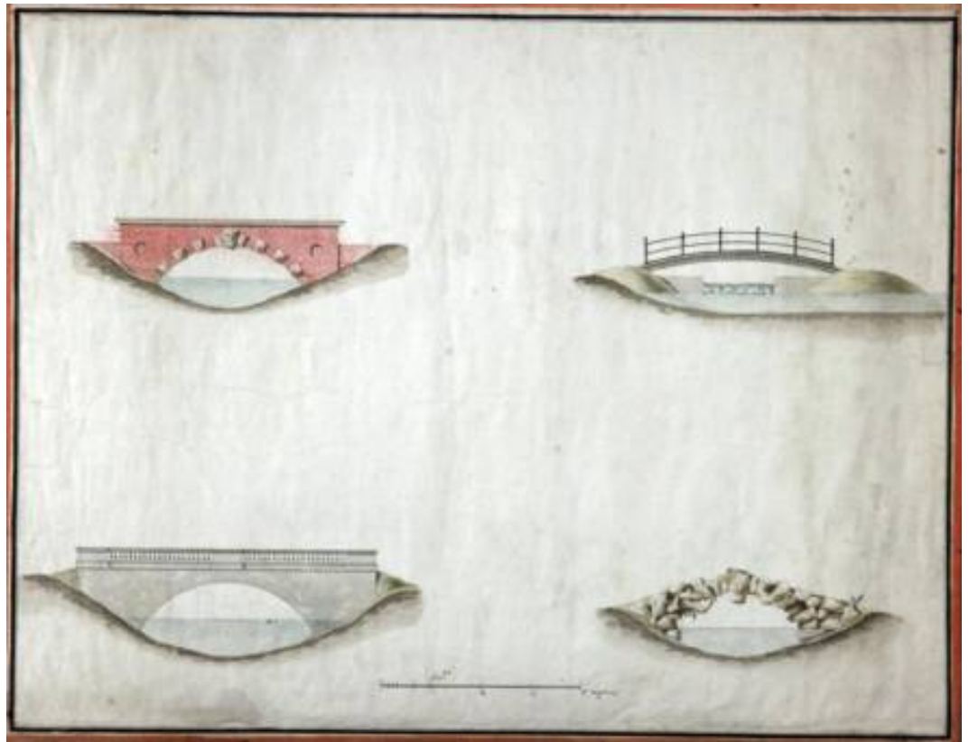
Ил. 5. Четыре моста. Фасады. Фиксационный чертеж. Около 1787 г. На тыльной стороне листа отгиснуто: «4 ponts» («4 моста»), «профили четырем мостам № 70»; на бумажной наклейке надпись: «№ 13 Мосту у Храма Дружбы Листовъ 1» Бумага верже без водяных знаков Тушь, акварель 477 × 619 Масштабная линейка в саженьях («сажени») и аршинах («аршинь»). Номер В. М. Конашевича: «198/К» Инв. № Ч-90 ПМ КП-42656_1. ГМЗ Павловск.
