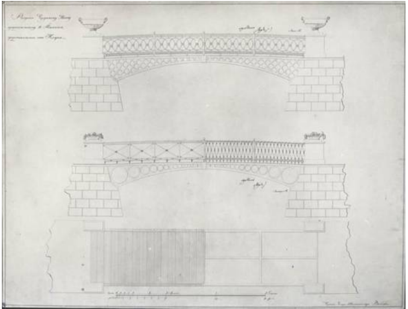
Ил. 15. Проект чугунного моста для Павловского парка. Фасад (три варианта и план). С черт. 596. № ГК:25680351, № КП (ГИК): НИМ РАХ КП-444/41, Инв.№: Ф-11178, ФГБУК НИМ РАХ.
