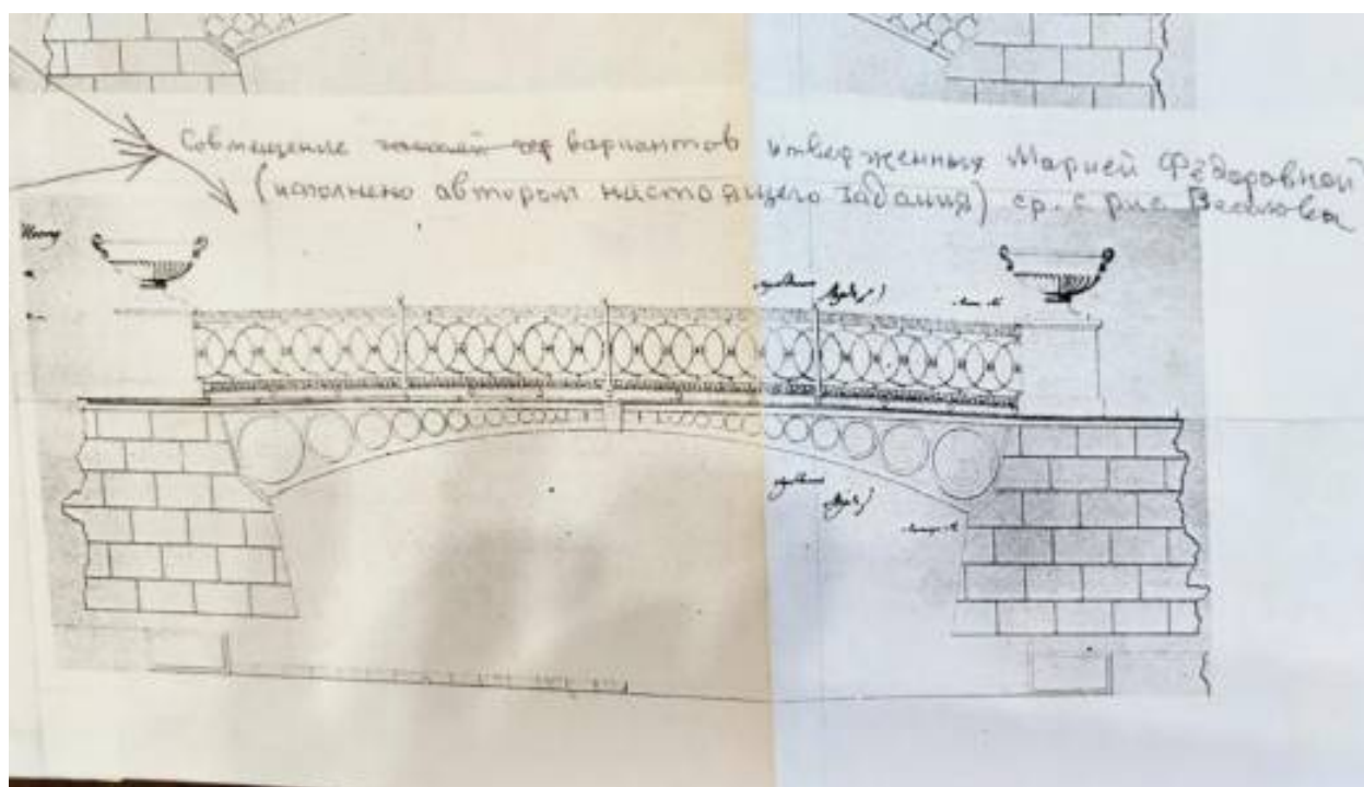
Ил. 16. Совмещение вариантов моста, утвержденных Марией Фёдоровной. Е.В. Королев. Октябрь 2000 г, Плановое задание на реставрацию-реконструкцию Чугунного мостика у Храма дружбы в павловском парке (вместо задания от 20 июня 1990 г.). ГМЗ Павловск.
