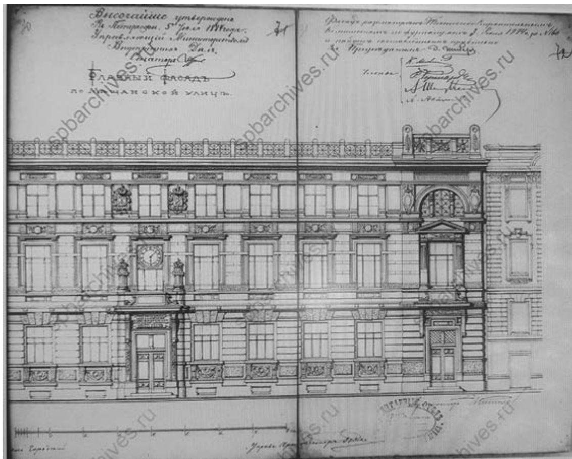
13. Фасад по Мешанкой ул. 1884 г. ЦГИА СПб. Фонд 513. Описание 101. Дело 290.
