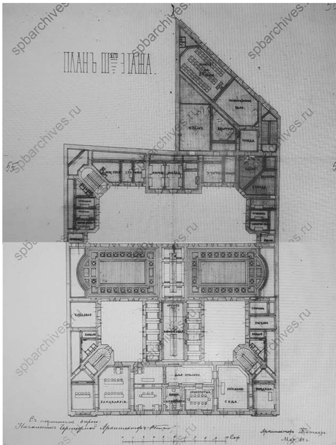
18. План 3-го этажа. ЦГА СПб. Фонд 513. Опись 101. Дело 290.
