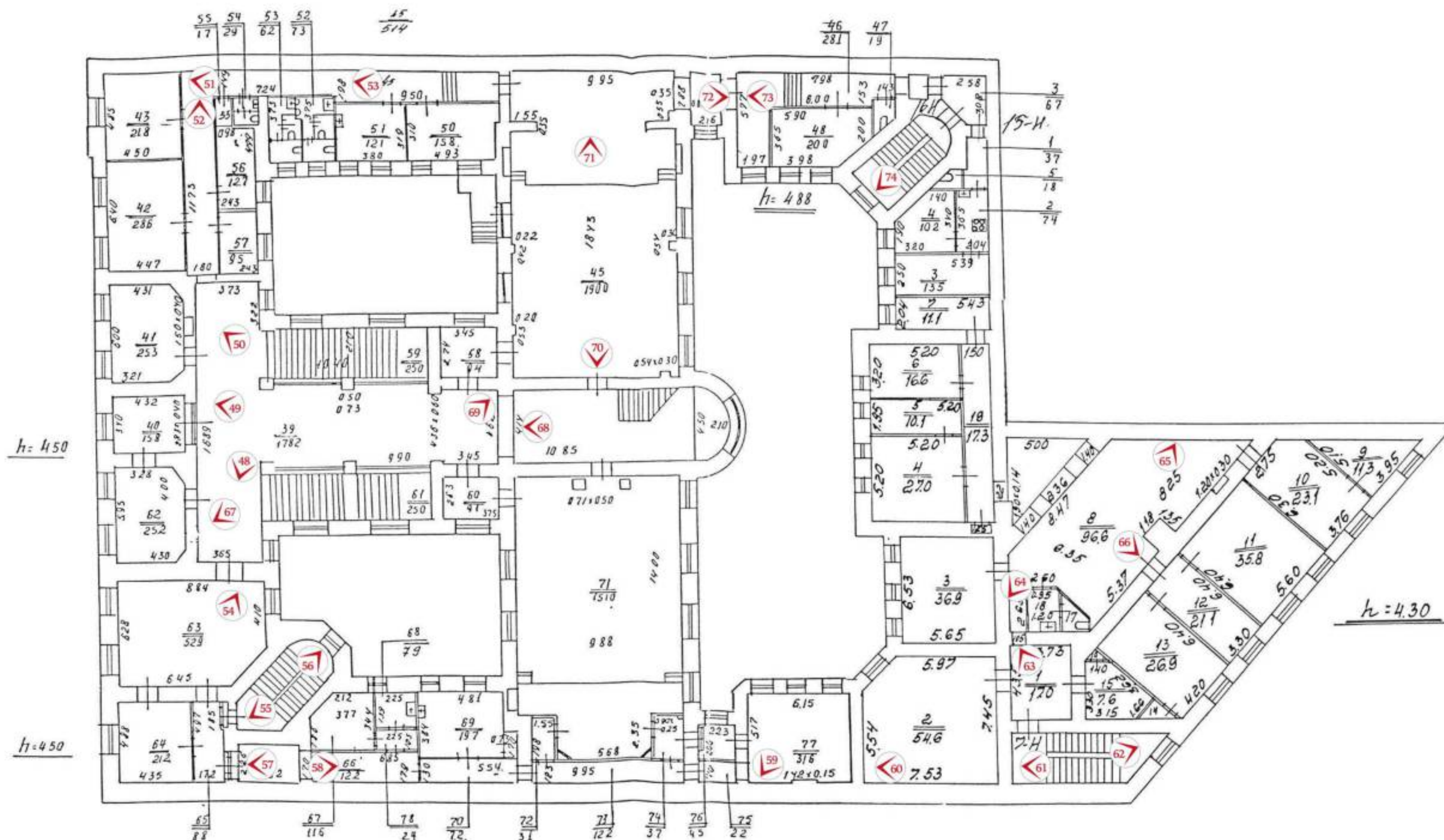
План 2 этажа
