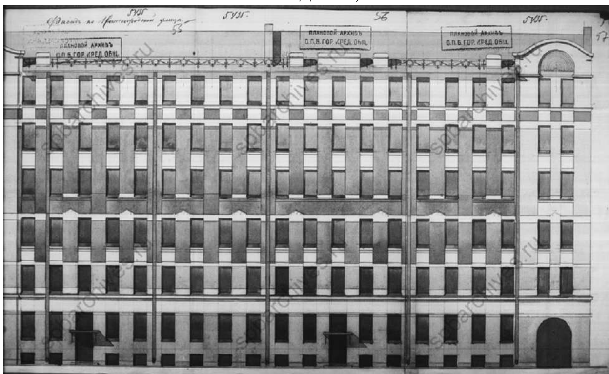
Илл. 18. Фасад по Нижегородской улице. 1904 г. (источник: ЦГИА СПб. Ф. 515. Оп. 4. Д. 3765).
