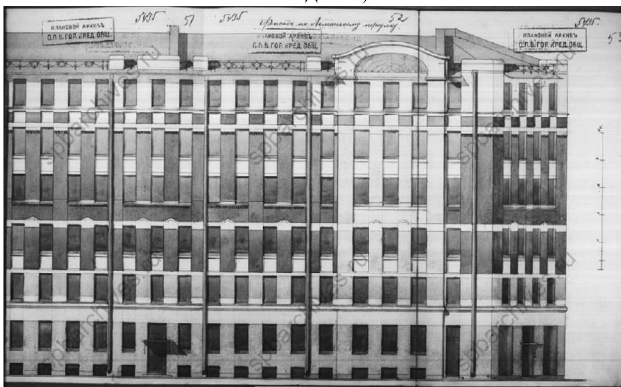
Илл. 16. Фасад по Ломанскому переулку. 1904 г. (источник: ЦГИА СПб. Ф. 515. Оп. 4. Д. 3765).
