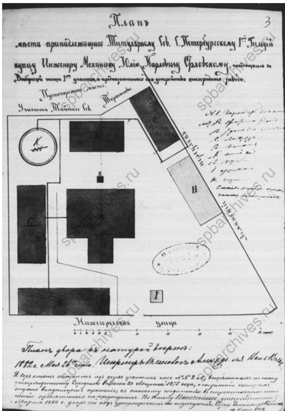
Илл. 8. План места, принадлежащего Титулярному Сов. С.-Петербургскому 1-й гильдии купцу инженеру-механику Юлию Карловичу Орловскому, находящегося в Выборгской части 1-го участка и предназначенного для устройства кислородного завода. 1882 г. (источник: ЦГИА СПб. Ф. 513. Оп. 102. Д. 2749).
