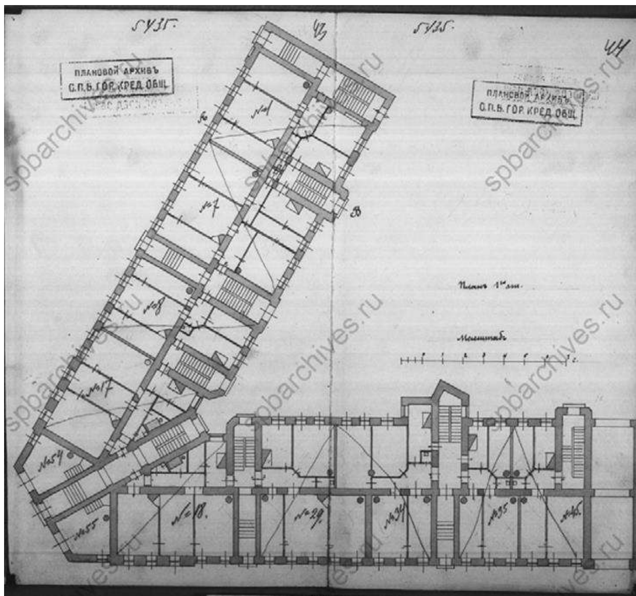
Илл. 14. План 1-го этажа. 1904 г. (источник: ЦГИА СПб. Ф. 515. Оп. 4. Д. 3765).
