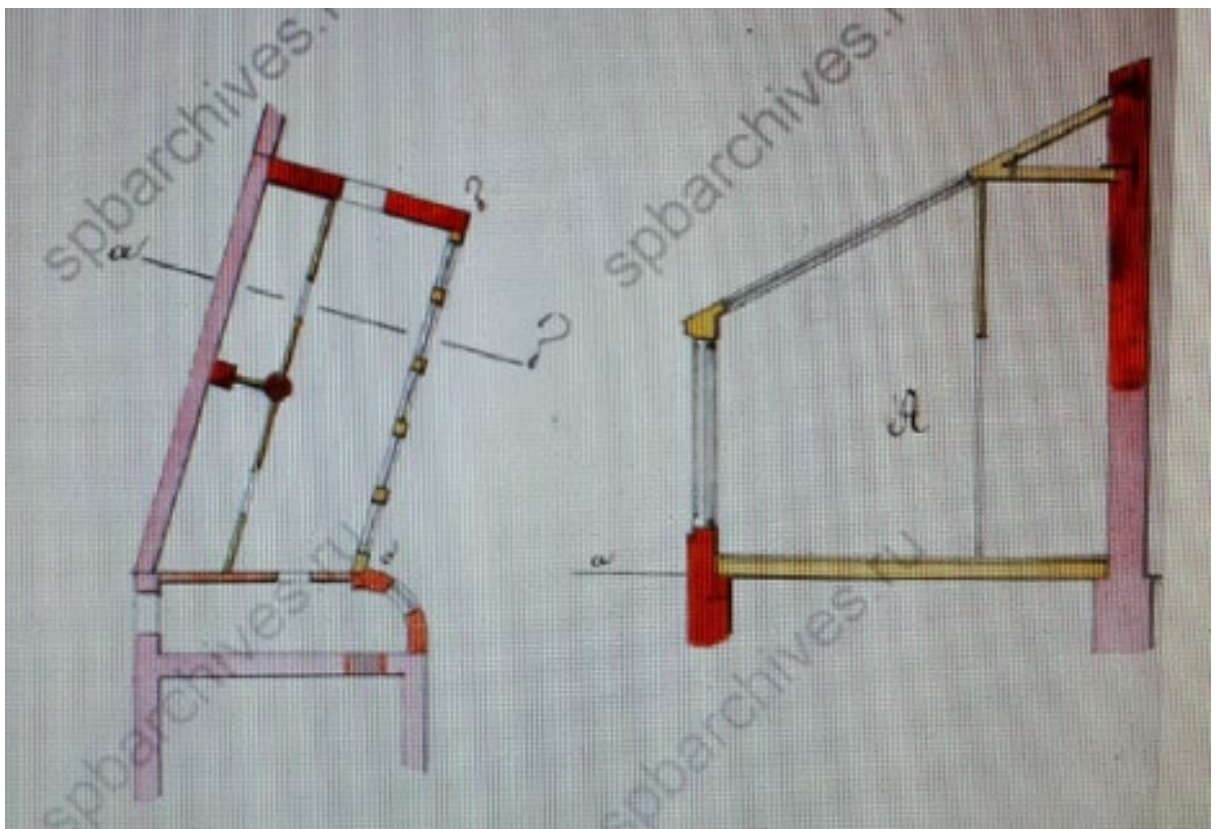
11. План и разрез фотографии. Лит. А. 1879 г. ЦГИА СПб. Ф. 513. Оп. 102. Д. 4501. Л. 86
