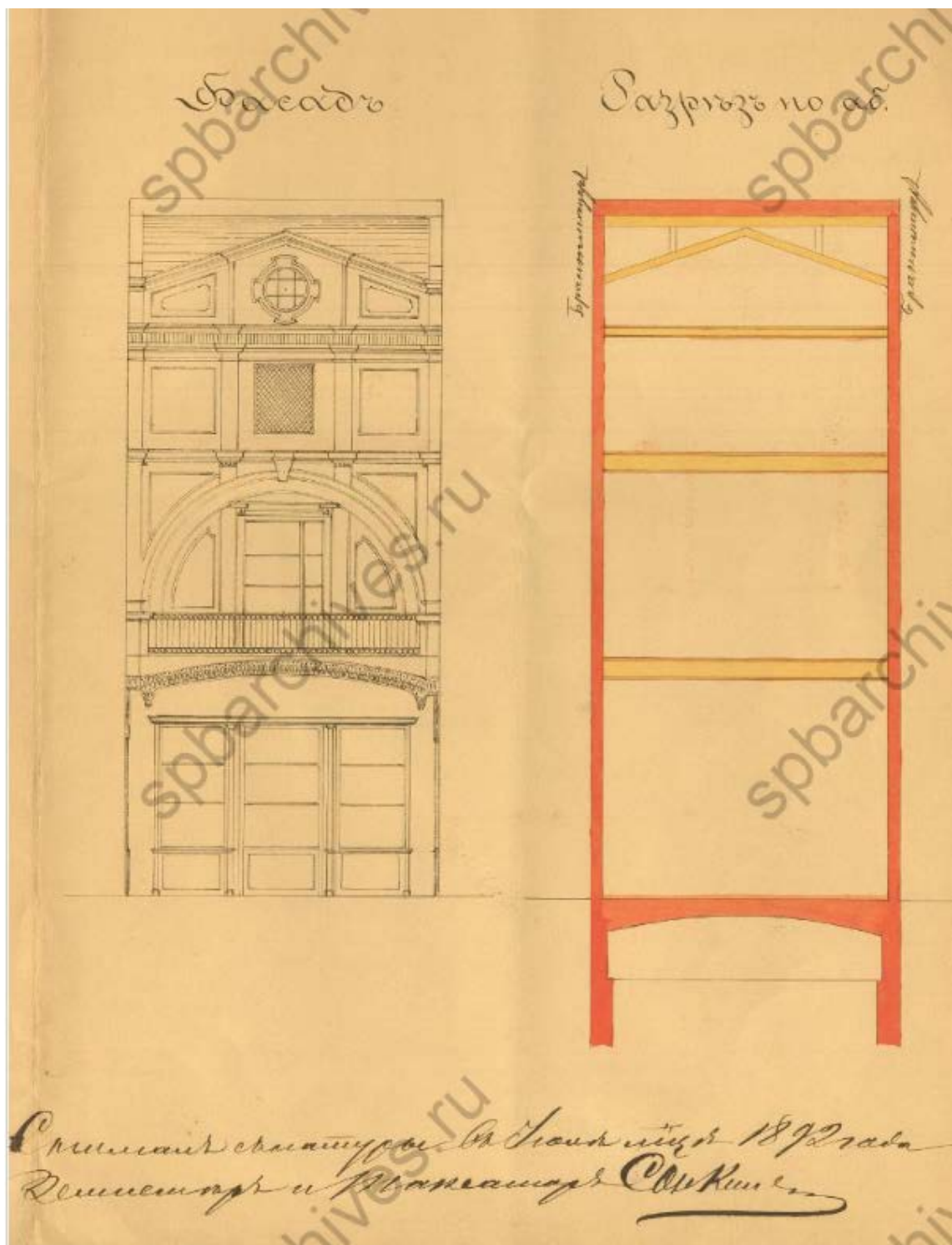
10. Чертежи каменной лавки № 15 С.И. Дойникова по Чернышеву пер. (ул. Ломоносова). Фрагмент фасада и разрез дома по аб. 1892 г. — ЦГИА СПб. Ф. 515. Оп. 4. Д. 5791.
