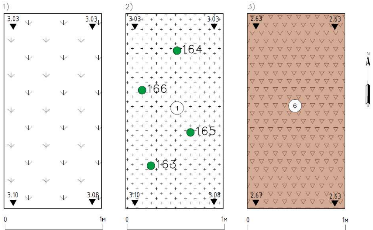
Рис. 50. ОАН «Участок культурного слоя Санкт-Петербурга XVIII –начала XIX в., по адресу: Санкт-Петербург, 14-я линия В.О., дом 57-61». Шурф №2. Чертежи. План 1)дневной поверхности, 2)верха пачки слоев коричневой и светло-коричневой мешаной супеси, 3)верха серо-коричневой супеси со строительным мусором XVIII в. (культурный слой).
