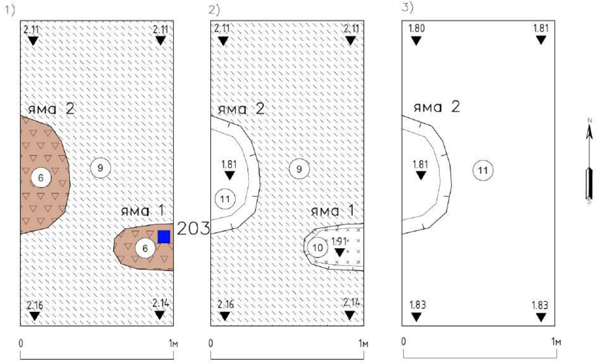
Рис. 51. ОАН «Участок культурного слоя Санкт-Петербурга XVIII –начала XIX в., по адресу: Санкт-Петербург, 14-я линия В.О., дом 57-61». Шурф №2. Чертежи. План 1)верха серо-желтой мешаной супеси, 2)верха серо-желтой мешаной супеси с выбранными ямами, 3)материковой поверхности.
