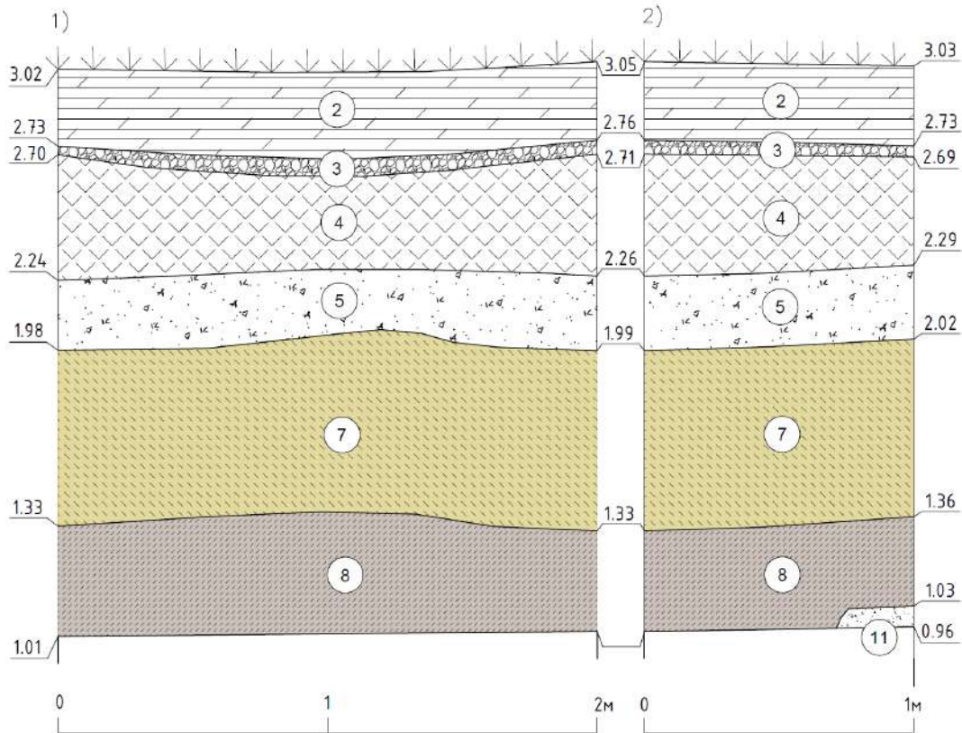
Рис. 79. ОАН «Участок культурного слоя Санкт-Петербурга XVIII –начала XIX в., по адресу: Санкт-Петербург, 14-я линия В.О., дом 57-61». Шурф №3. Чертежи. Стратиграфия 1)южного, 2)западного бортов.
