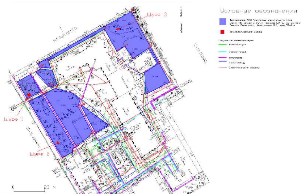
Рис.1. Топографический план ВОАН «Участок культурного слоя Санкт-Петербурга XVIII – начала XIX в., по адресу: Санкт-Петербург, 14-я линия В.О., дом 57-61» с указанием местоположения шурфов. Масштаб 1:500
