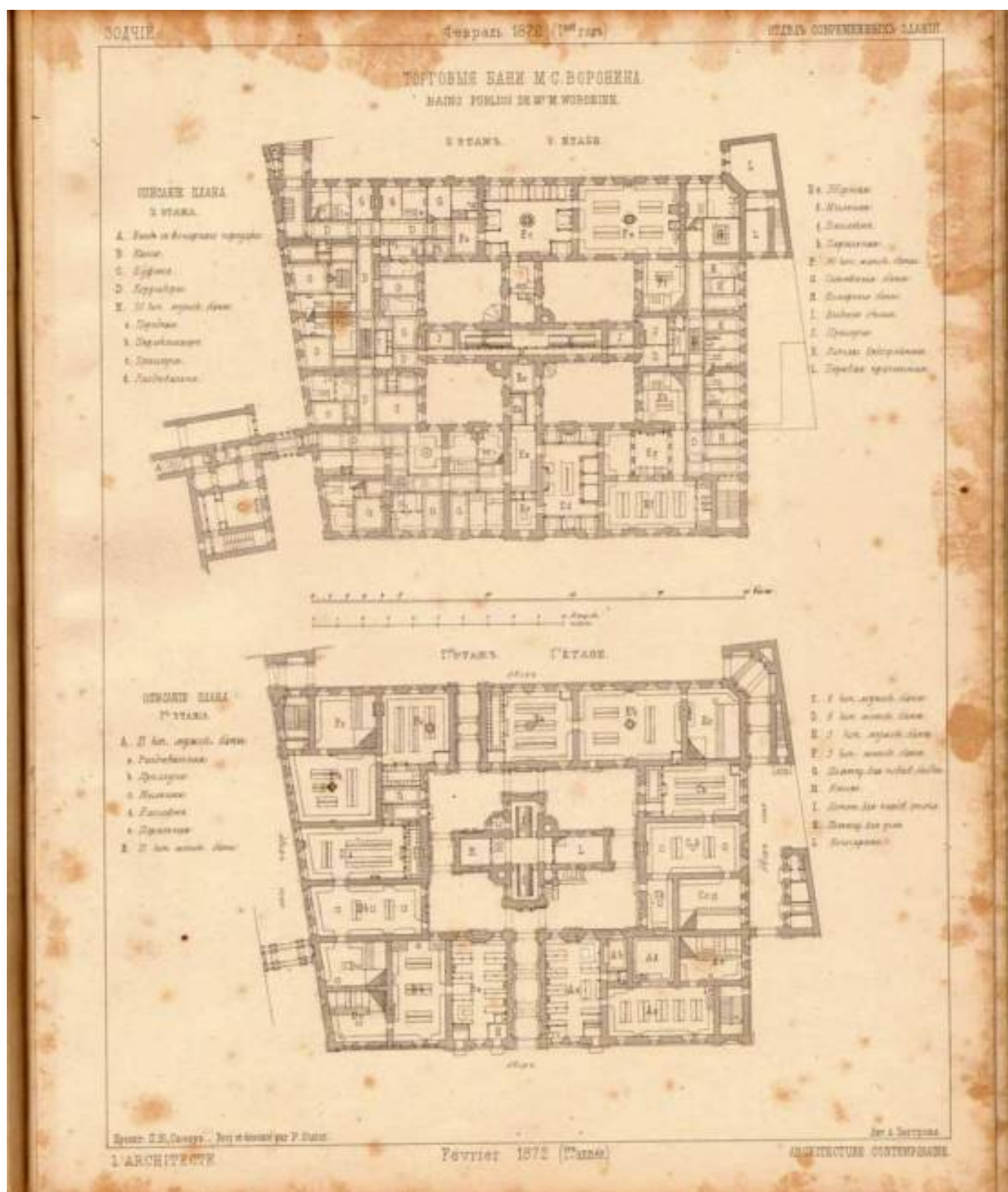
Илл. № 22. 1872 г. Торговые бани М.С. Воронина. План 1-го и 2-го этажей. Зодчий, 1872, №2: Журн., изд. С.-Петербург. о-вом архитекторов. – СПб.
