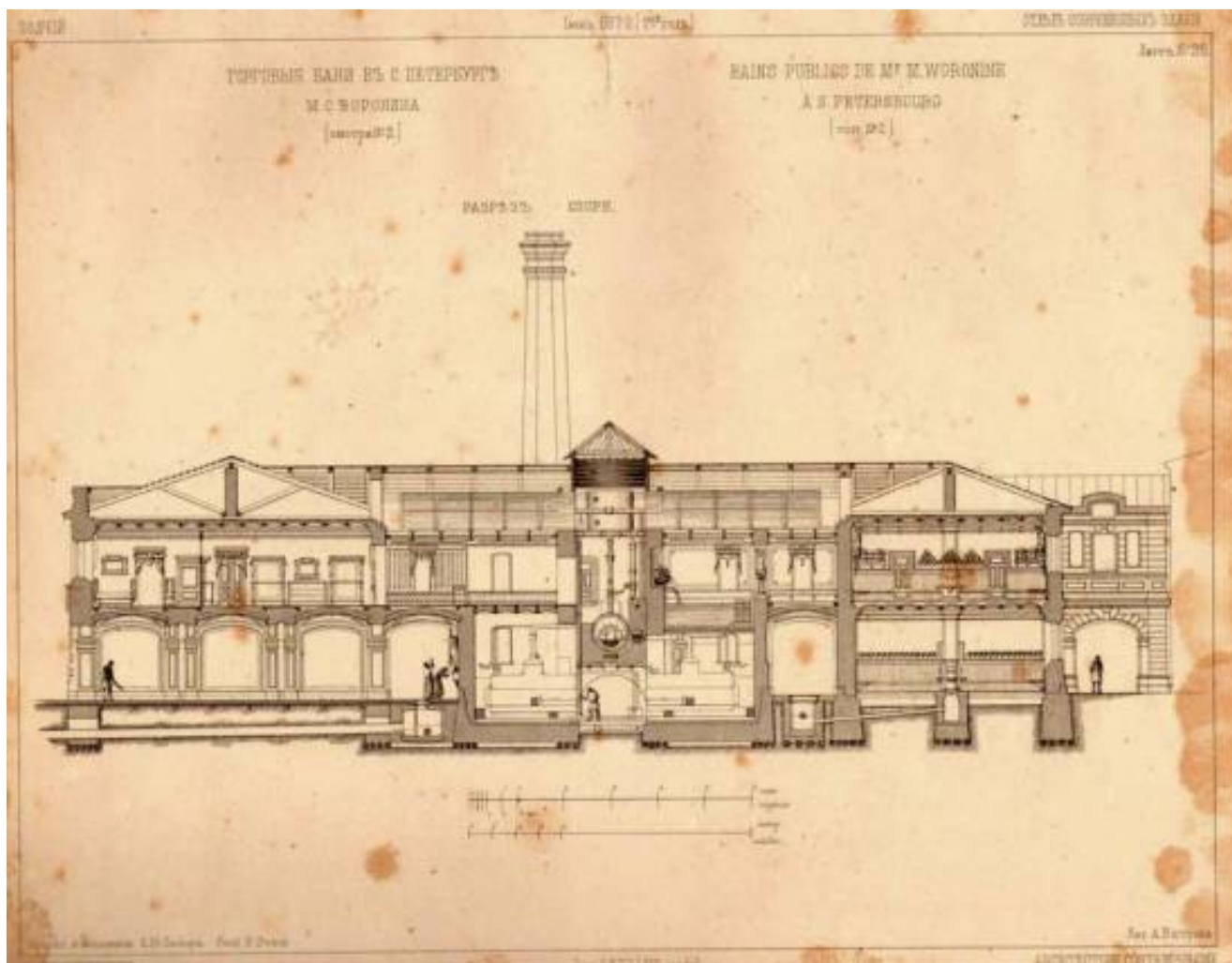
Илл. № 20. 1872 г. Торговые бани М.С. Воронина. Разрез. Зодчий, 1872, №2: Журн., изд. С.-Петербурб. о-вом архитекторов. – СПб.
