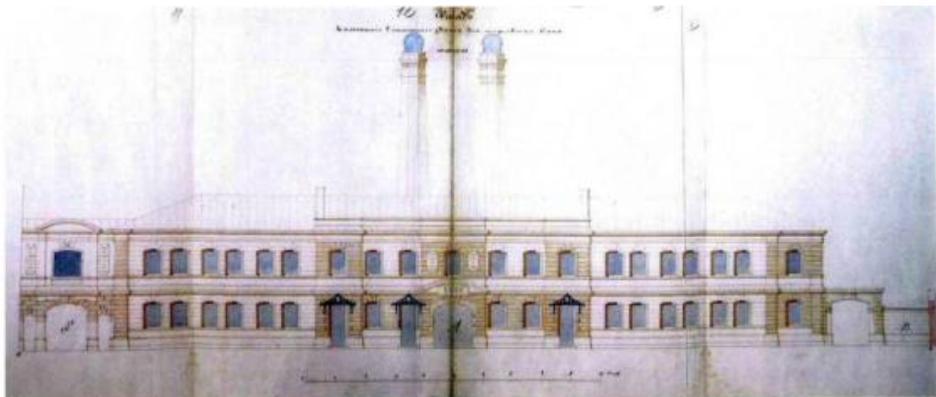
Илл. № 23. 1871 г. Главный (северный) фасад. Архитектор П.Ю. Сюзор. 1871. ЦГИА СПб. Ф. 515. Оп. 4. Д. 5607. Л. 11-14.
