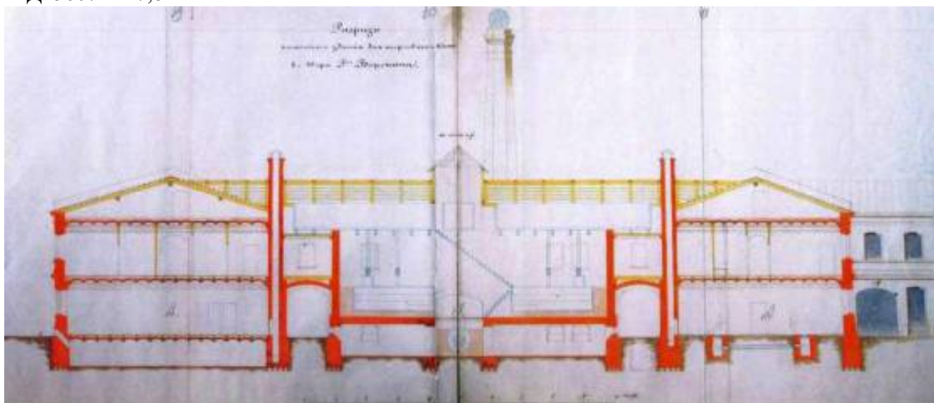
Илл. № 19. 1871 г. Разрез каменного здания для торговых бань во дворе Г-на Воронина. 1871. . ЦГИА СПб. Ф. 515. Оп. 4. Д. 5607. Л. 39-42.
