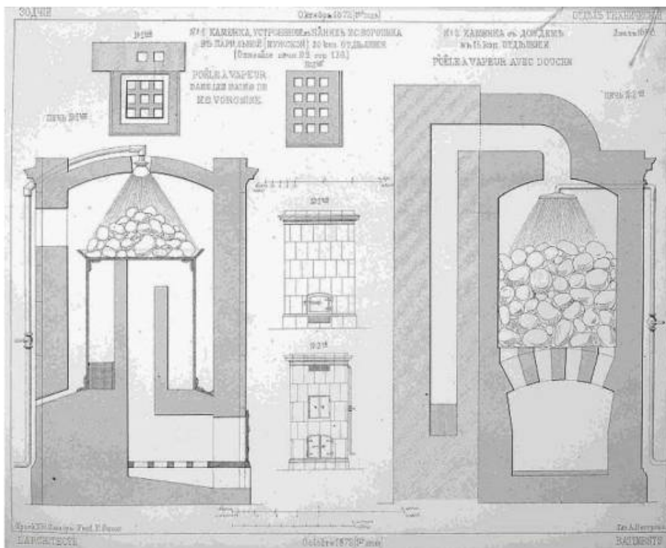
Илл. № 21. 1872 г. Торговые бани М.С. Воронина. Чертежи печей. Зодчий, 1872, №2: Журн., изд. С.-Петербур. о-вом архитекторов. – СПб.
