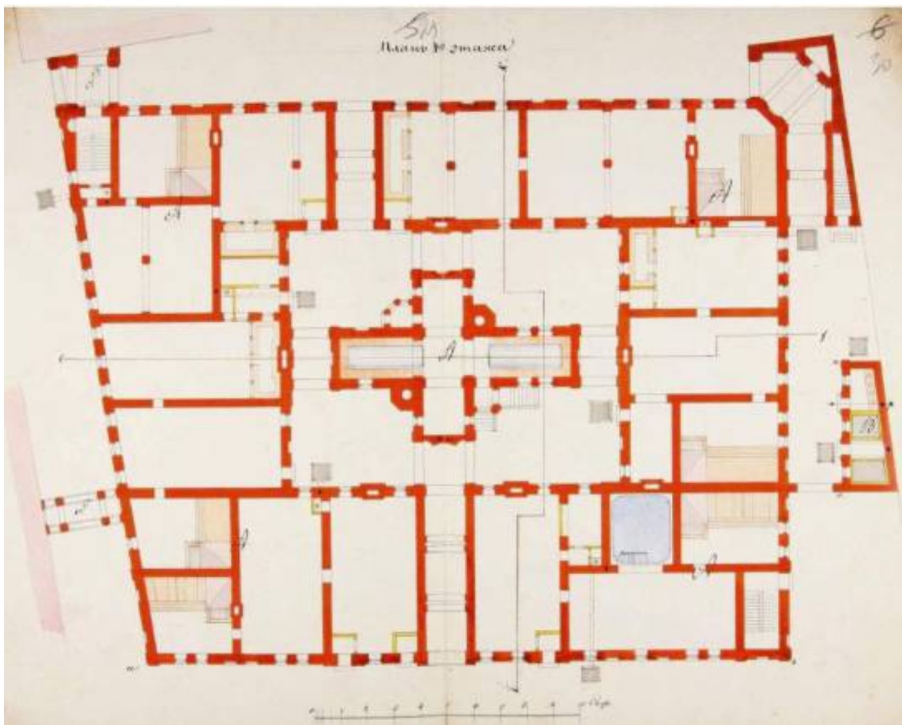
Илл. № 17. 1871 г. Торговые бани М.С. Воронина. План 1-го этажа. 1871. ЦГИА СПб. Ф. 515. Оп. 4. Д. 5607. Л. 5,6.
