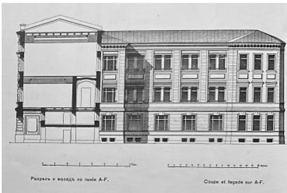
Илл.4. Здание для Высших женских курсов на месте снесенных построек. Арх. А.Красовский. 1884 г. Разрез. Барановский Г.В. Архитектурная энциклопедия второй половины XIX века. Т. II. СПб, 1908.
