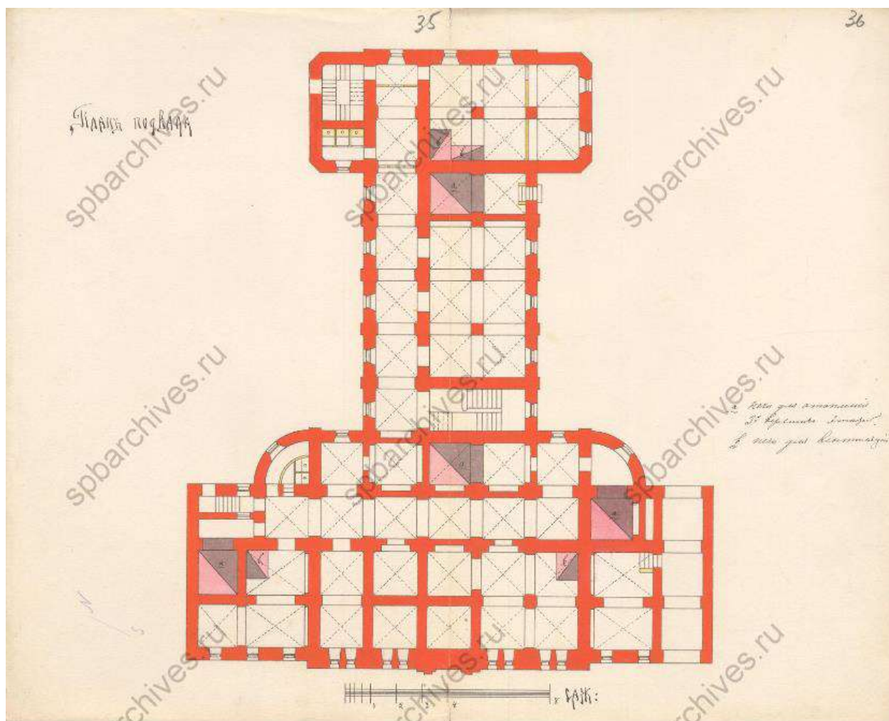
Илл.2. Здание для Высших женских курсов на месте снесенных построек. Арх. А.Красовский. 1884 г. План подвала (проект). ЦГИА СПб. Ф.513. Оп.102. Д.1751. Л.36.
