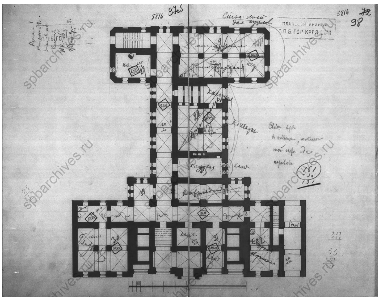
Илл.2а. Здание для Высших женских курсов на месте снесенных построек. Арх. А.Красовский. 1884 г. План подвала (фиксационный чертеж). ЦГИА СПб. Ф.515. Оп.4. Д.2839. Л.97 об-98.
