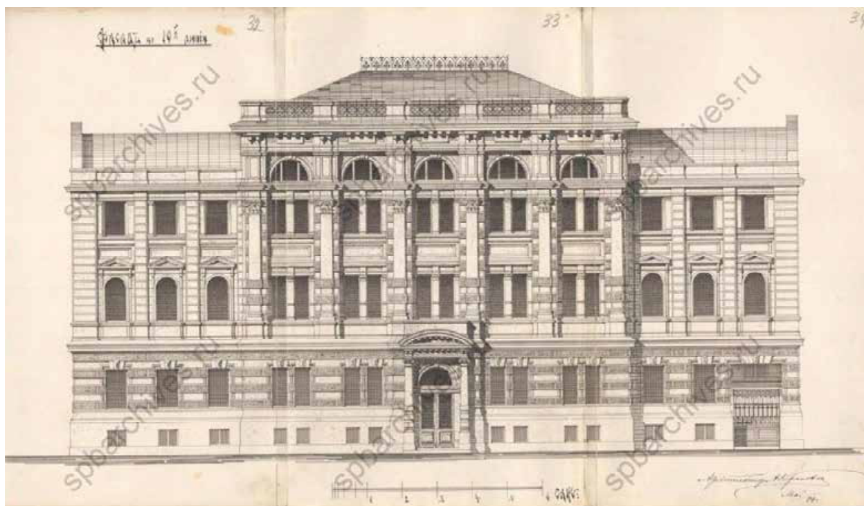
Илл.3. Здание для Высших женских курсов на месте снесенных построек. Арх. А.Красовский. 1884 г. Фасад. ЦГИА СПб. Ф.513. Оп.102. Д.1751. Л.32-34.
