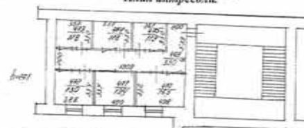
План антресоли.
