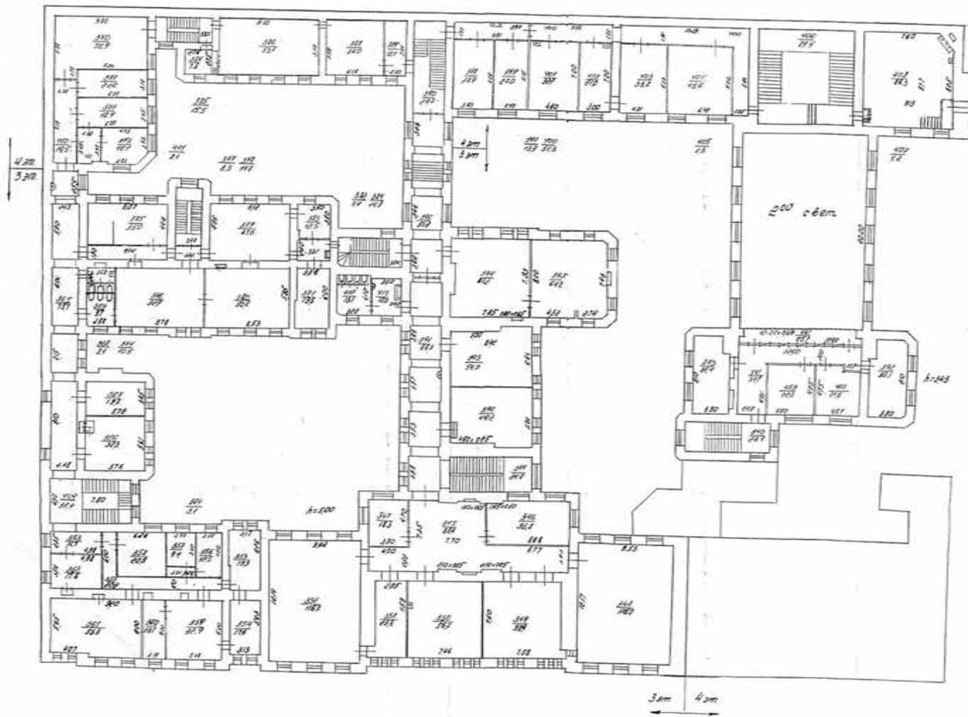
План 3 и 4 этажа
