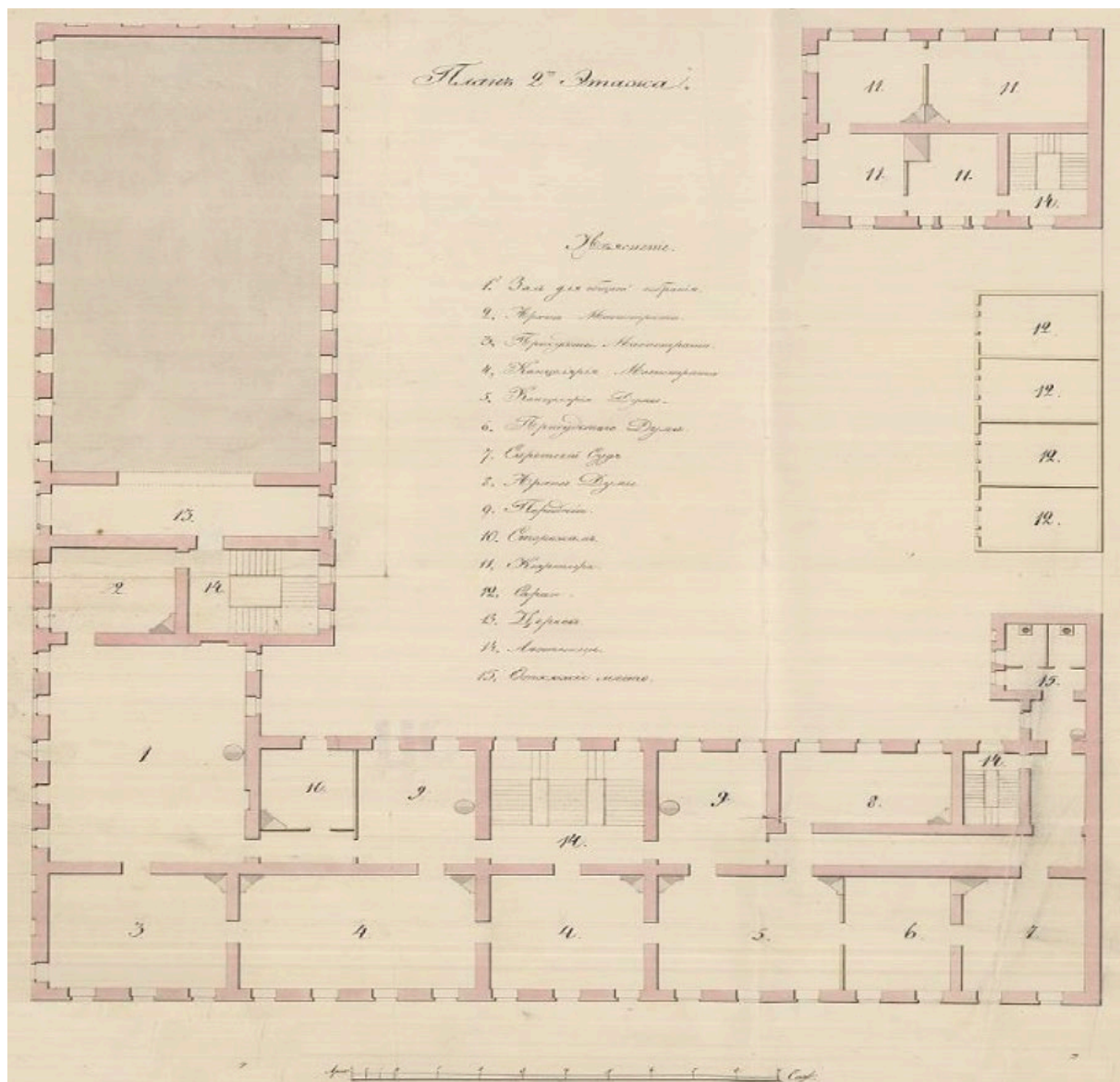
30. Проект здания «Градских присутственных мест» (литера С). План 2-го этажа (без клапана). Арх. Э. Х. Анерт. 1833 г. РГА ВМФ. Ф. 409. Оп. 2. Д. 1238.
