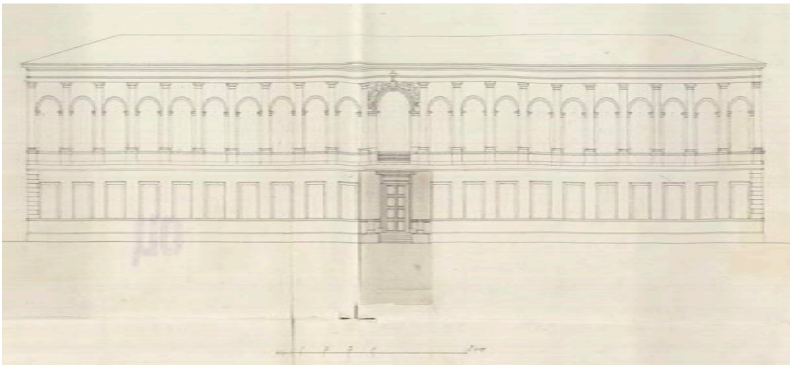
36. Проект здания «Градских присутственных мест». Фасад по Цитадельской улице (с клапаном). Арх. А.П. Брюллов. 1834 г. РГА ВМФ. Ф. 409. Оп. 2. Д. 1243.
