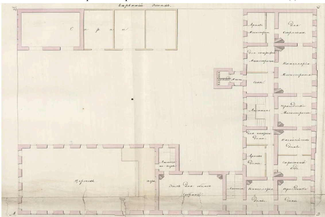
11. План 2-го этажа. Арх. Ф. И. Трапезников. 1833 г. РГА ВМФ. Ф. 409. Оп. 2. Д. 1219.
