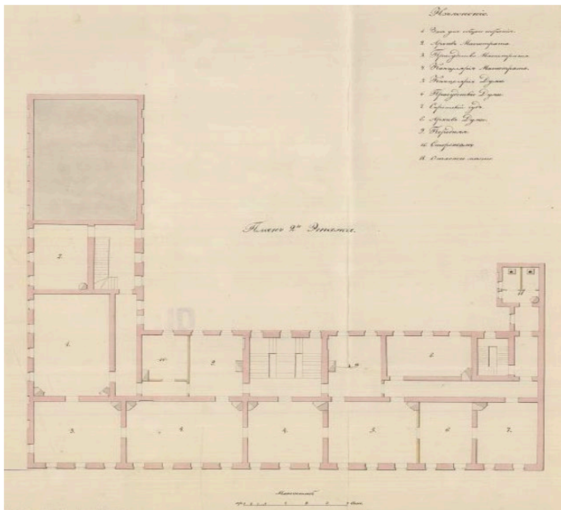
21. План 2-го этажа. Арх.Э. Х. Анерт. 1833 г. РГА ВМФ. Ф. 409. Оп. 2. Д. 1230.
