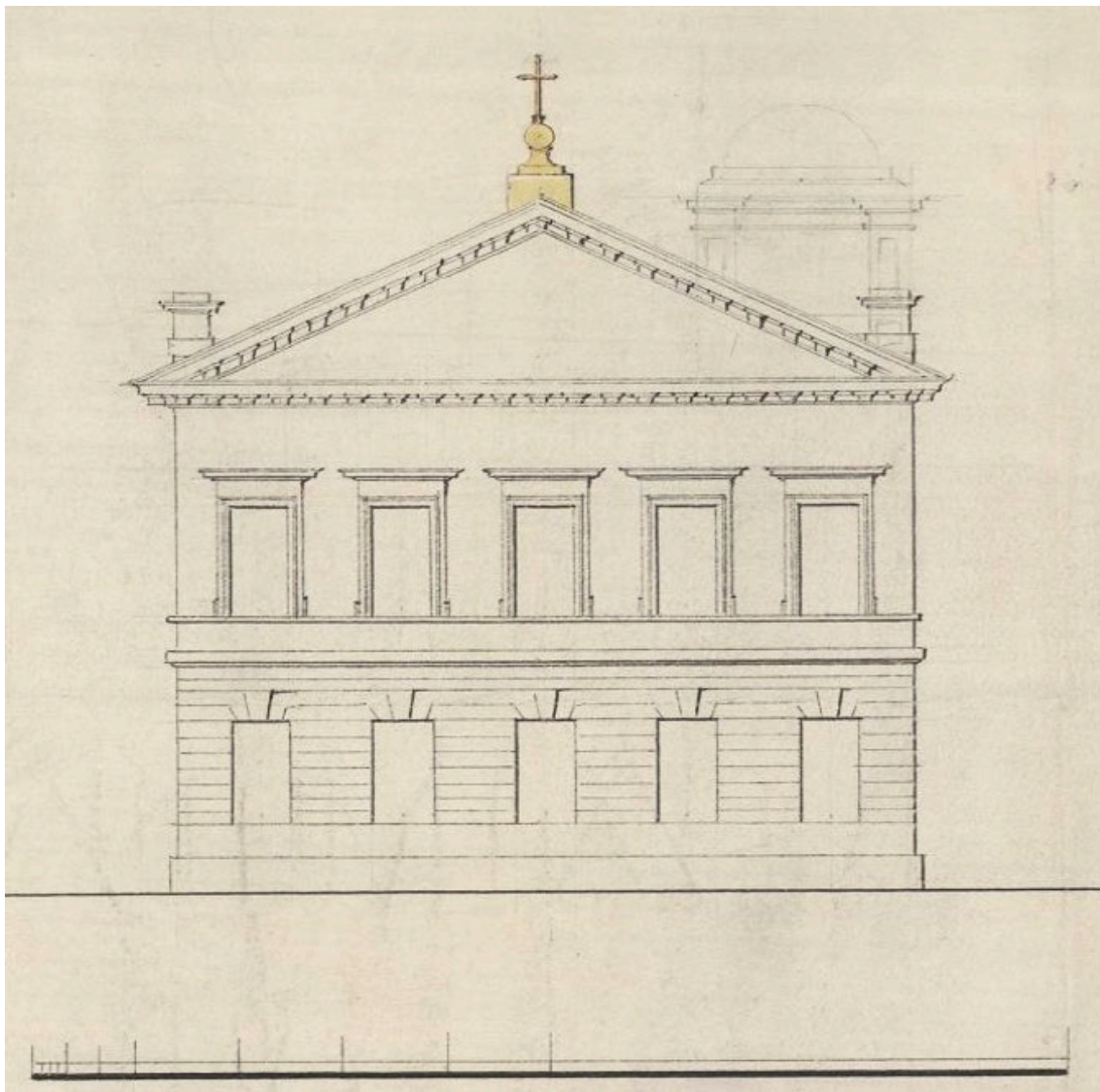
42. Фасад оконечности здания по Соборной улице с показанием изображения креста. Вероятно, 1834 г. РГА ВМФ. Ф. 409. Оп. 2. Д. 1253.
