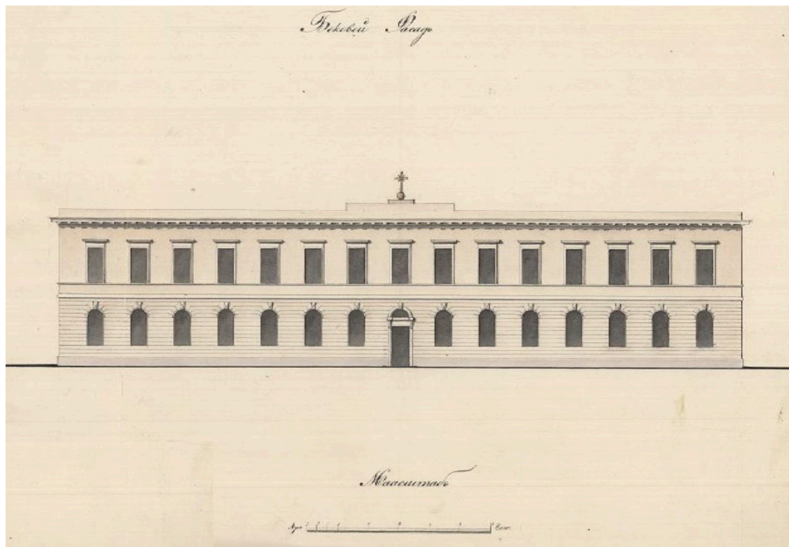
19. Боковой фасад. Арх.Э. Х. Анерт. 1833 г. РГА ВМФ. Ф. 409. Оп. 2. Д. 1227.
