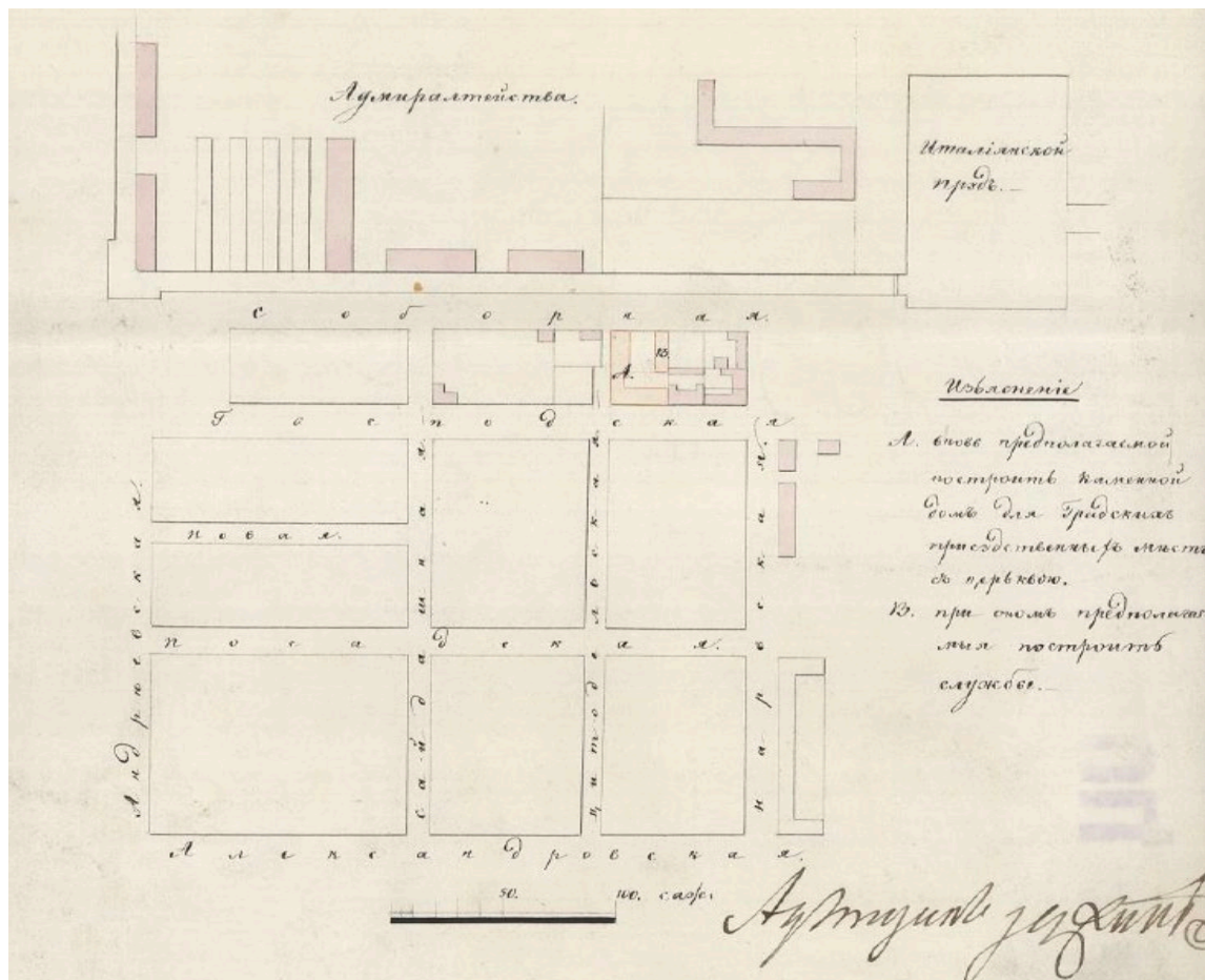
5. Генеральный план части города с показанием расположения предполагаемого к постройке здания «Губернских присутственных мест» с церковью и службами. Арх. Ф.И. Трапезников. 1833 г. РГА ВМФ. Ф. 409. Оп. 2. Д. 1217.
