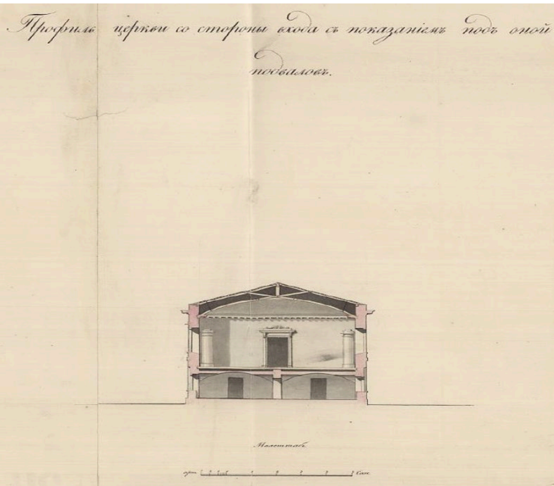
33. Проект здания «Градских присутственных мест». Профиль церкви со стороны входа с показанием подвалов. Арх. Э. Х. Анерт. 1833 г. РГА ВМФ. Ф. 409. Оп. 2. Д. 1240.
