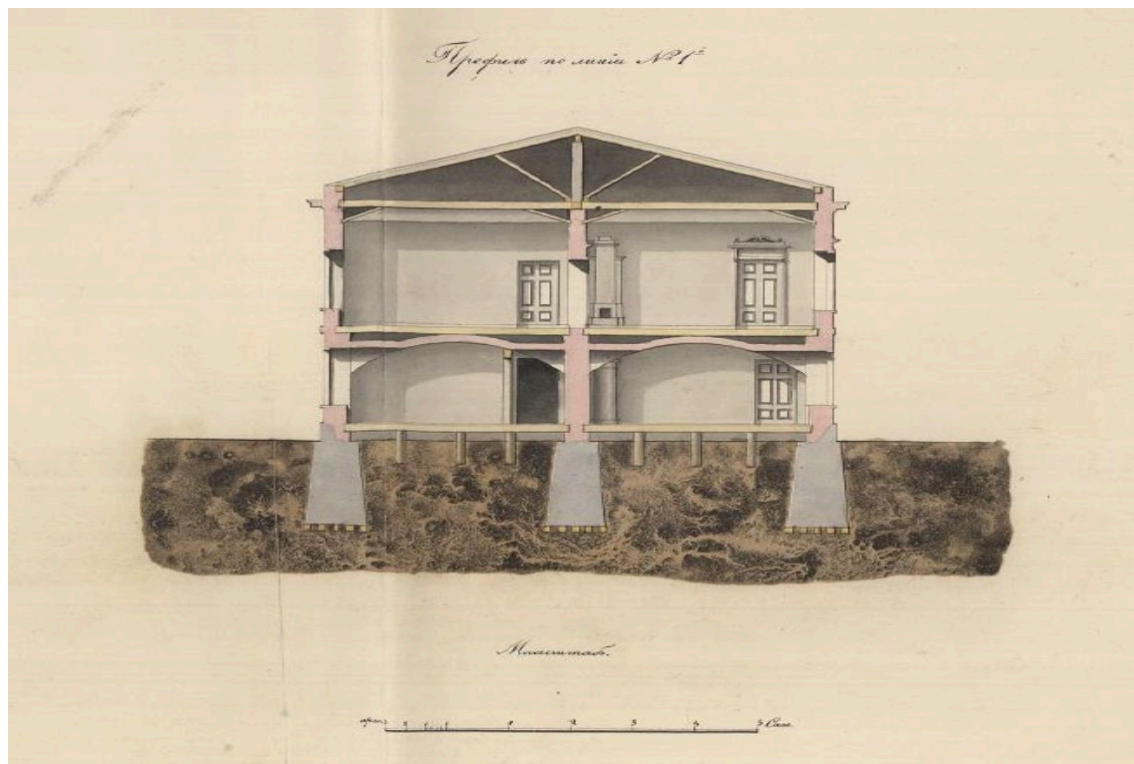
24. Проект здания «Градских присутственных мест» (литера В) с церковью и службами. Профиль по линии № 1. Арх. Э. Х. Анерт. 1833 г. РГА ВМФ. Ф. 409. Оп. 2. Д. 1233.
