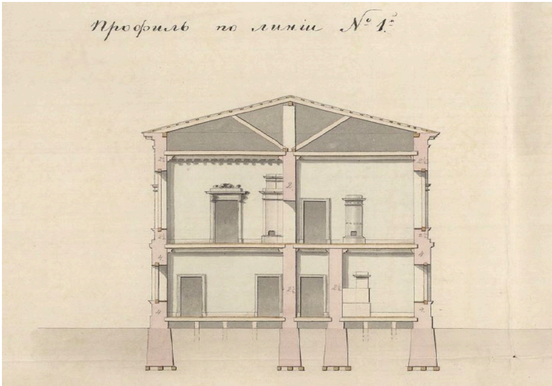
15. Профиль по линии № 1. Арх. Ф. И. Трапезников. 1833 г. РГА ВМФ. Ф. 409. Оп. 2. Д. 1223.
