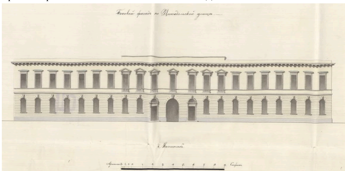
39. Проект здания «Градских присутственных мест». Фасад по Цитадельской улице. Арх. А.П. Брюллов. 1834 г. РГА ВМФ. Ф. 409. Оп. 2. Д. 1246.
