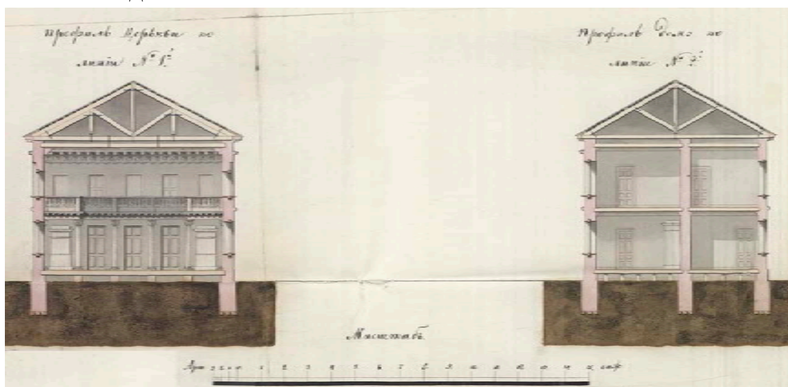
9. Профиль церкви по линии № 1. Профиль дома по линии № 2. Арх. Ф. И. Трапезников. 1833 г. РГА ВМФ. Ф. 409. Оп. 2. Д. 1218.
