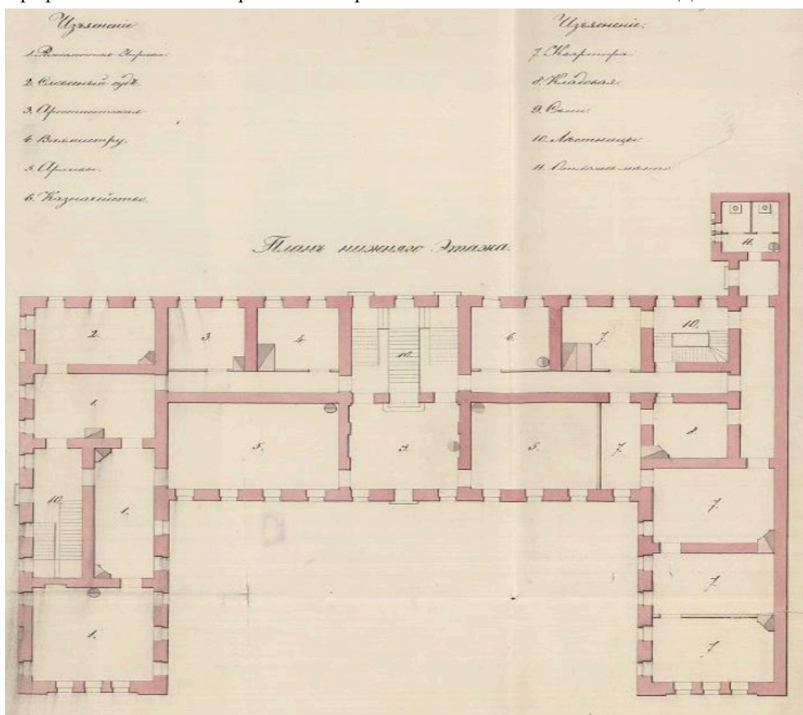
25. Проект здания «Градских присутственных мест» (литера В) с церковью и службами. План нижнего этажа. Арх. Э. Х. Анерт. 1833 г. РГА ВМФ. Ф. 409. Оп. 2. Д. 1234.
