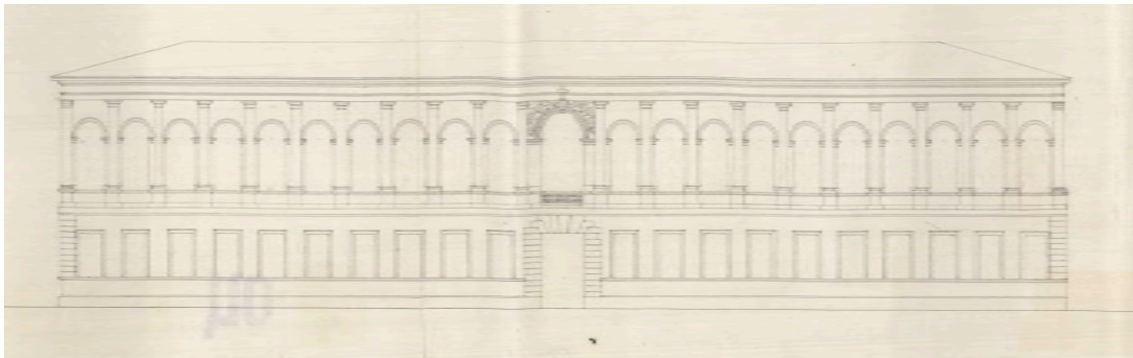
35. Проект здания «Градских присутственных мест». Фасад по Цитадельской улице (без клапана). Арх. А.П. Брюллов. 1834 г. РГА ВМФ. Ф. 409. Оп. 2. Д. 1243.
