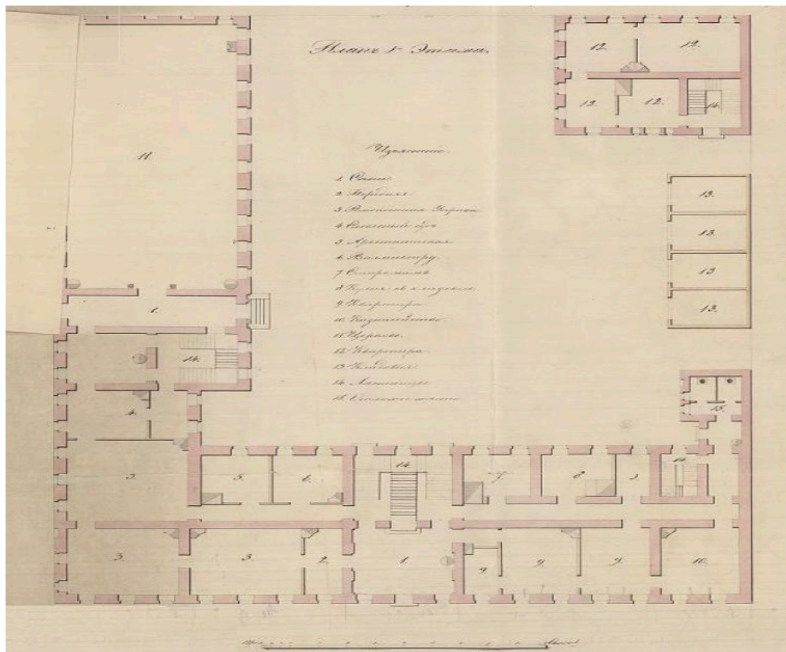
28. Проект здания «Градских присутственных мест» (литера С). План 1-го этажа (без клапана). Арх. Э. Х. Анерт. 1833 г. РГА ВМФ. Ф. 409. Оп. 2. Д. 1237.
