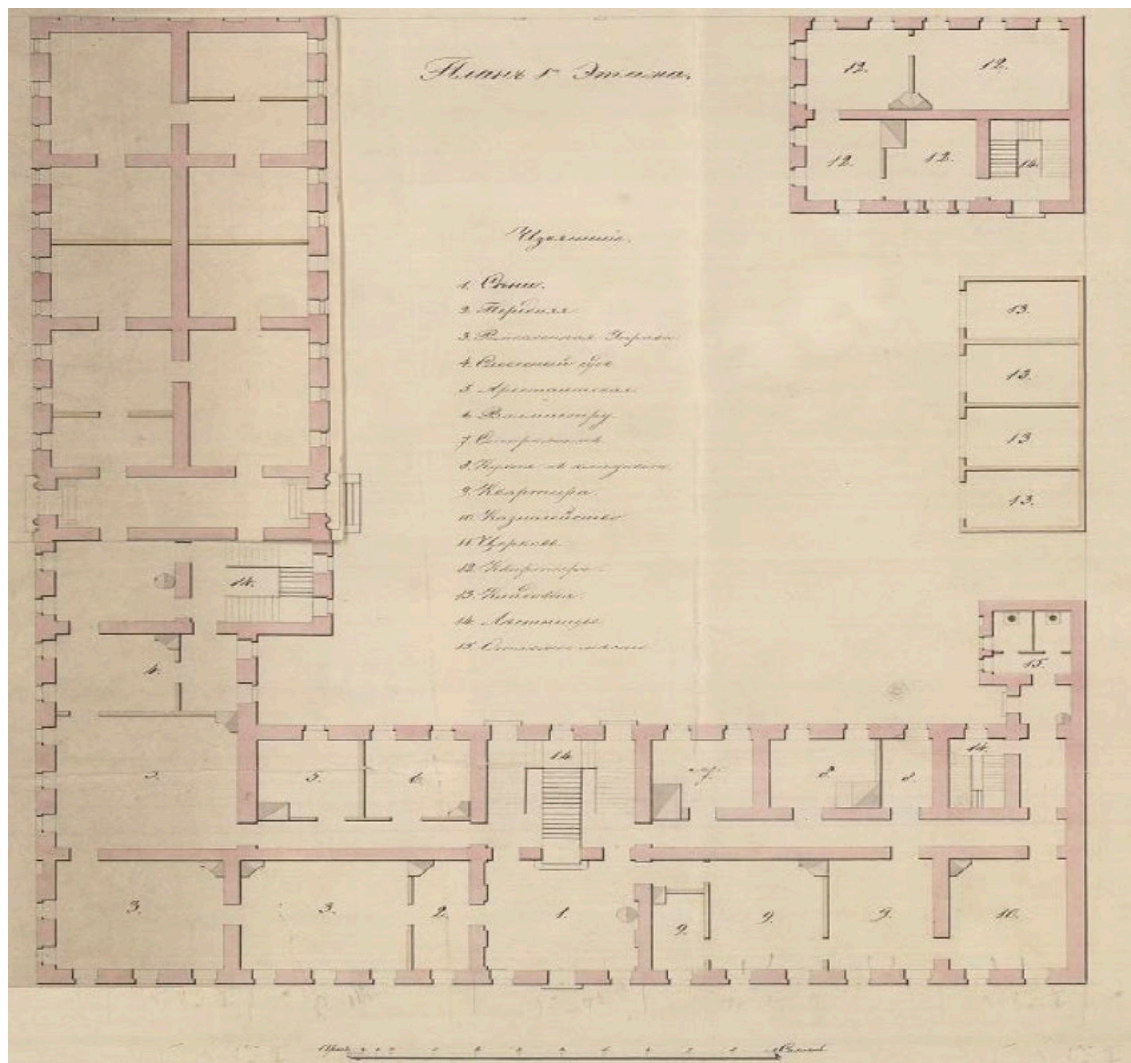
29. Проект здания «Градских присутственных мест» (литера С). План 1-го этажа (с клапаном). Арх. Э. Х. Анерт. 1833 г. РГА ВМФ. Ф. 409. Оп. 2. Д. 1237.
