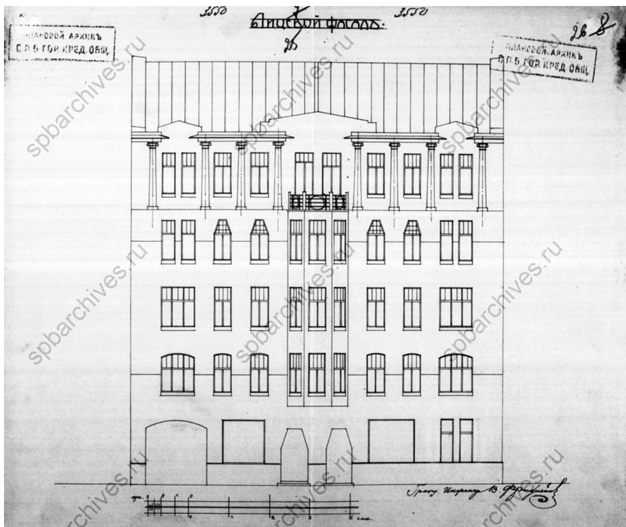
Илл. 17. Лицевой фасад. 1911 г. ЦГИА СПб. Ф. 515. Оп. 4. Д. 4535. Л. 24.
