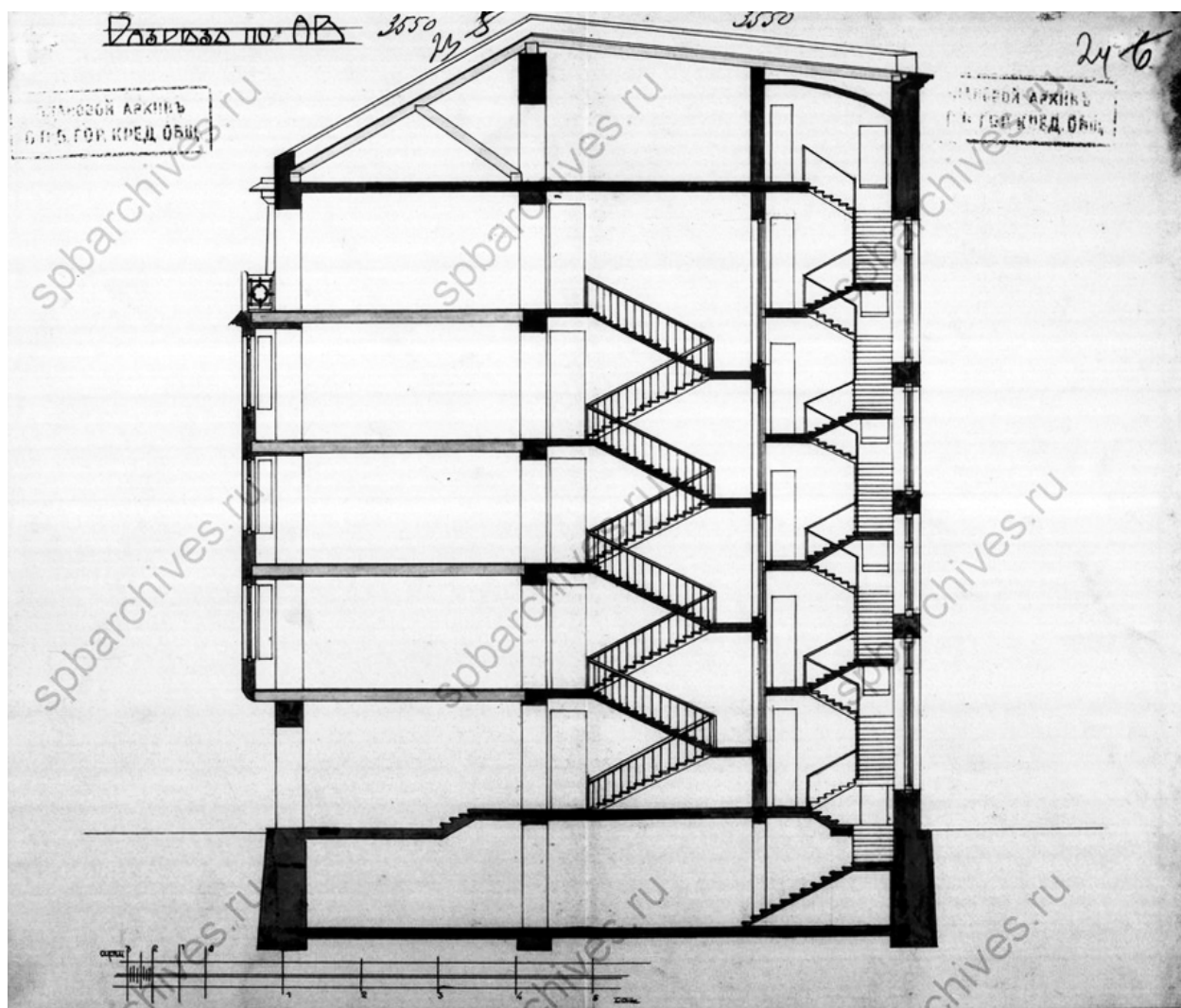
Илл. 16. Разрез по АВ. 1911 г. ЦГИА СПб. Ф. 515. Оп. 4. Д. 4535. Л. 23.
