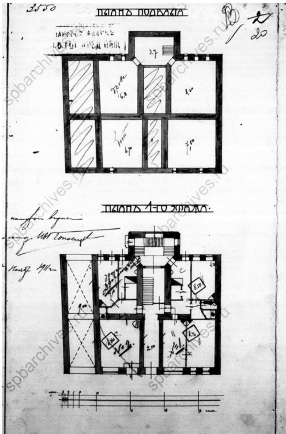
Илл. 13. Планы подвала и 1-го этажа. 1911 г. ЦГИА СПб. Ф. 515. Оп. 4. Д. 4535. Л. 20.
