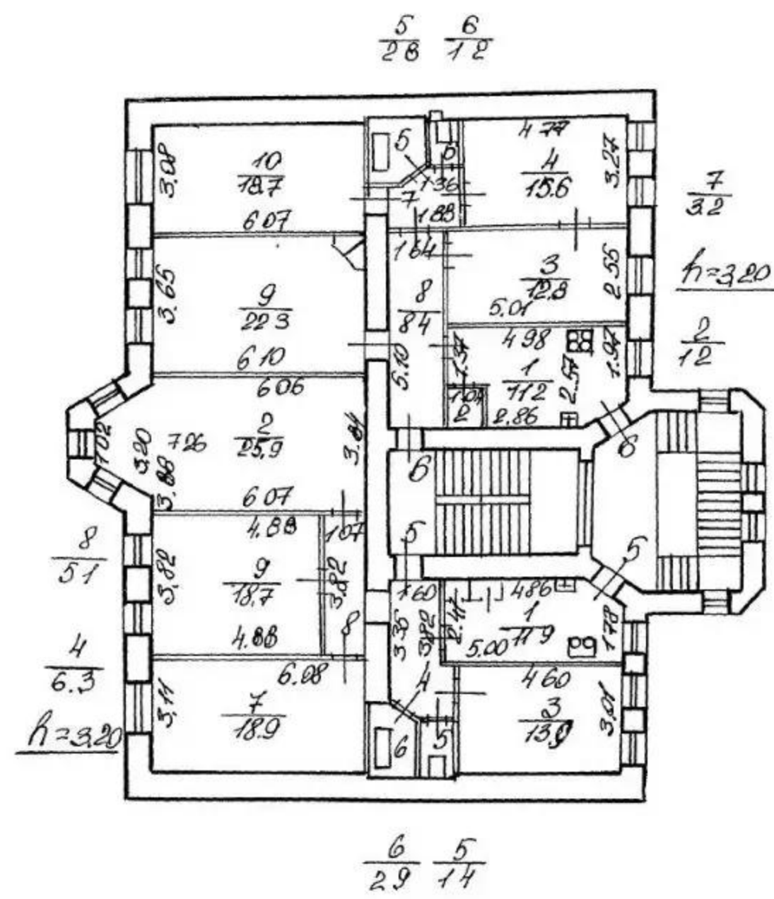
План 3 этажа
