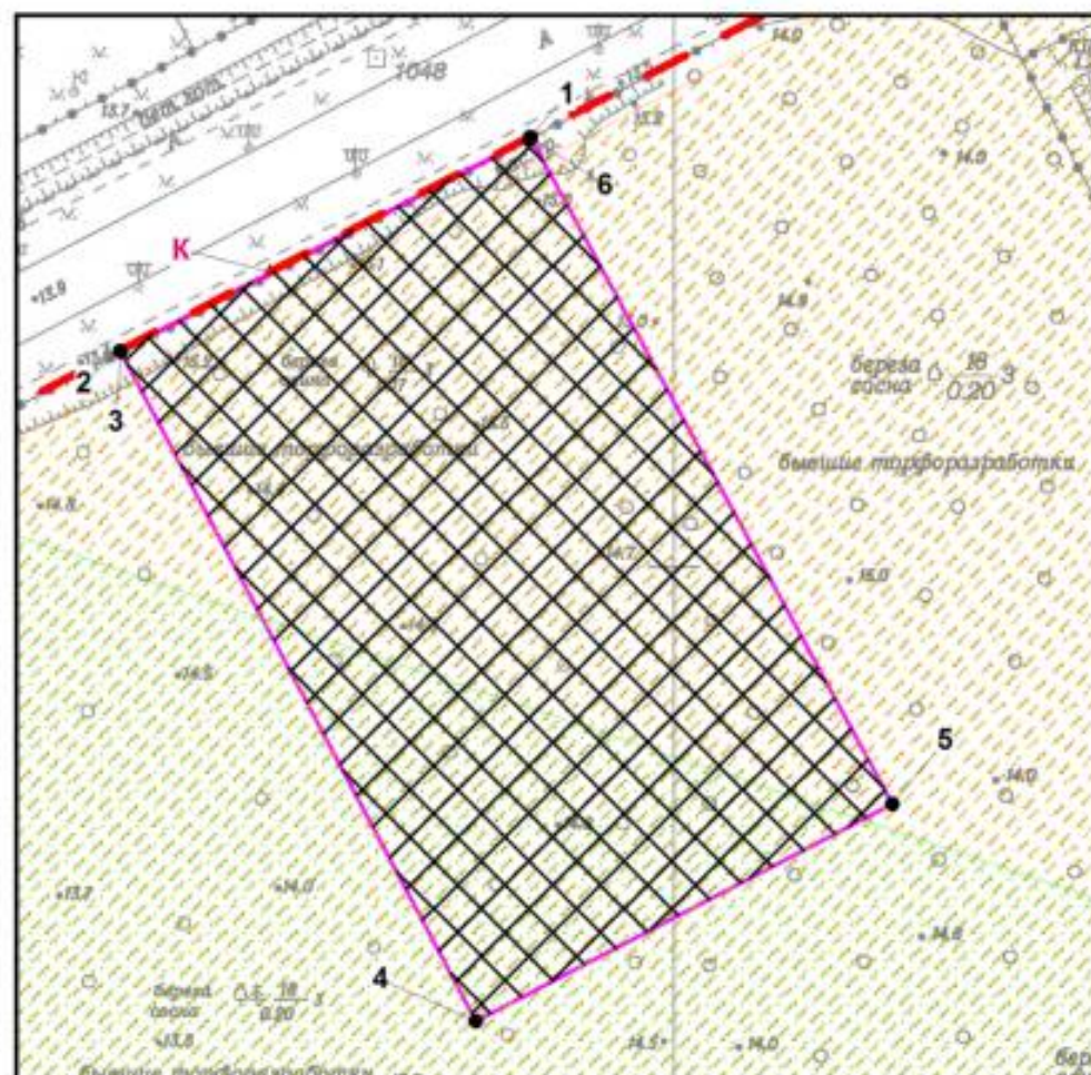
Схема расположения земельного участка в окружении смежно расположенных земельных участков (ситуационный план), М1:10000
