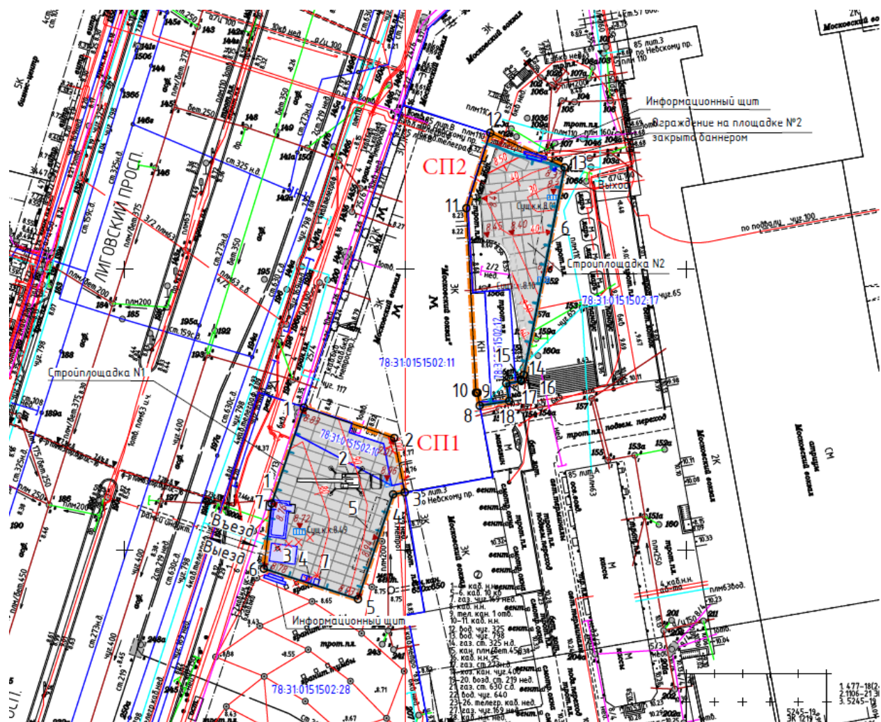
Расположение строительной площадки 1 (СП1) и строительной площадки 2 (СП2)
