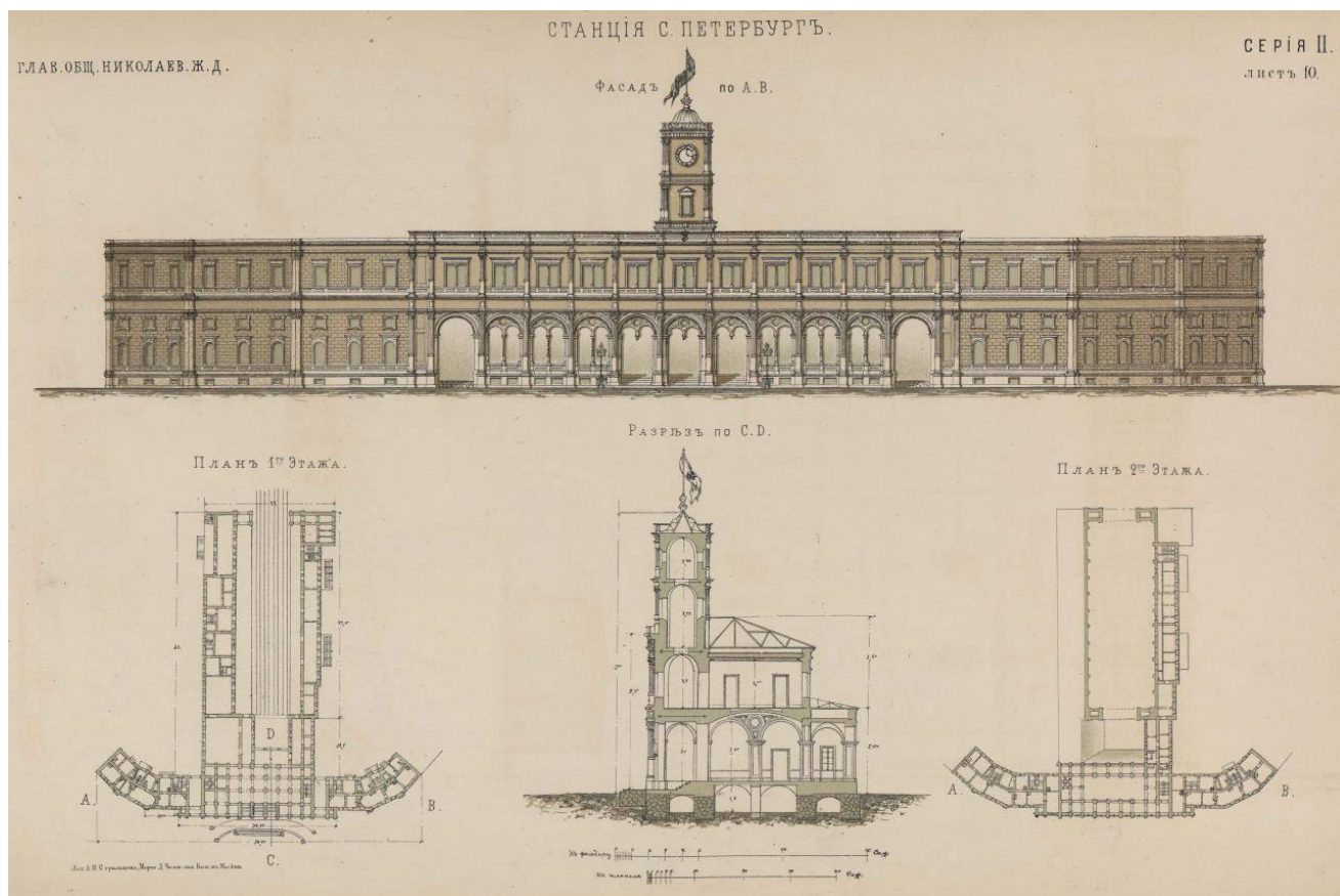
1. Здание Московского (бывш. Николаевского) вокзала. 1868, 1878 гг. //
