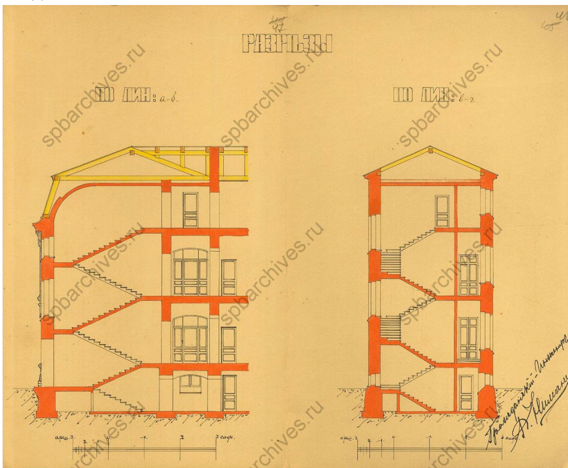
26. Чертежи дома на участке, принадлежавшем Колкачеву, Герасимовой, А.И. Дворжецкой, А.Я. Фрею, А.Э. Бари по 5-й линии В.О., 60. ЦГИА СПб. Фонд 513. Опись 102. Дело 1591. Разрезы.
