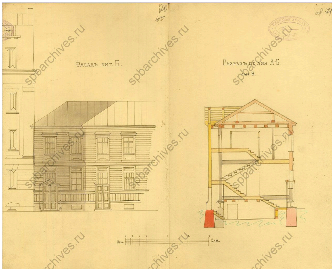
40. Чертежи дома на участке, принадлежавшем Колкачеву, Герасимовой, А.И. Дворжецкой, А.Я.FREY, A.Э. Бари по 5-й линии В.О., 60. ЦГИА СПб. Фонд 513. Описание 102. Дело 1591. Фасад и разрез.
