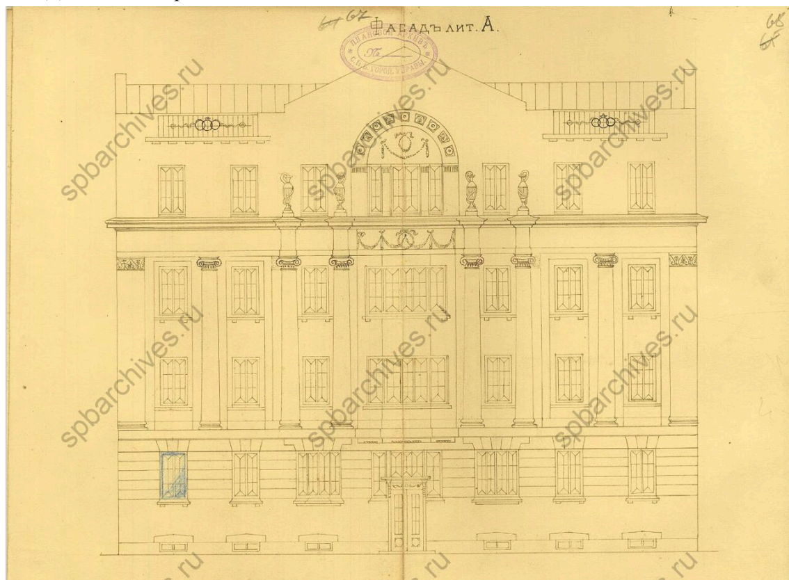
38. Чертежи дома на участке, принадлежавшем Колкачеву, Герасимовой, А.И. Дворжецкой, А.Я. Фрею, А.Э. Бари по 5-й линии В.О., 60. ЦГИА СПб. Фонд 513. Опись 102. Дело 1591. Фасад.
