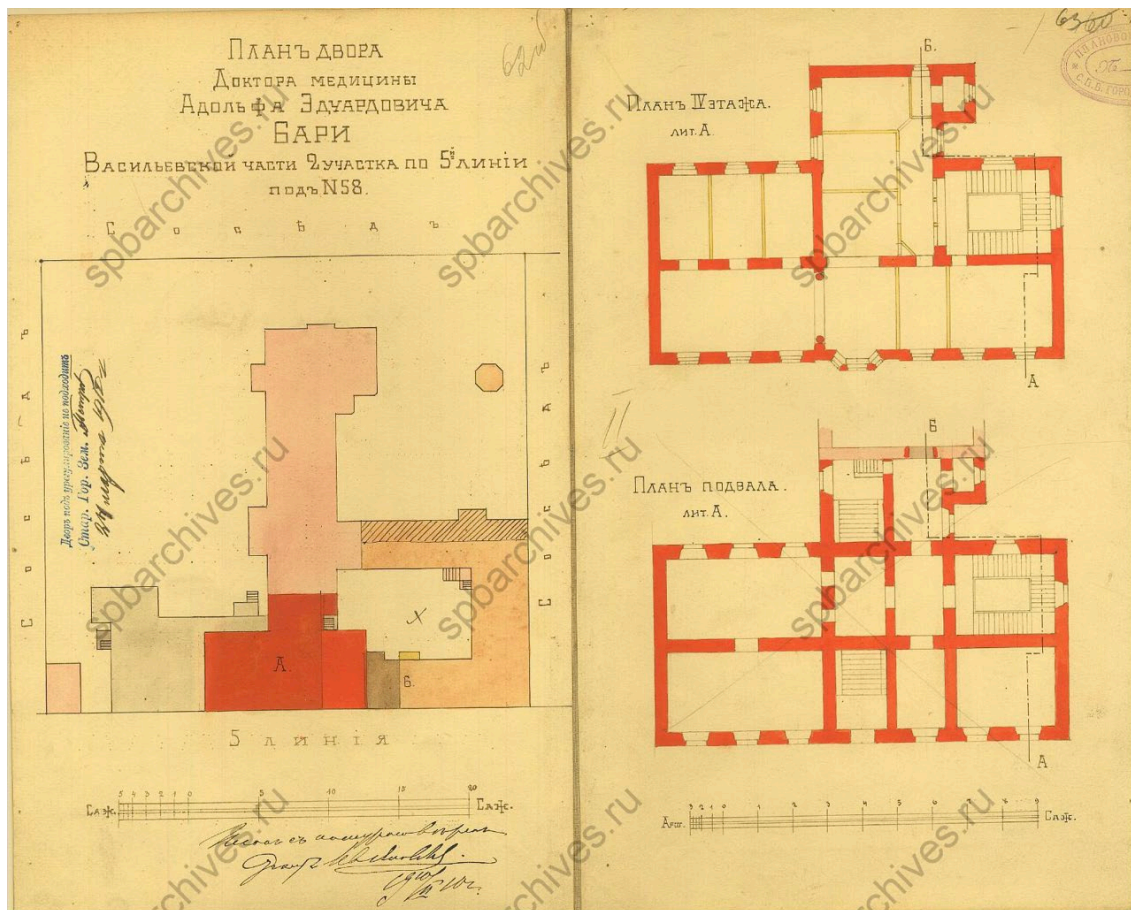
35. Чертежи дома на участке, принадлежавшем Колкачеву, Герасимовой, А.И. Дворжецкой, А.Я. Фрею, А.Э. Бари по 5-й линии В.О., 60. ЦГИА СПб. Фонд 513. Опись 102. Дело 1591. План двора Бари, 1910 г. и планы подвала и 4 этажей.
