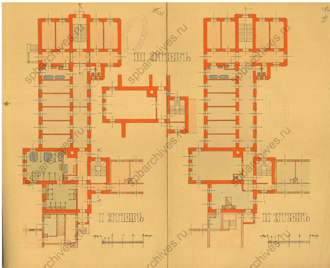
23. Чертежи дома на участке, принадлежавшем Колкачеву, Герасимовой, А.И. Дворжецкой, А.Я.FREY, A.E. Бари по 5-й линии В.О., 60. ЦГИА СПб. Фонд 513. Описание 102. Дело 1591. Планы 1,2 и 3 этажей.
