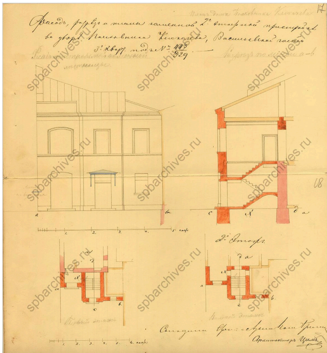
14. Чертежи дома на участке, принадлежавшем Колчаеву, Герасимовой, А.И. Дворжецкой, А.Я. Фрею, А.Э. Бари по 5-й линии В.О., 60. ЦГИА СПб. Фонд 513. Опись 102. Дело 1591. Фасад и разрез.
