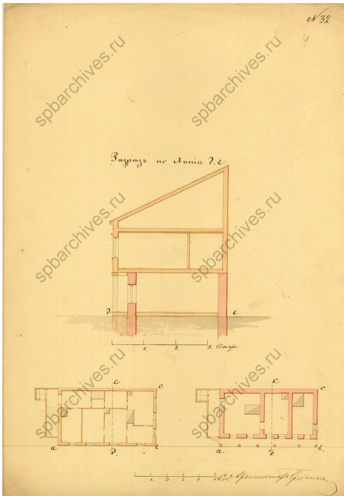
6. Чертежи дома на участке, принадлежавшем Колкачеву, Герасимовой, А.И. Дворжецкой, А.Я. Фрею, А.Э. Бари по 5-й линии В.О., 60. ЦГИА СПб. Фонд 513. Опись 102. Дело 1591. Разрезы.
