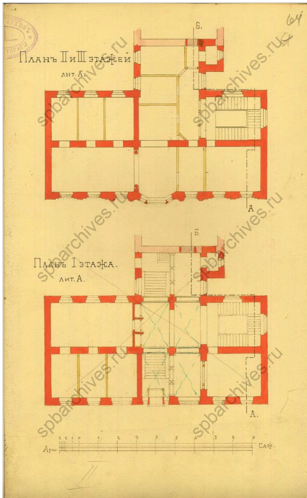
36. Чертежи дома на участке, принадлежавшем Колкачеву, Герасимовой, А.И. Дворжецкой, А.Я. Фрею, А.Э. Бари по 5-й линии В.О., 60. ЦГИА СПб. Фонд 513. Опись 102. Дело 1591. Планы 1, 2, 3 этажей.
