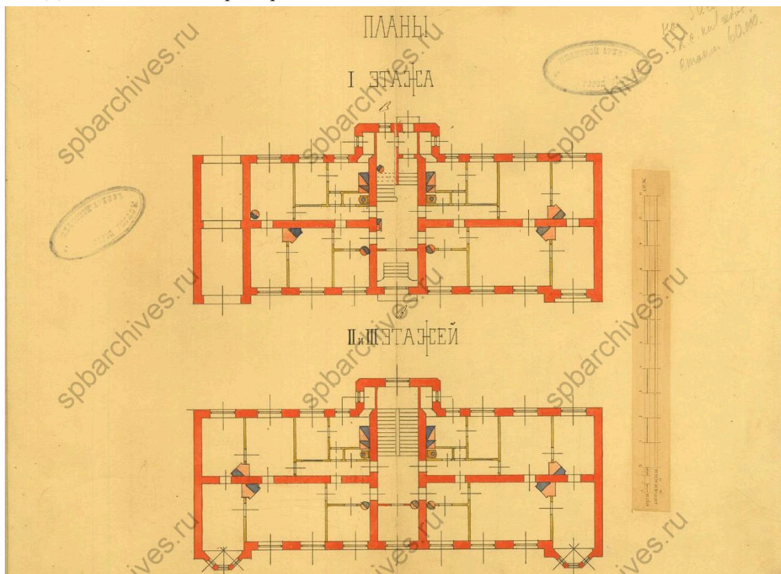
30. Чертежи дома на участке, принадлежавшем Колкачеву, Герасимовой, А.И. Дворжецкой, А.Я. Фрею, А.Э. Бари по 5-й линии В.О., 60. ЦГИА СПб. Фонд 513. Описание 102. Дело 1591. Планы 1, 2, 3 этажей.
