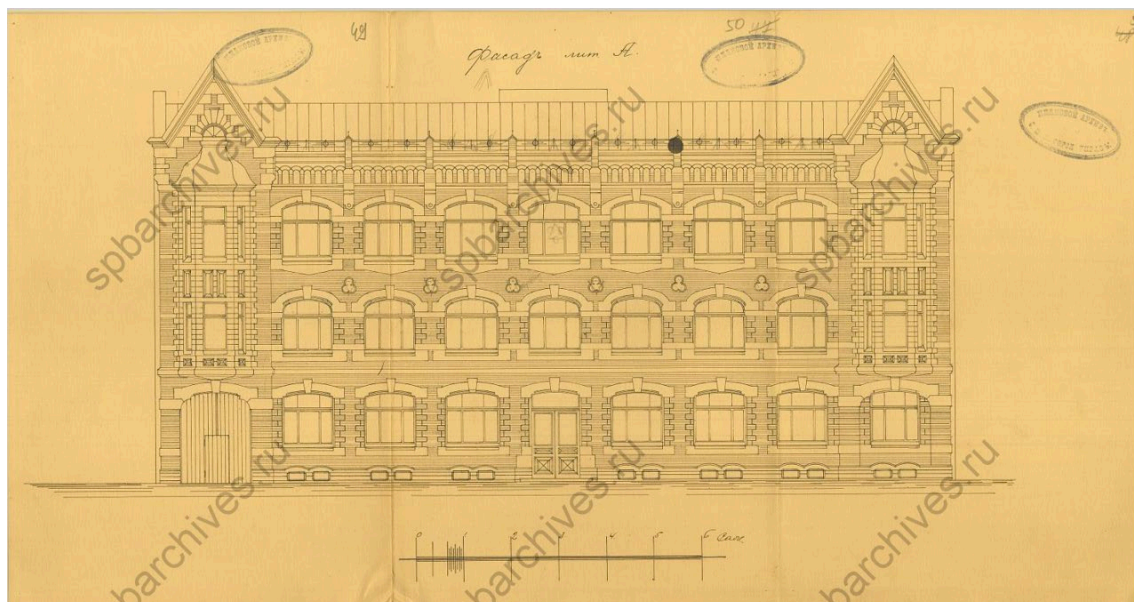
27. Чертежи дома на участке, принадлежавшем Колкачеву, Герасимовой, А.И. Дворжецкой, А.Я. Фрею, А.Э. Бари по 5-й линии В.О., 60. ЦГИА СПб. Фонд 513. Опись 102. Дело 1591. Фасад.
