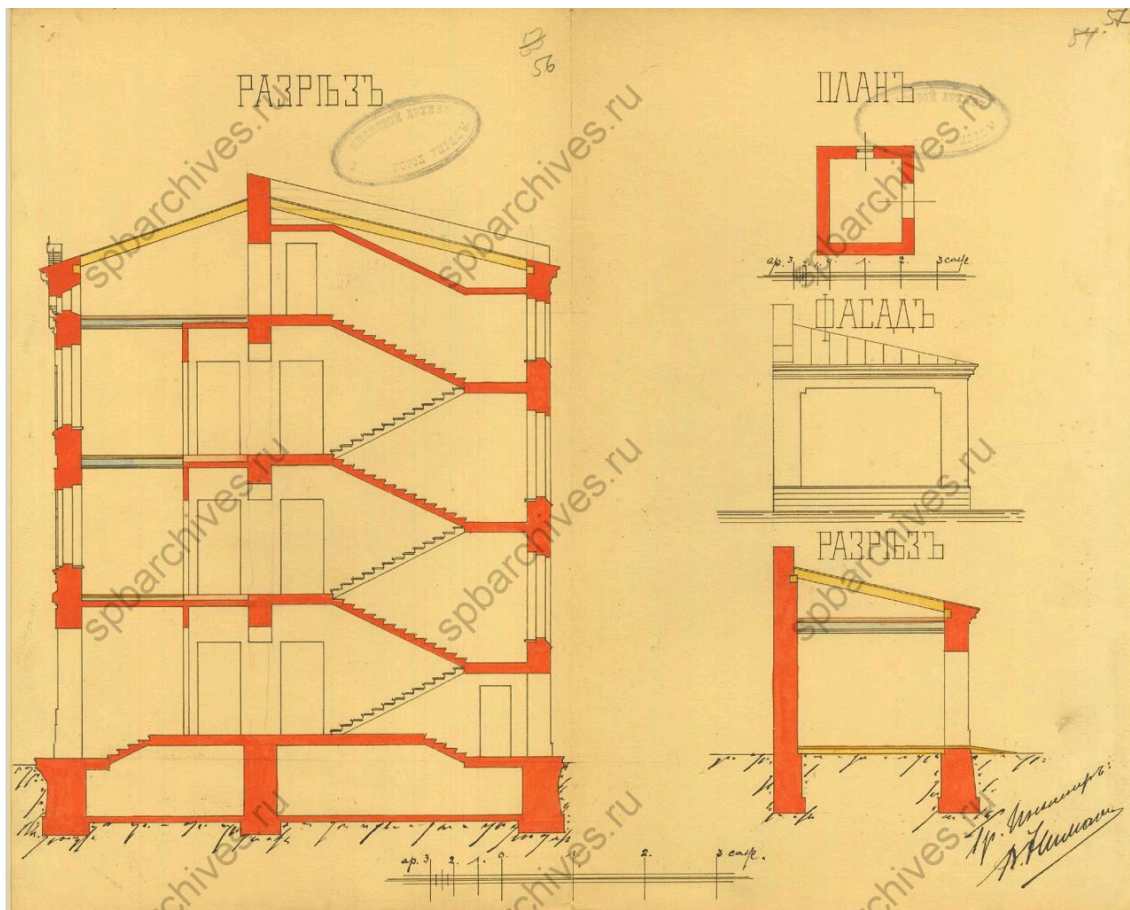
31. Чертежи дома на участке, принадлежавшем Колкачеву, Герасимовой, А.И. Дворжецкой, А.Я. Фрею, А.Э. Бари по 5-й линии В.О., 60. ЦГИА СПб. Фонд 513. Опись 102. Дело 1591. Разрезы.
