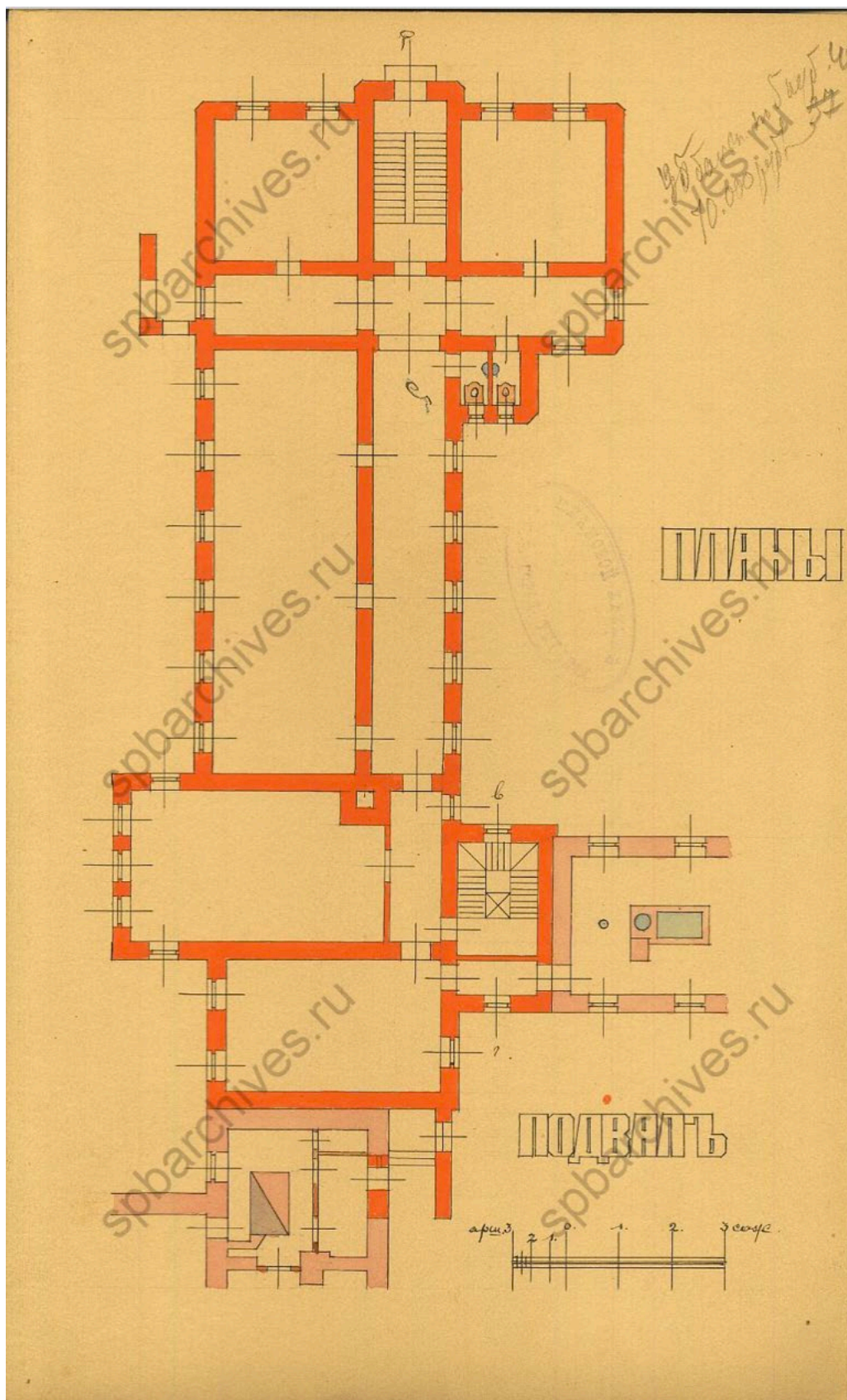
22. Чертежи дома на участке, принадлежавшем Колкачеву, Герасимовой, А.И. Дворжецкой, А.Я. Фрею, А.Э. Бари по 5-й линии В.О., 60. ЦГИА СПб. Фонд 513. Опись 102. Дело 1591. План подвала.
