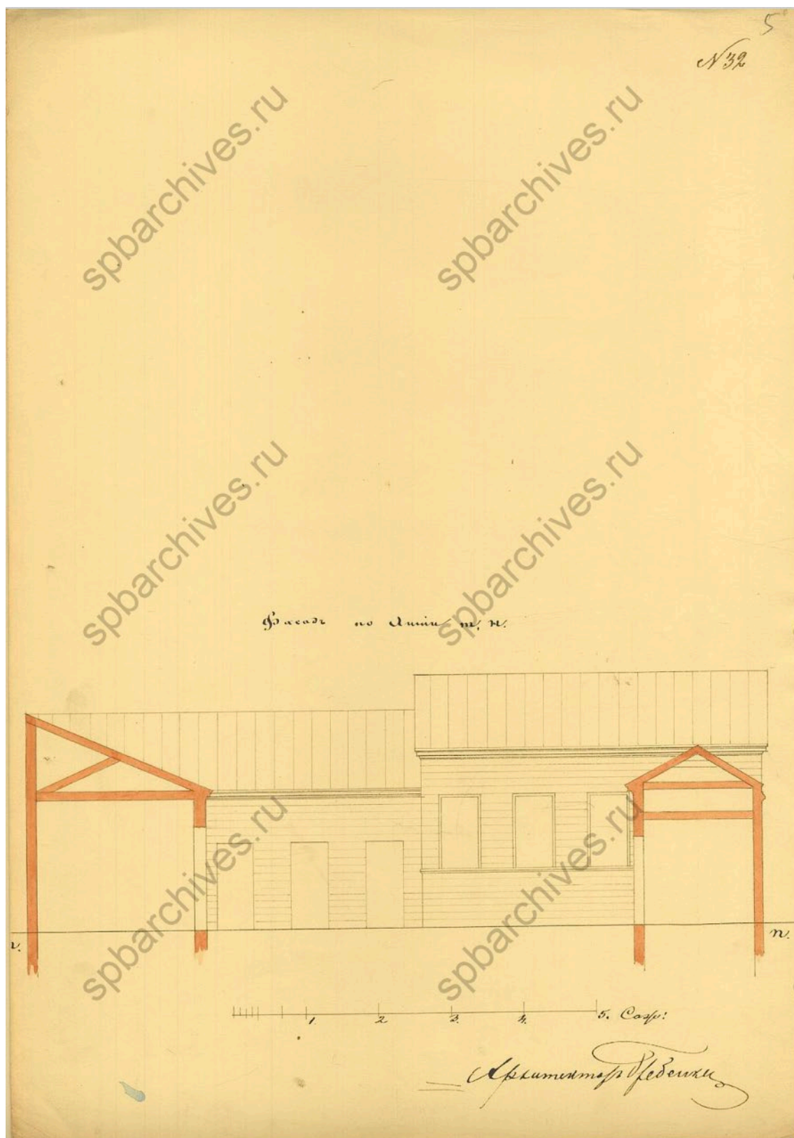
7. Чертежи дома на участке, принадлежавшем Колкачеву, Герасимовой, А.И. Дворжецкой, А.Я.FREY, А.Э. Бари по 5-й линии В.О., 60. ЦГИА СПб. Фонд 513. Опись 102. Дело 1591.
