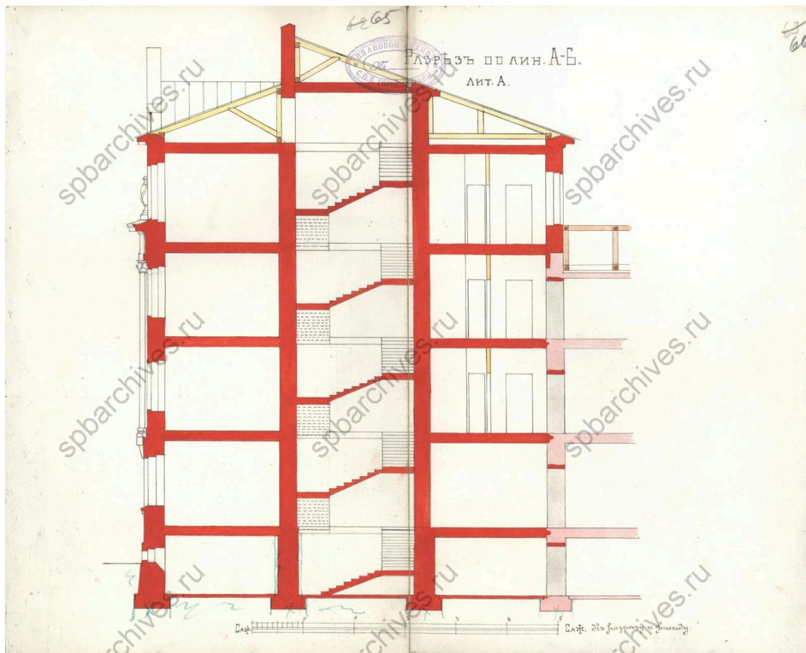
37. Чертежи дома на участке, принадлежавшем Колкачеву, Герасимовой, А.И. Дворжецкой, А.Я. Фрею, А.Э. Бари по 5-й линии В.О., 60. ЦГИА СПб. Фонд 513. Описание 102. Дело 1591. Разрез.
